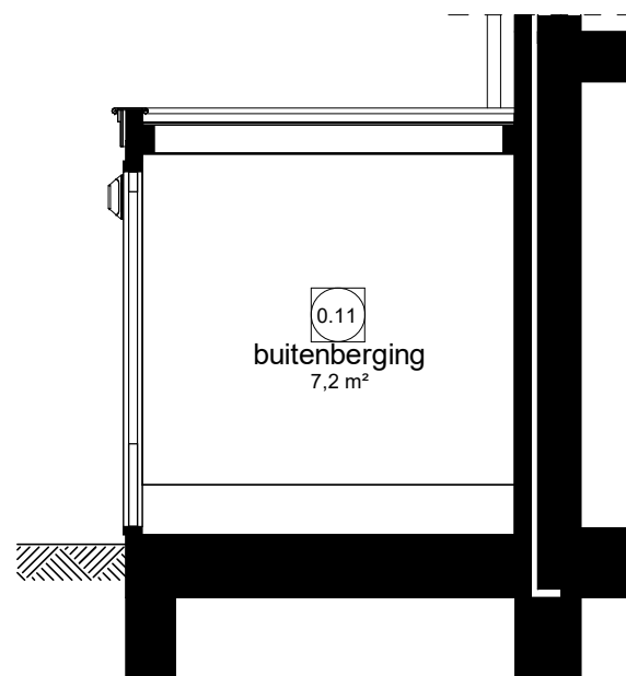
Doorsnede E1.1
