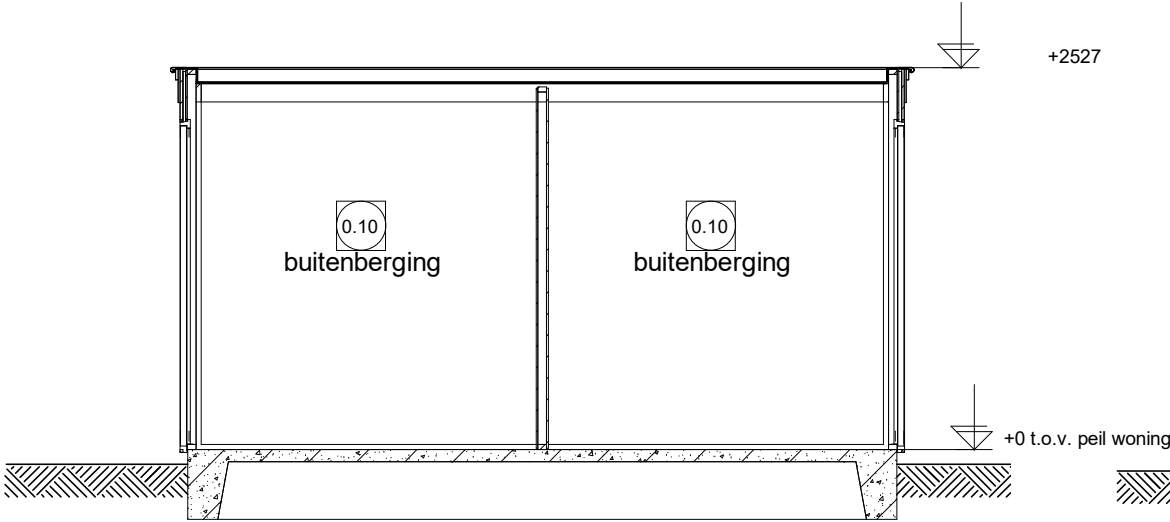
Doorsnede R
