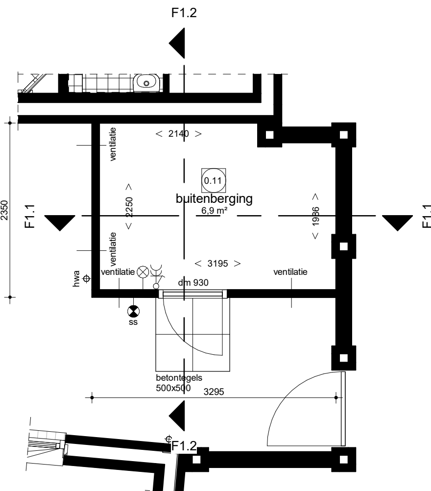
Begane grond
