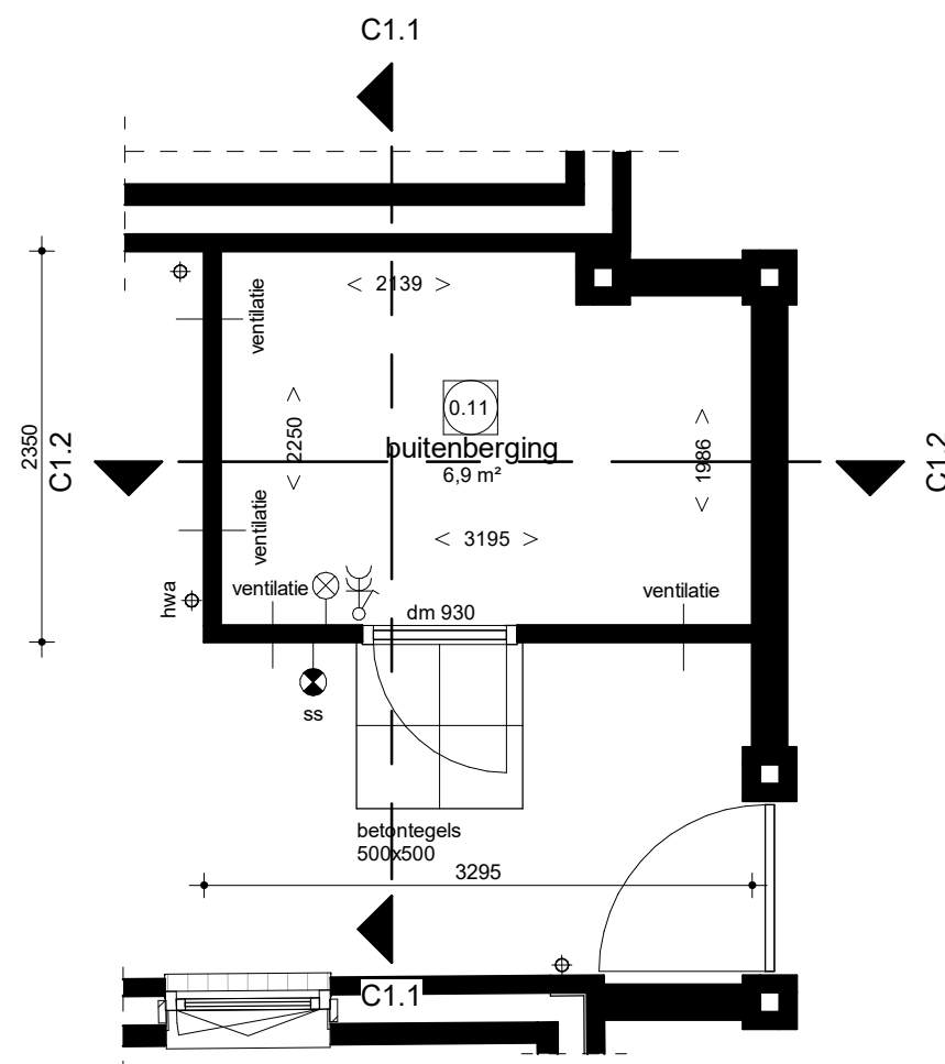
Begane grond
