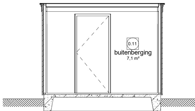
Doorsnede D1.1
