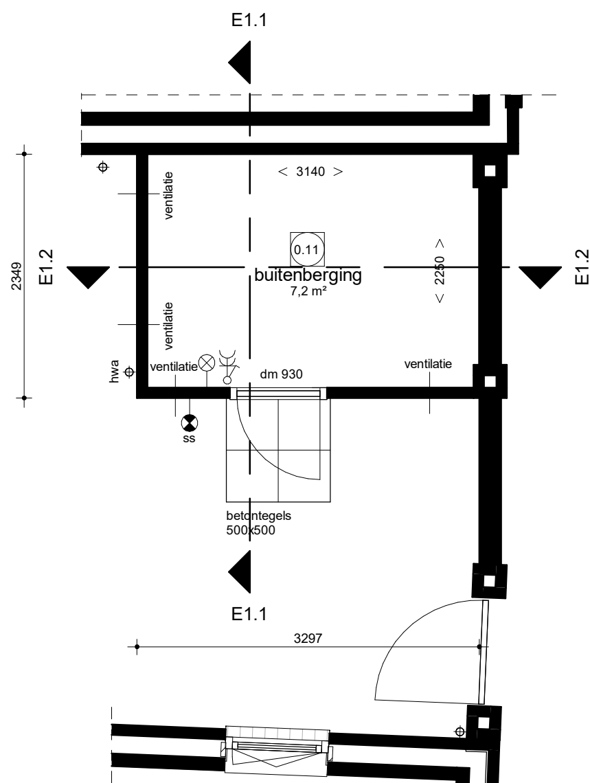
Begane grond
