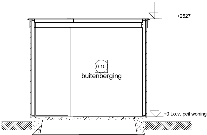
Doorsnede V
