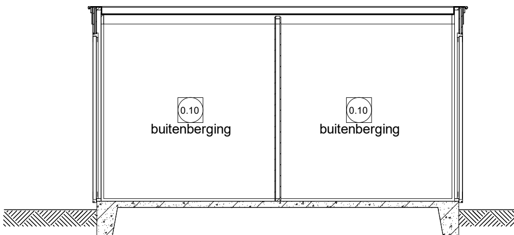
Doorsnede Q
