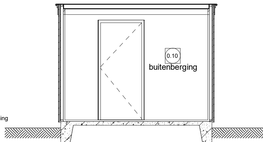
Doorsnede Y
