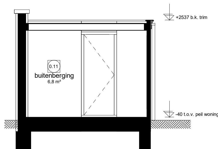
Doorsnede G1.2
