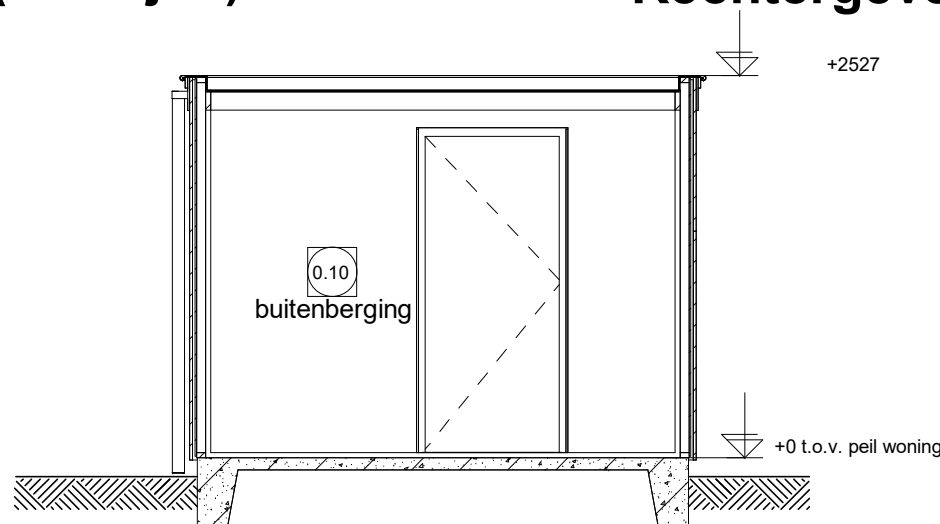
Doorsnede P
