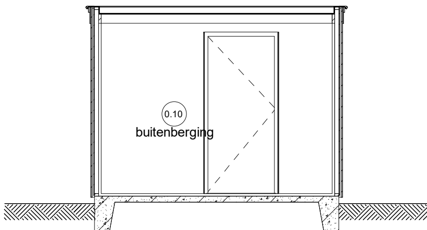
Doorsnede G
