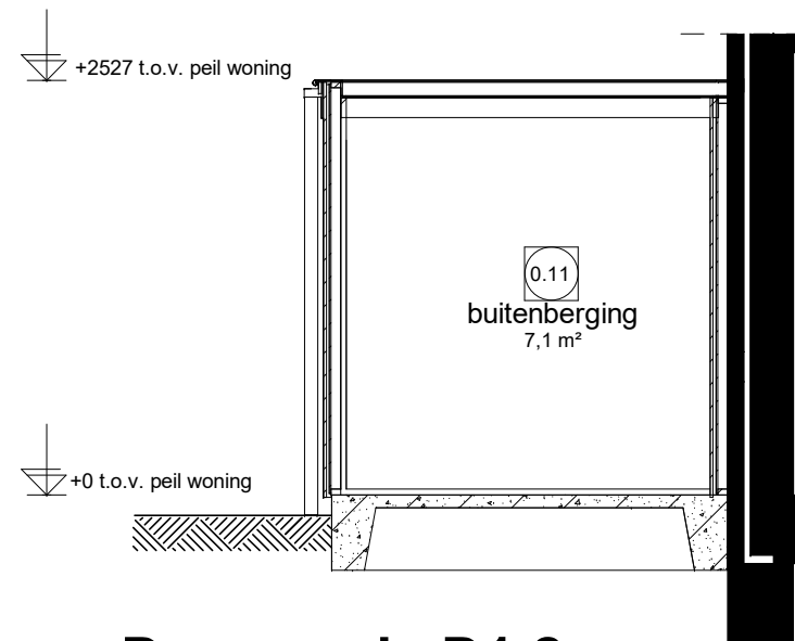
Doorsnede D1.2
