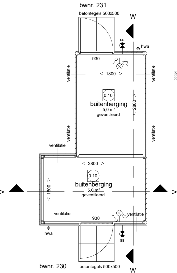
Begane grond
