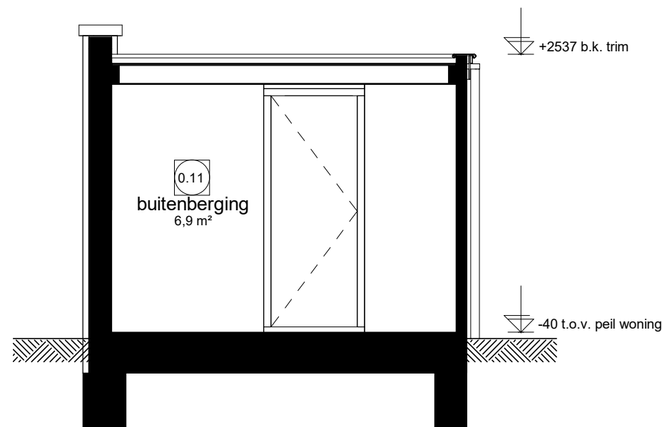
Doorsnede C1.2
