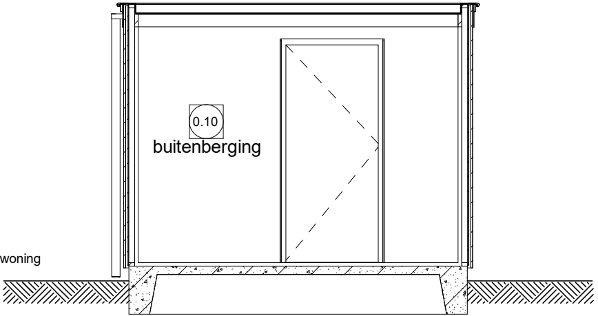
Doorsnede S
