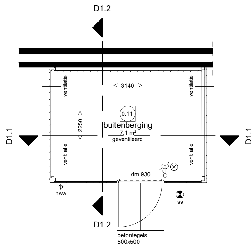
Begane grond
