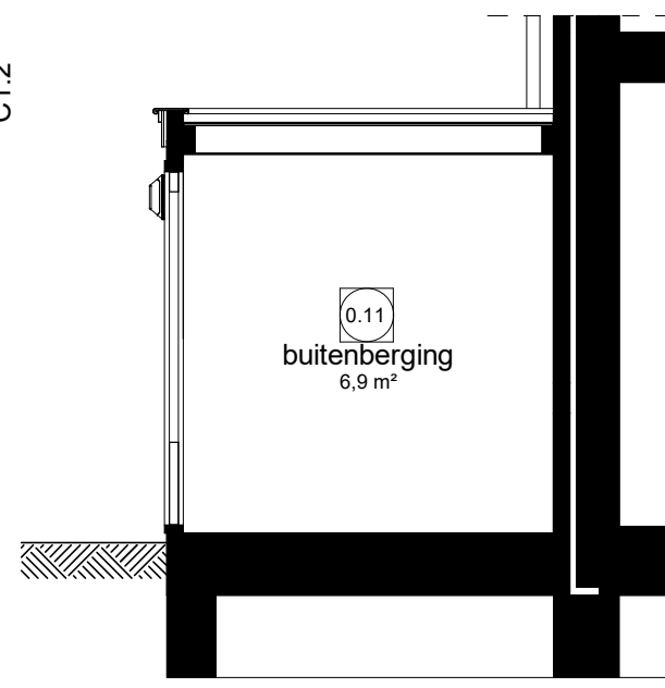
Doorsnede C1.1
