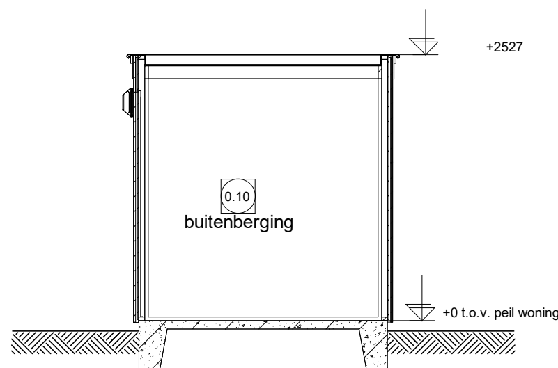
Doorsnede F
