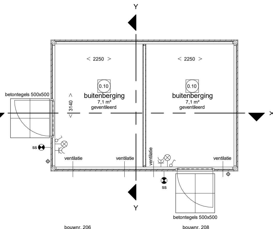
Begane grond
