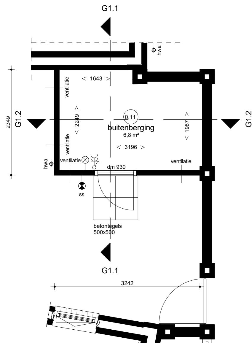
Begane grond
