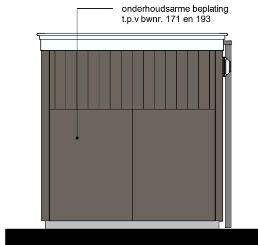
Linkergevel
