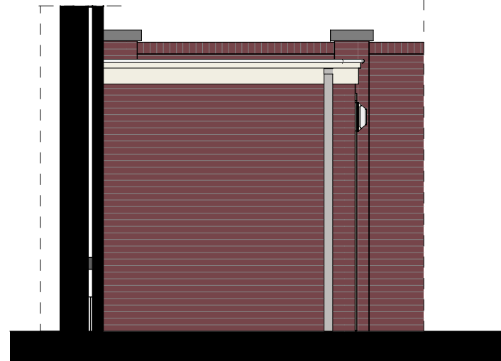
Linkergevel
