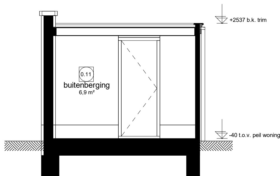
Doorsnede F1.1
