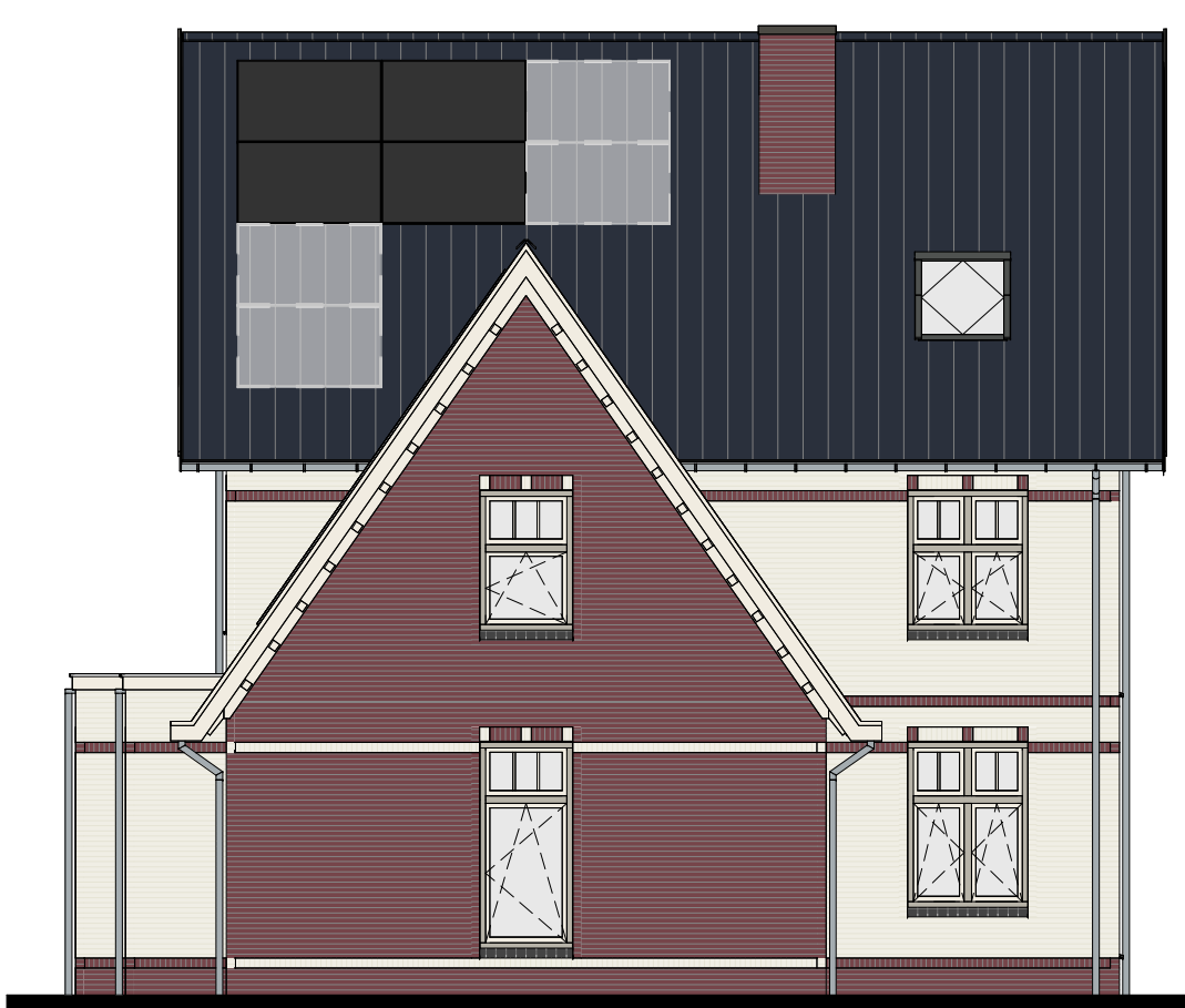
Linkergevel
