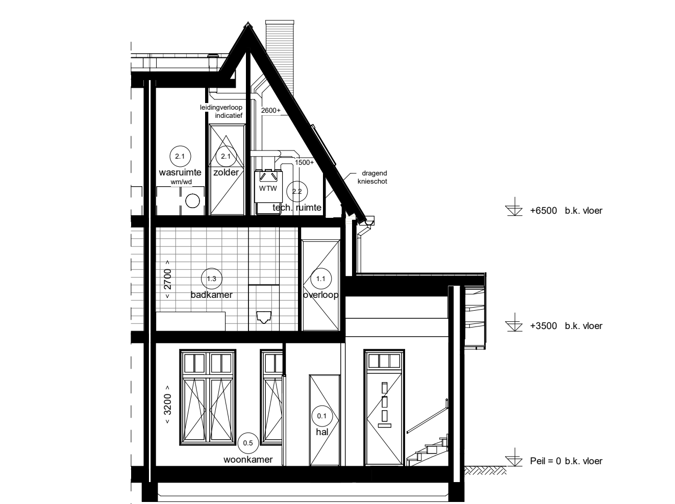
Doorsnede D04.3
