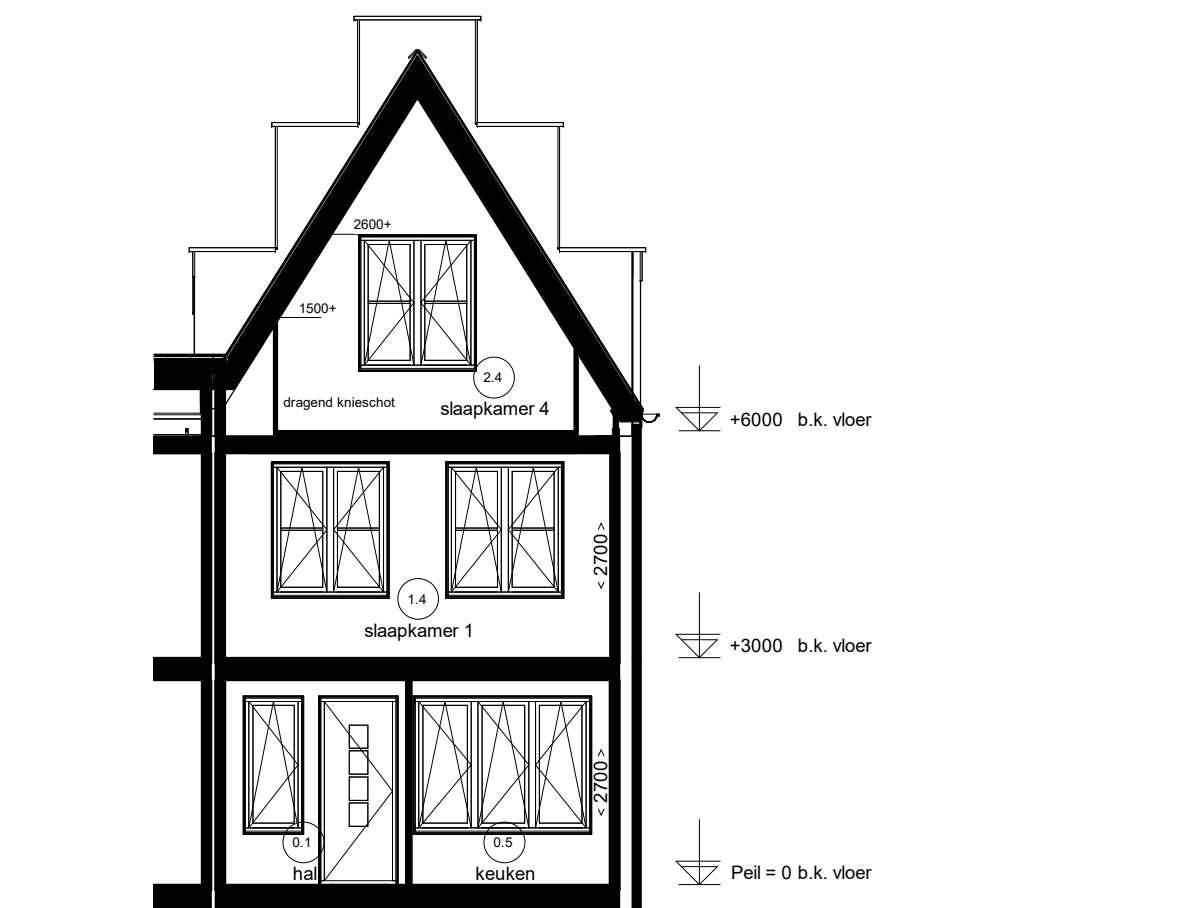
Doorsnede D3.C
