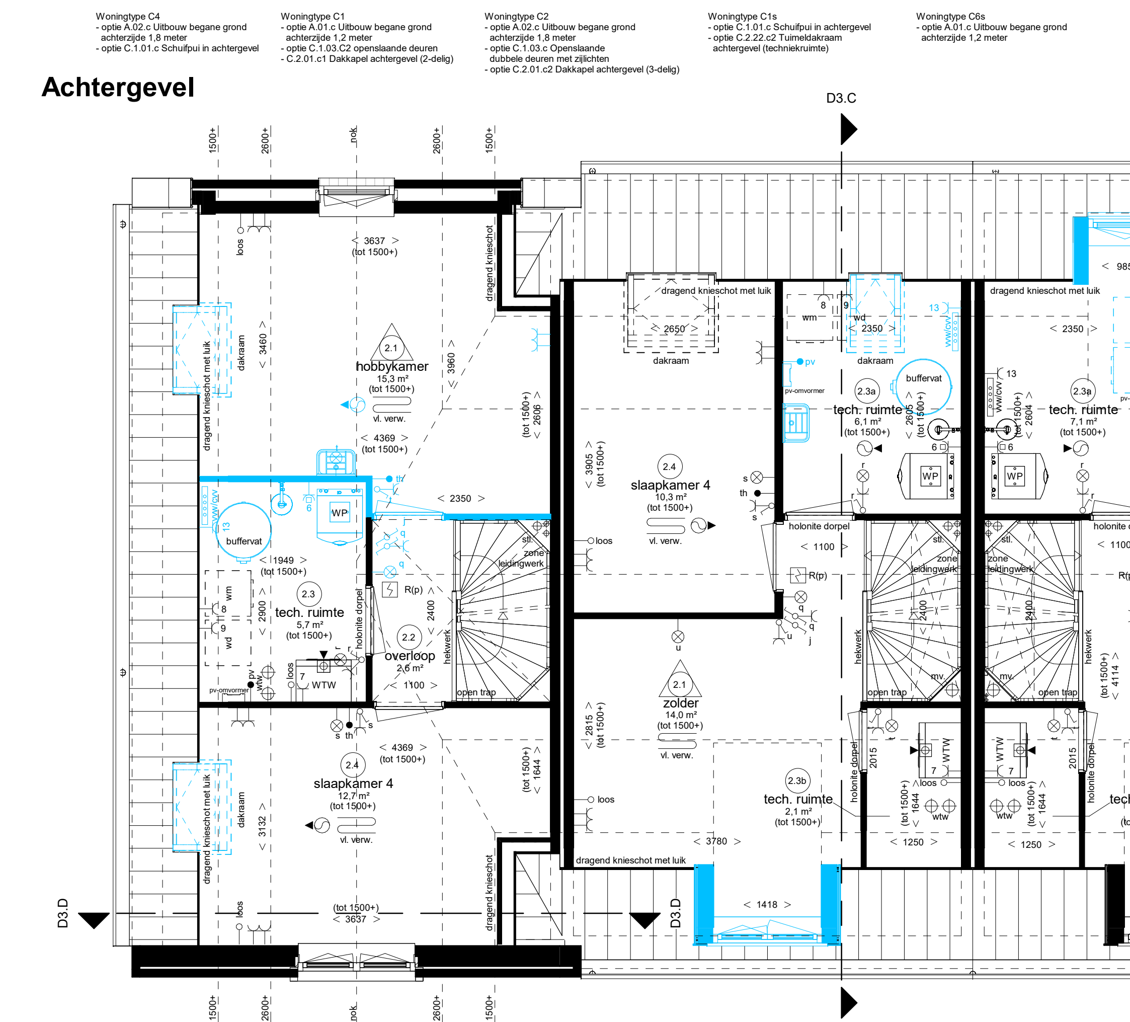
Tweede verdieping
