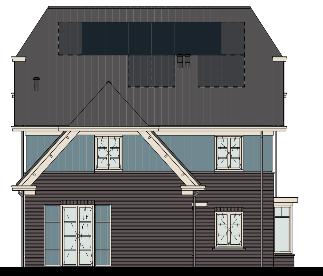
linker zijgevel
