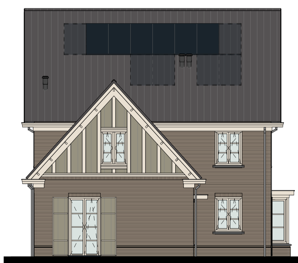
linker zijgevel
