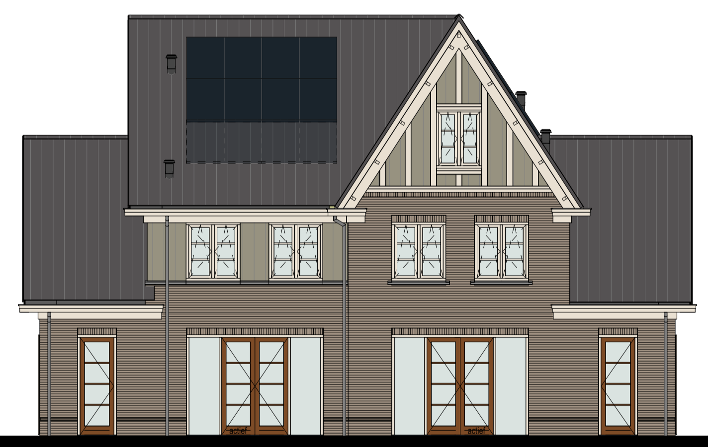
achtergevel
