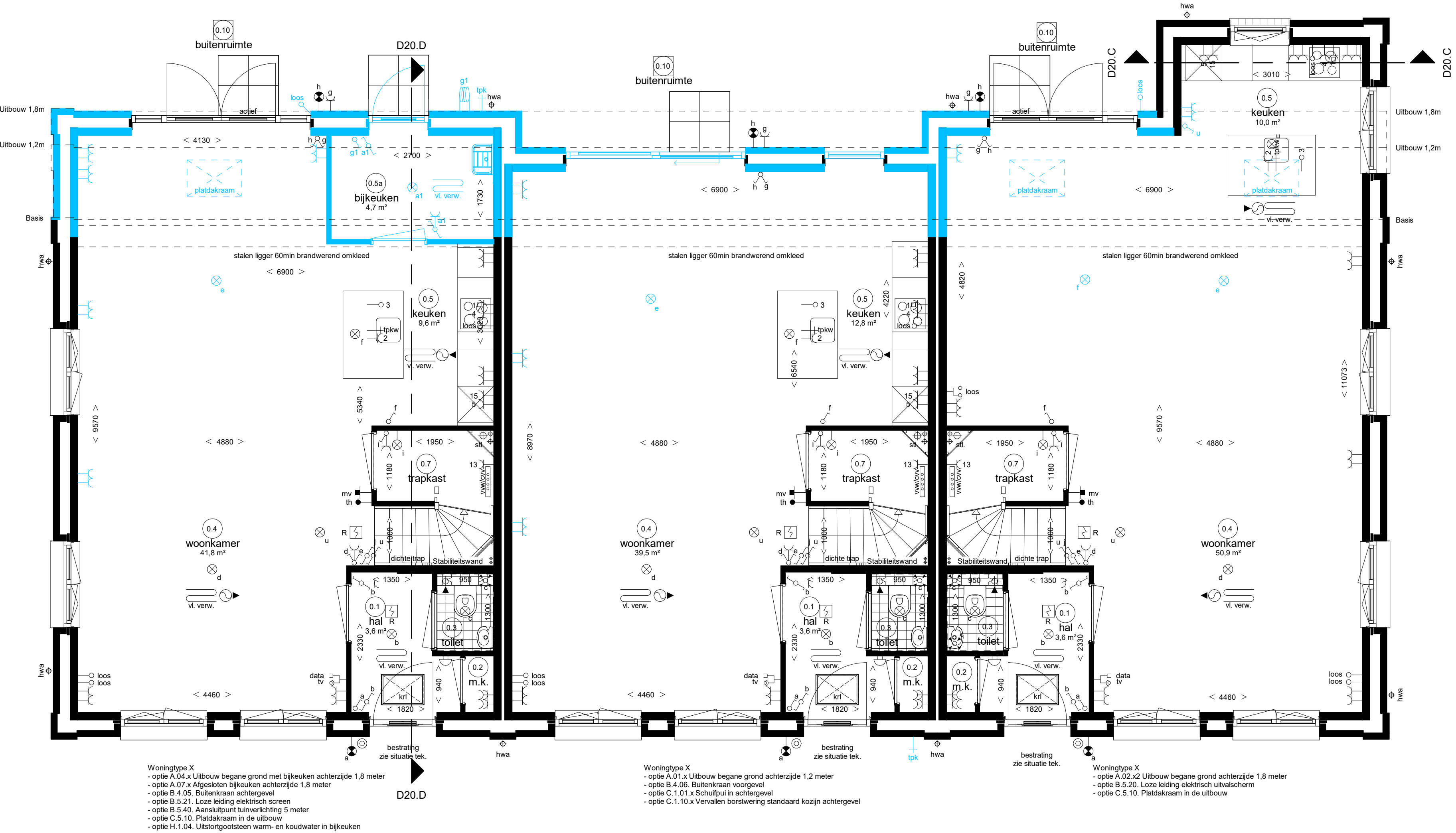
Begane grond
