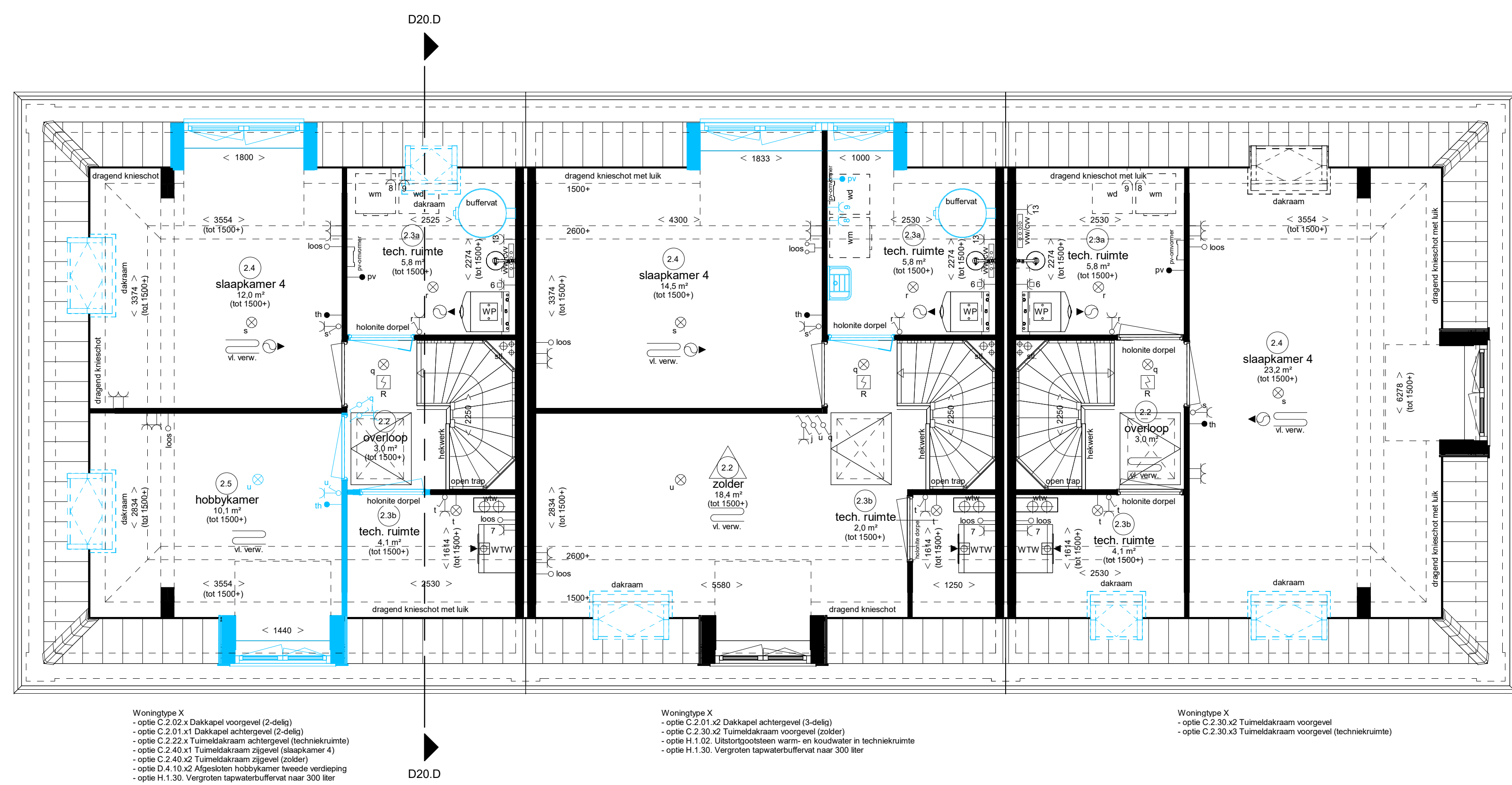
Tweede verdieping
