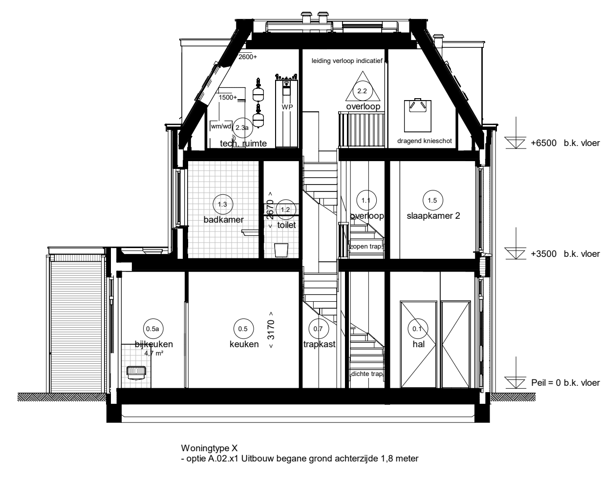
Doorsnede D20.D
