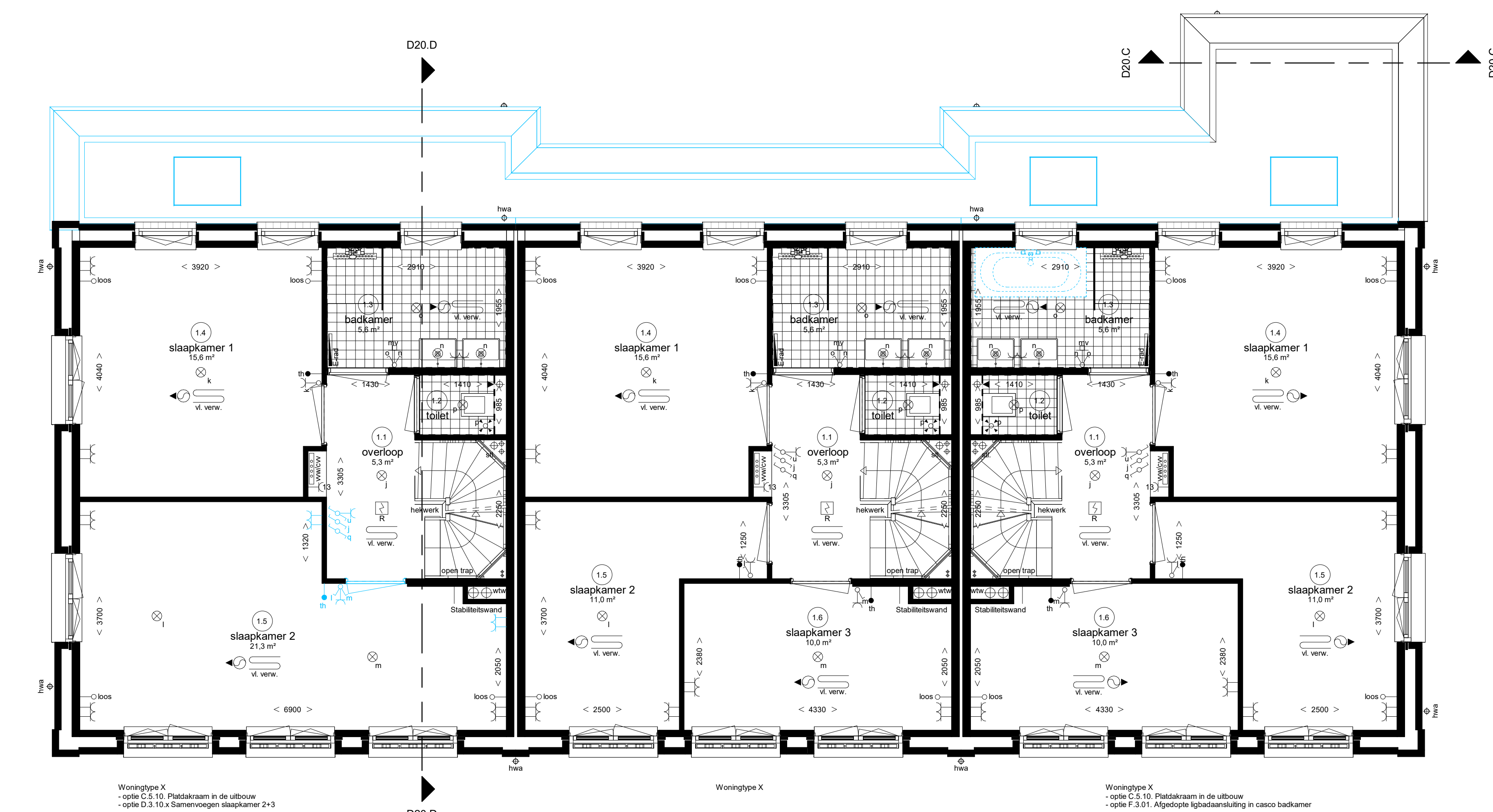
Eerste verdieping
