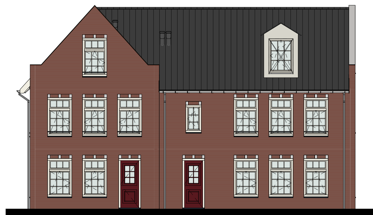
Woningtype D21s bwnr 54
