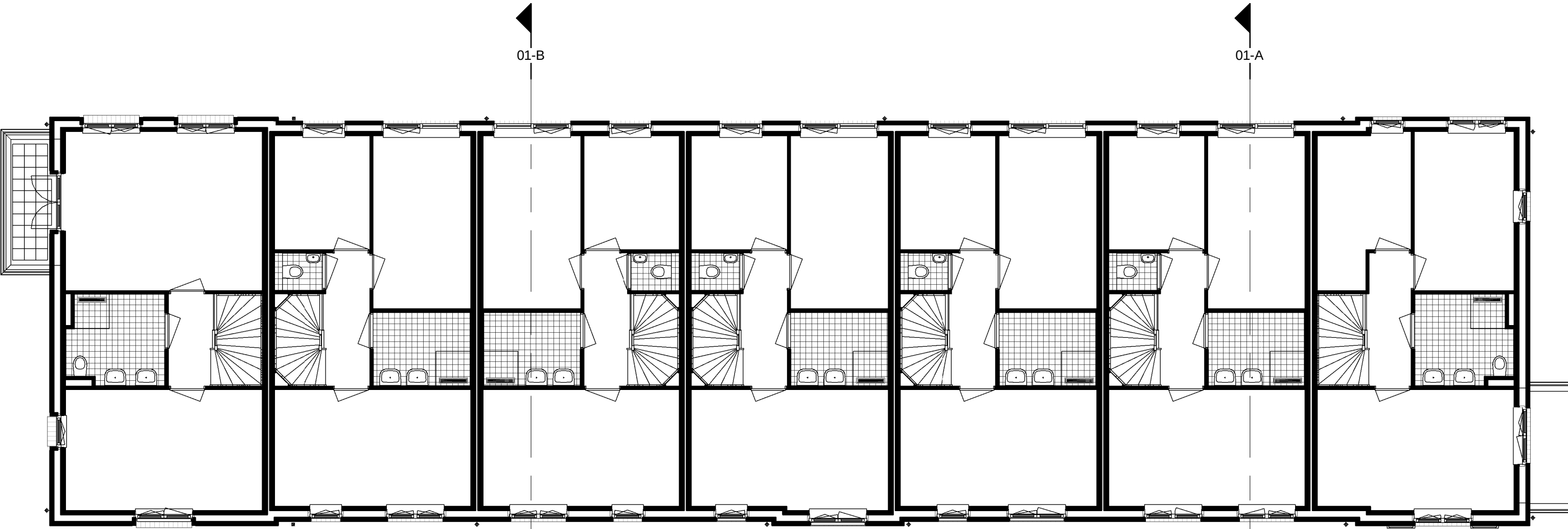
Eerste verdieping
