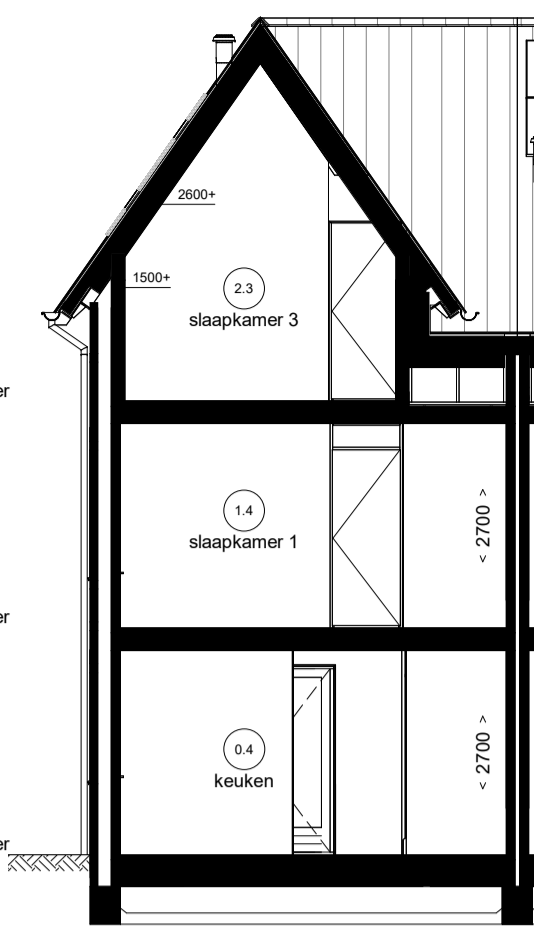
Doorsnede D11.3
