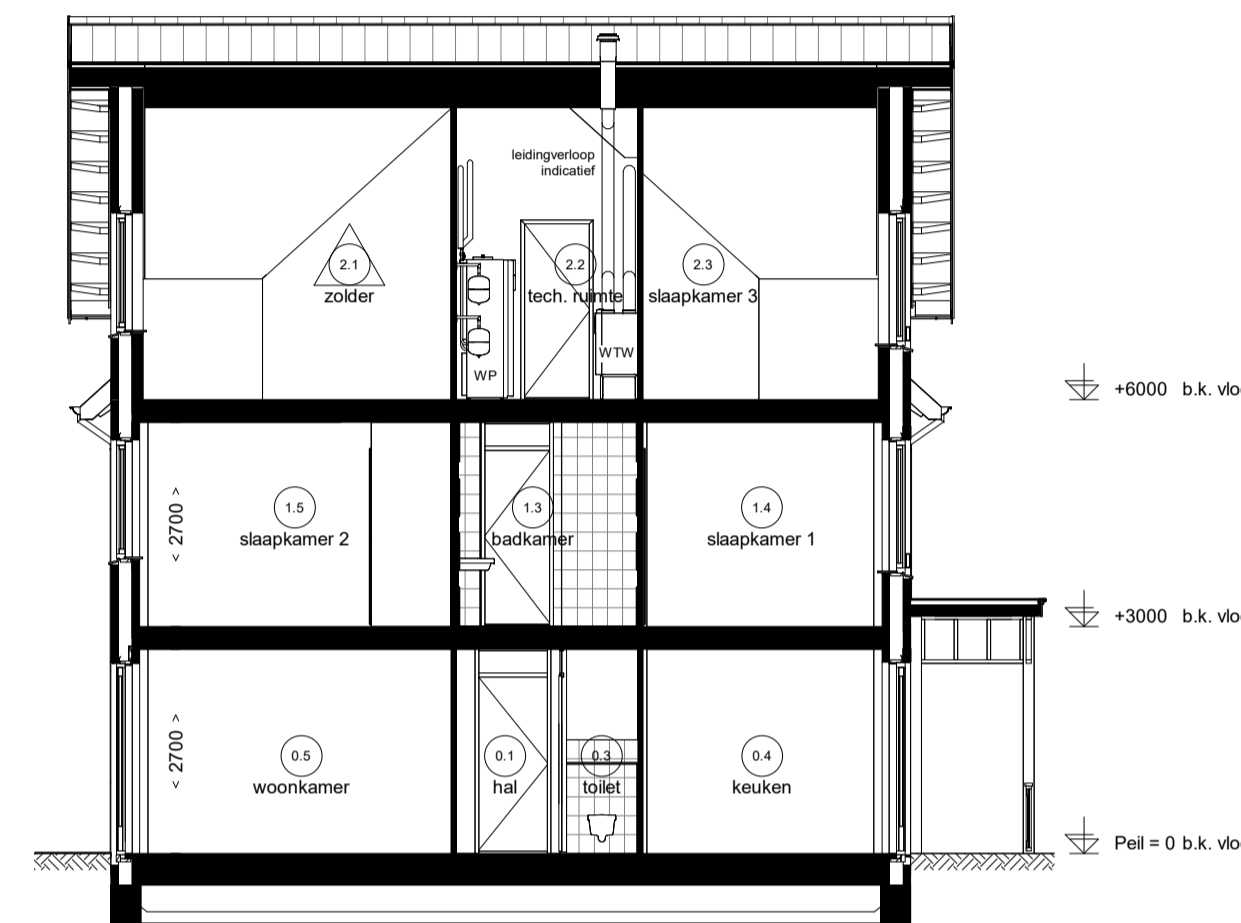
Doorsnede D11.2
