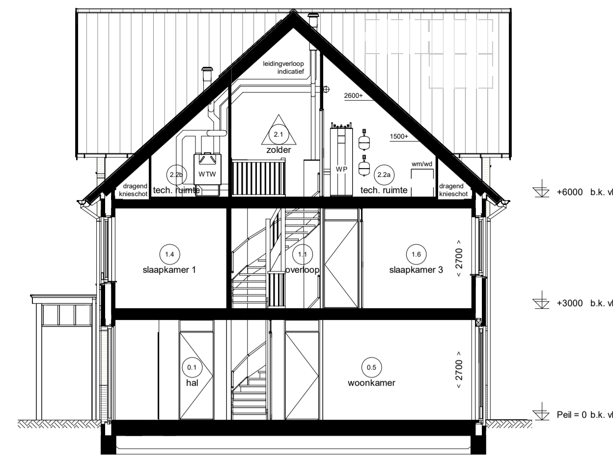
Doorsnede D11.1
