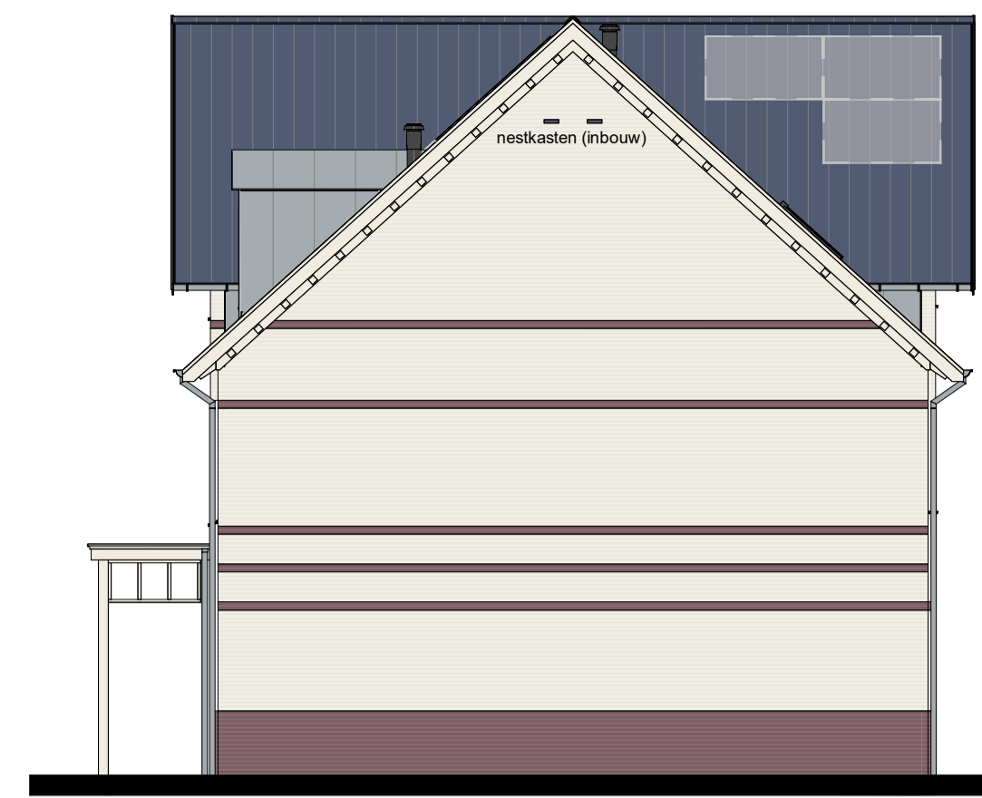
Woningtype C2s bwnr 338 Rechtergevel
