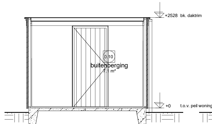
Doorsnede 5.1
