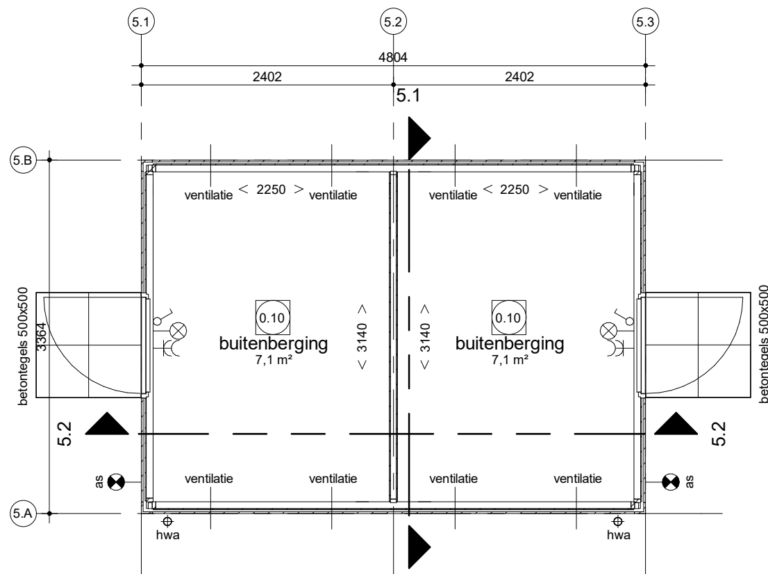
Begane grond
