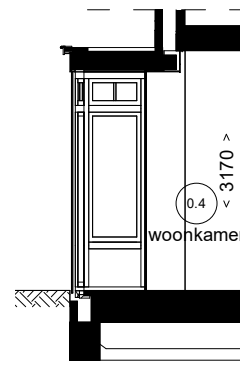
Doorsnede D12.6
