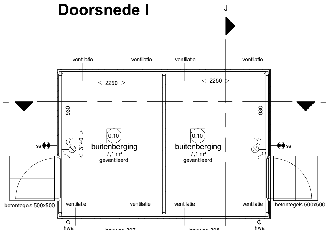
Begane grond
