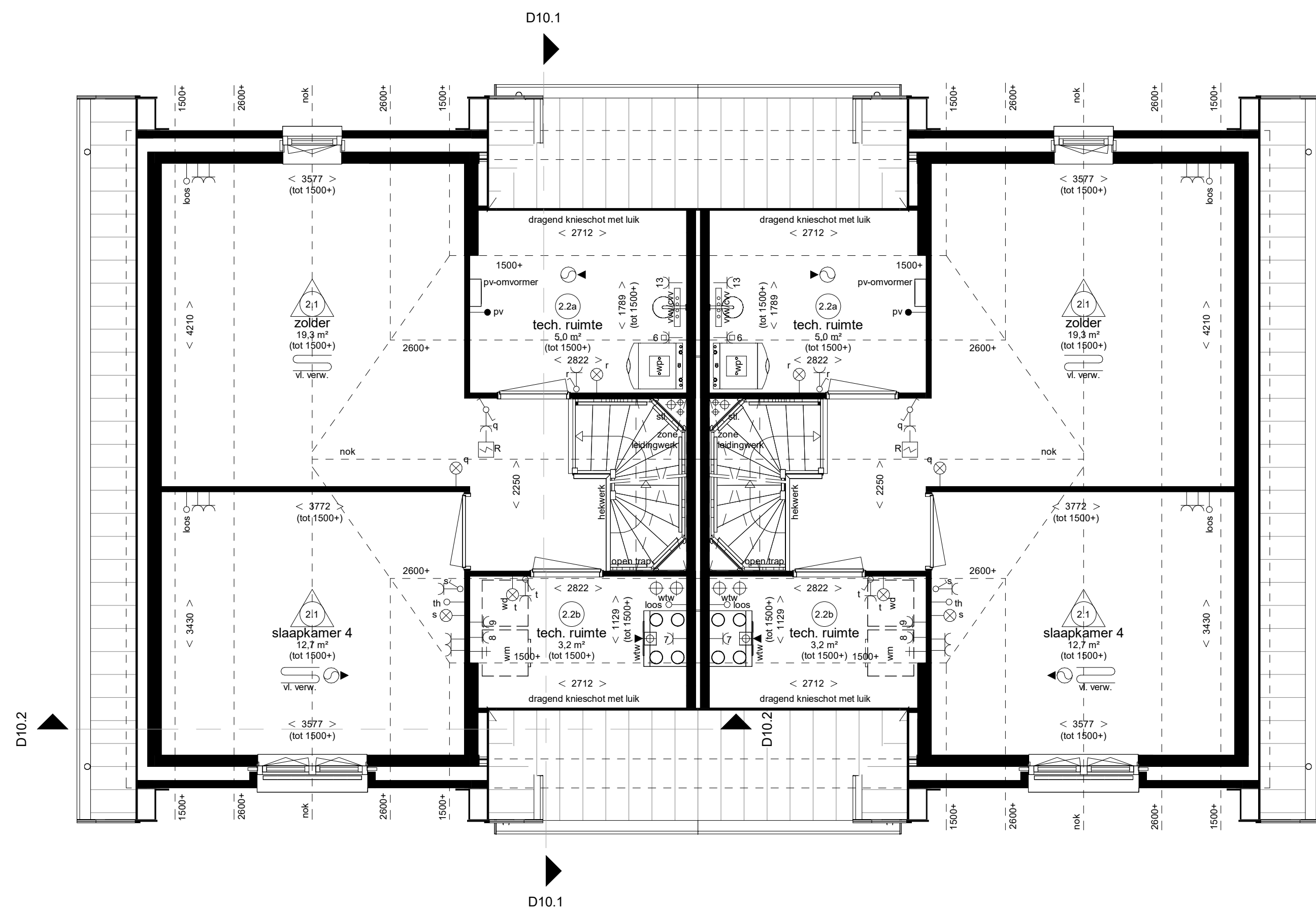
Woningtype X3sv bwnr 337 Tweede verdieping
