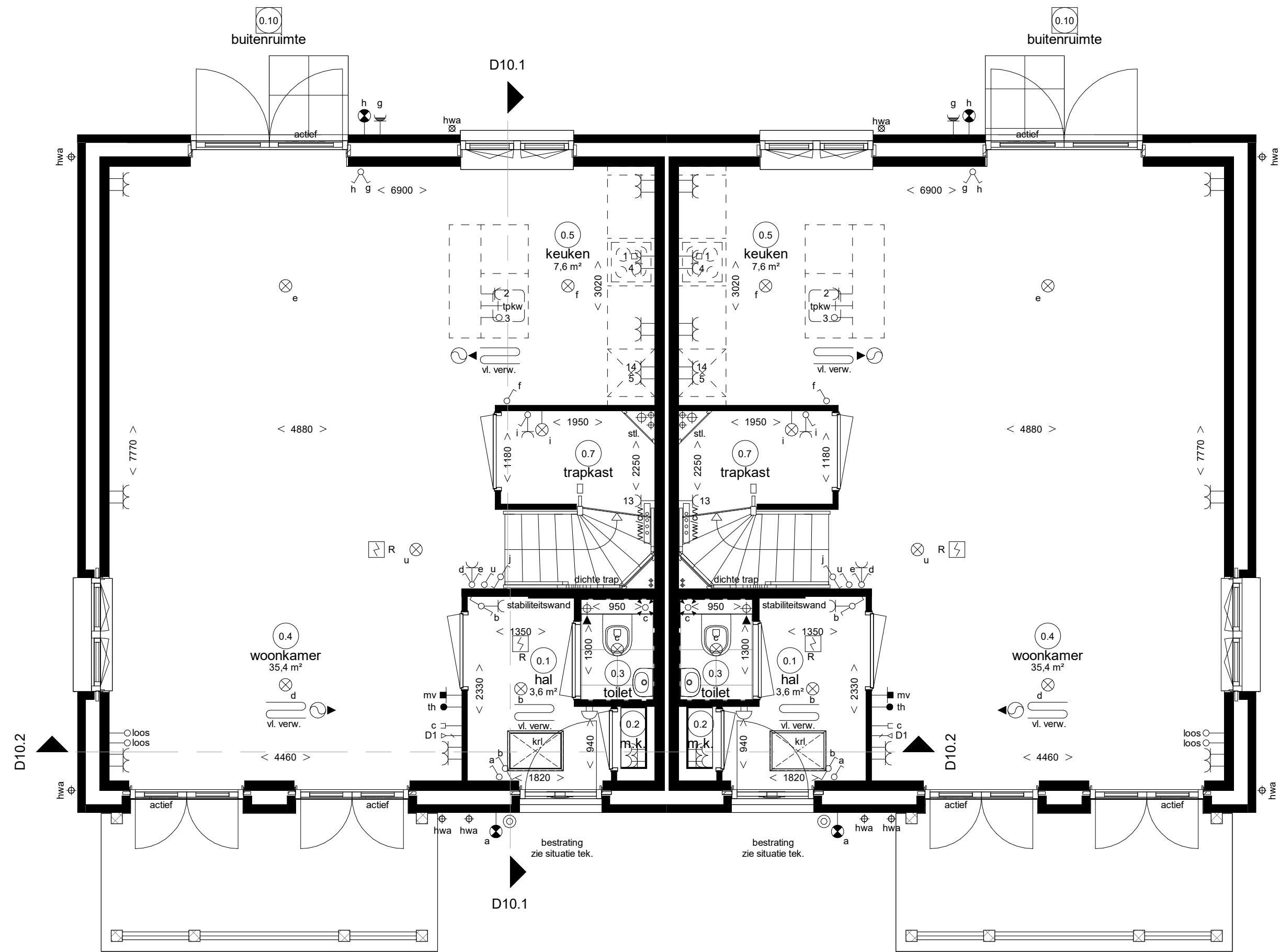
Woningtype X3sv bwnr 337 Begane grond
