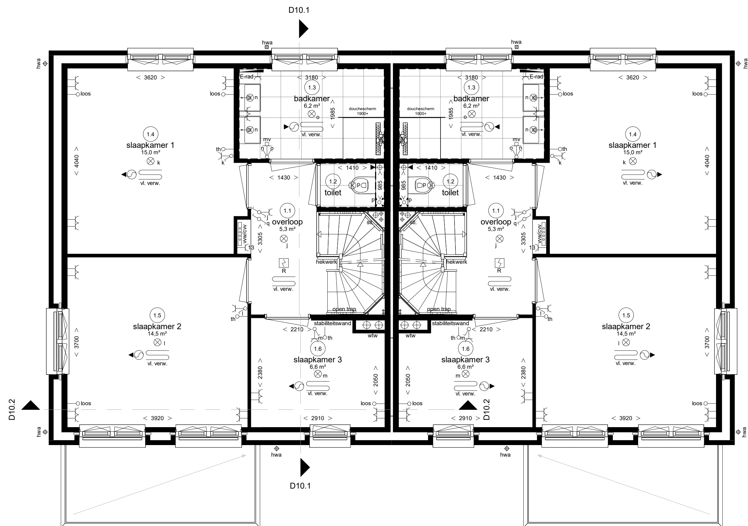
Woningtype X3sv bwnr 337 Eerste verdieping
