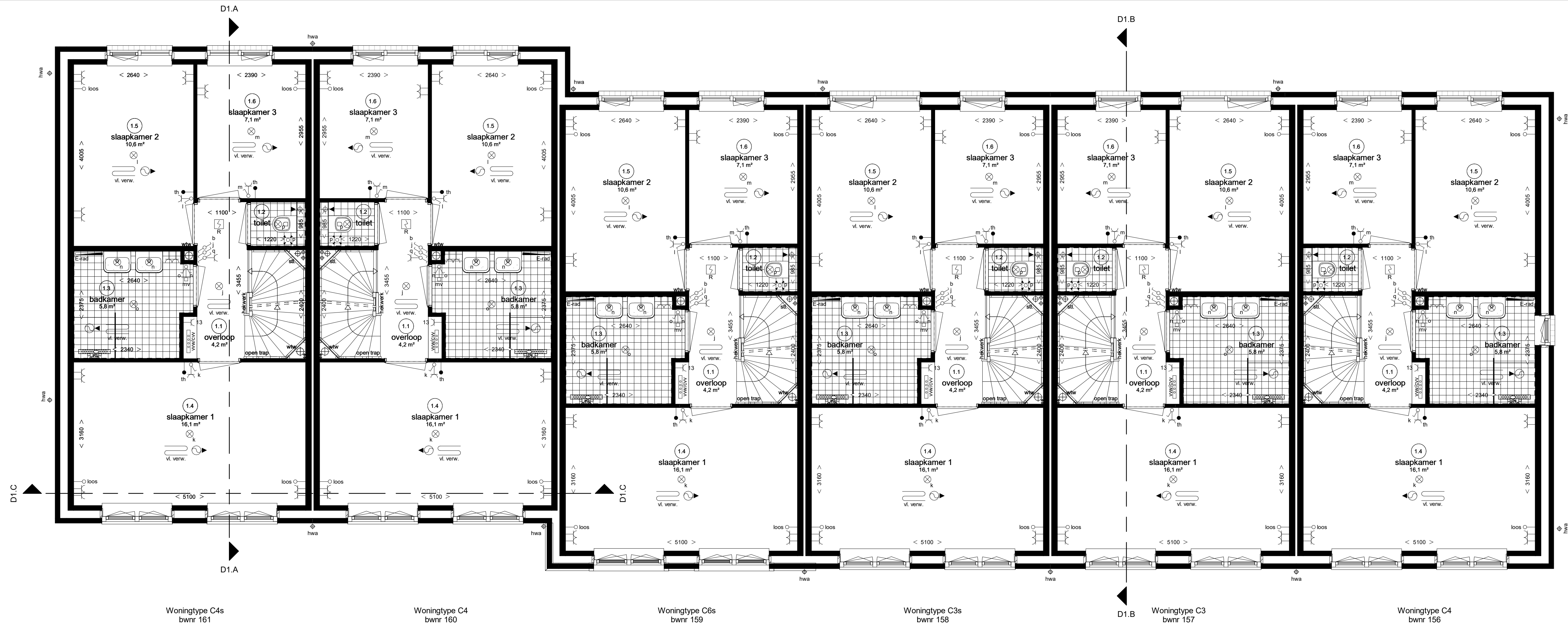
Eerste verdieping
