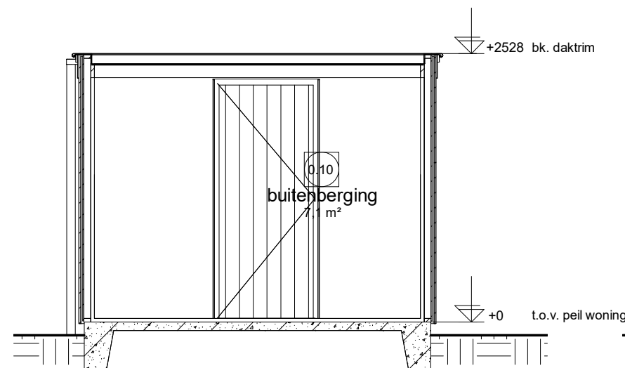
Doorsnede 4.1
