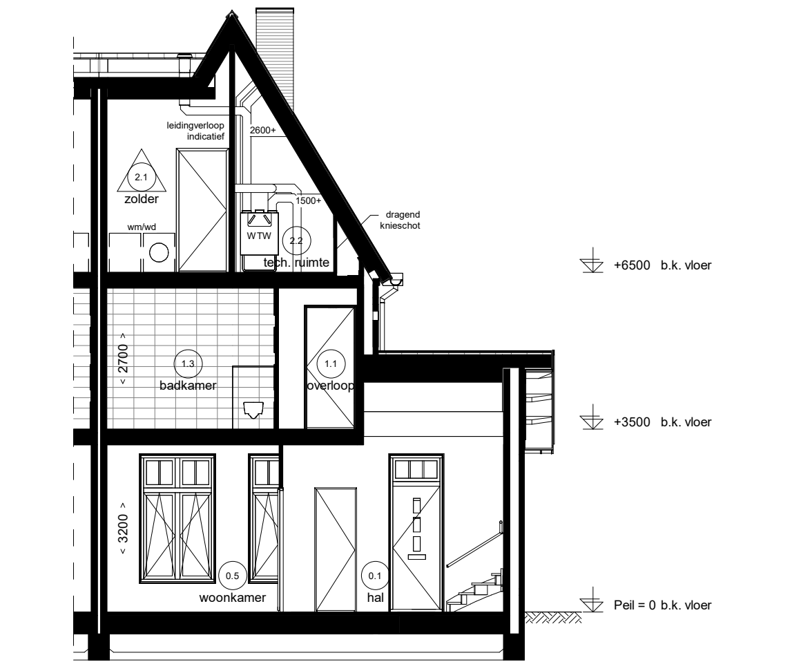
Doorsnede D04.1
