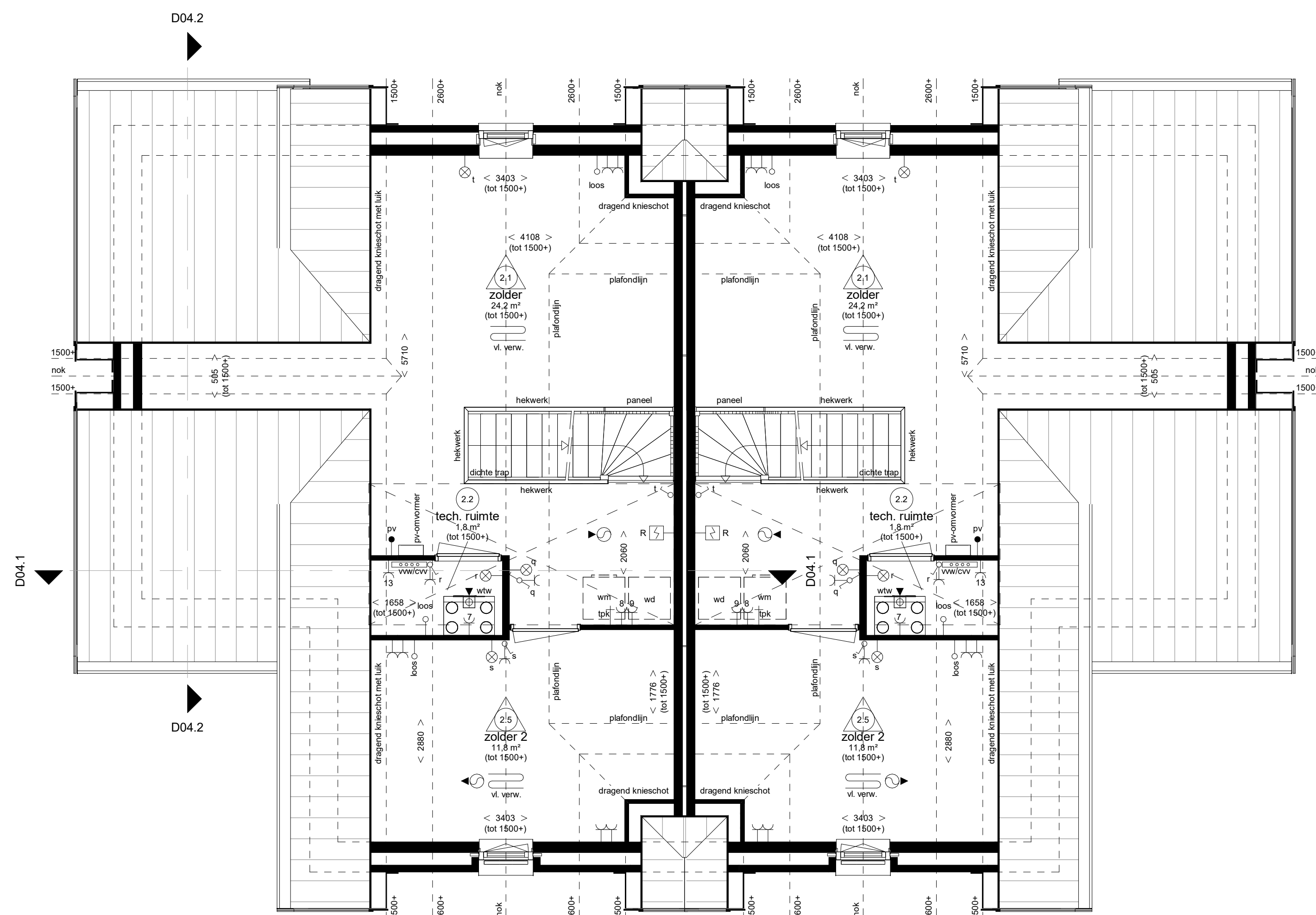
Woningtype J1 bwnr 322 Woningtype J1s bwnr 321 Tweede verdieping
