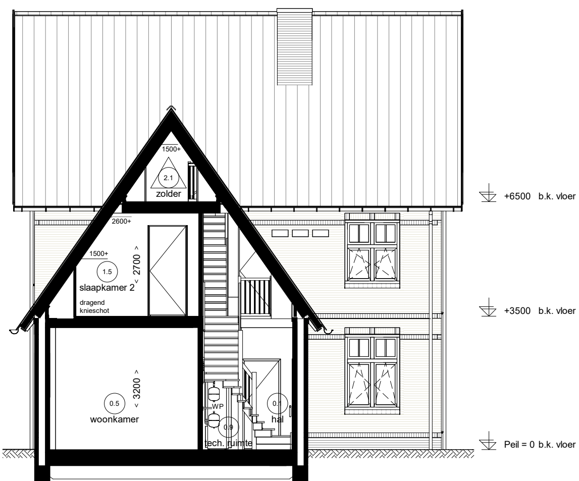
Doorsnede D04.2
