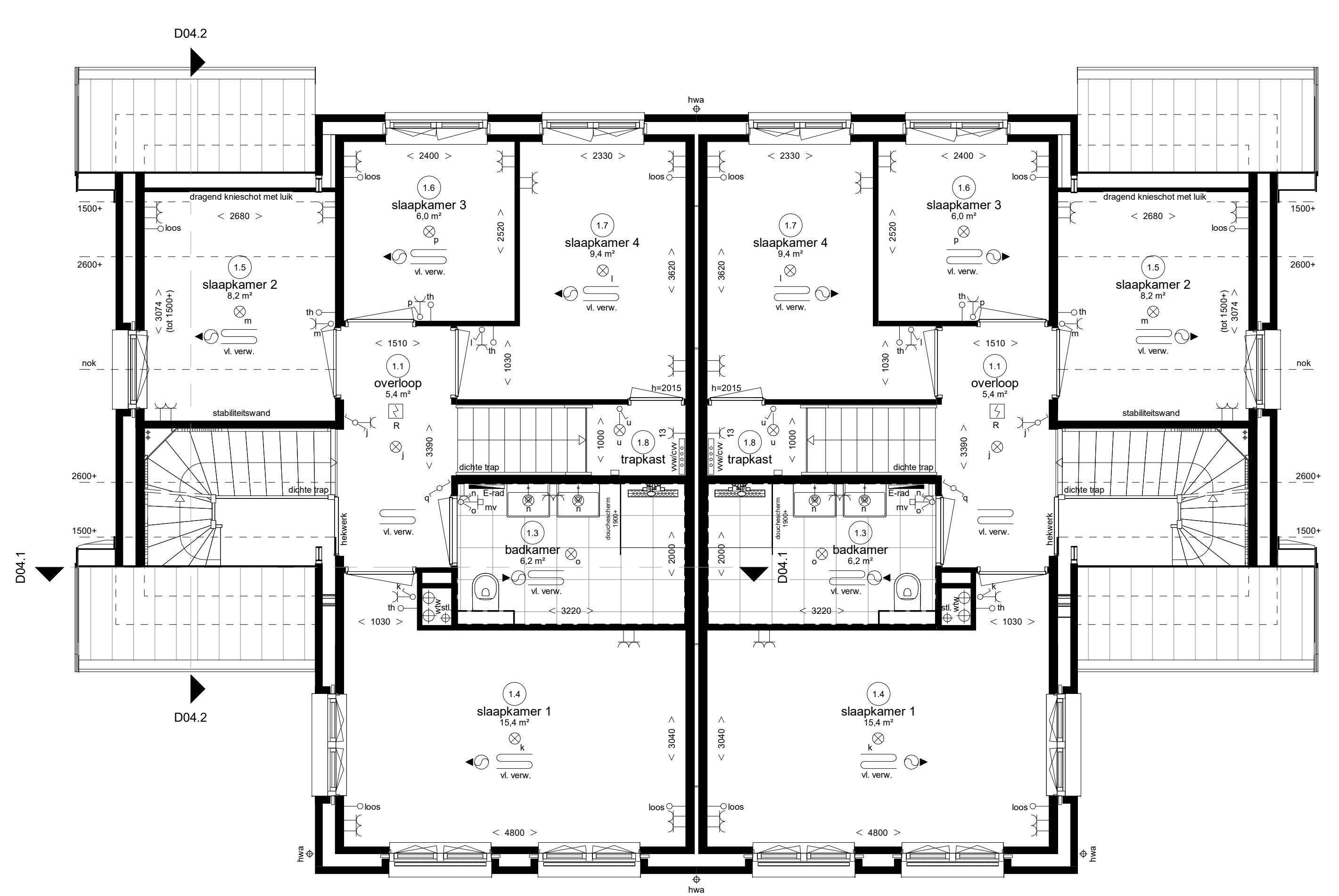
Woningtype J1 bwnr 322 Woningtype J1s bwnr 321 Eerste verdieping
