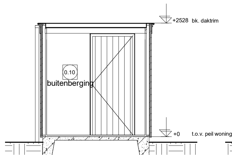
Doorsnede 7.1
