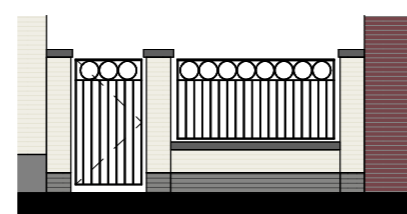
Vooraanzicht
