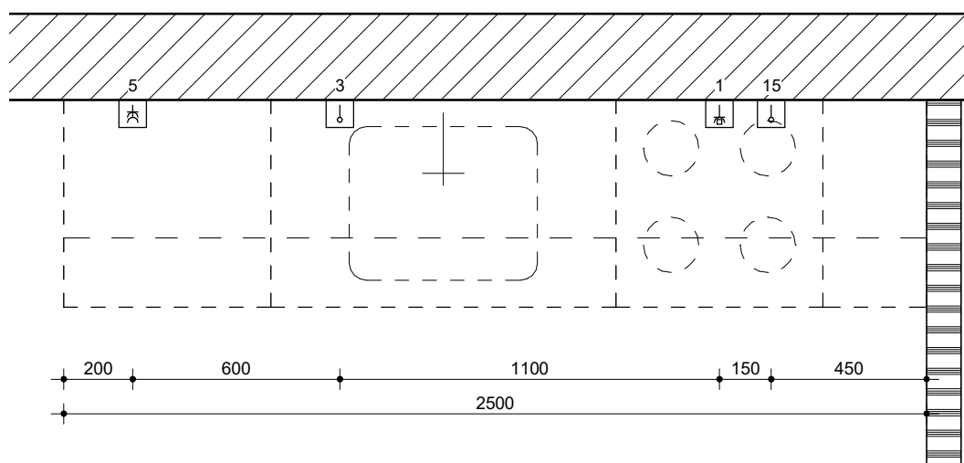
Plattegrond keuken
