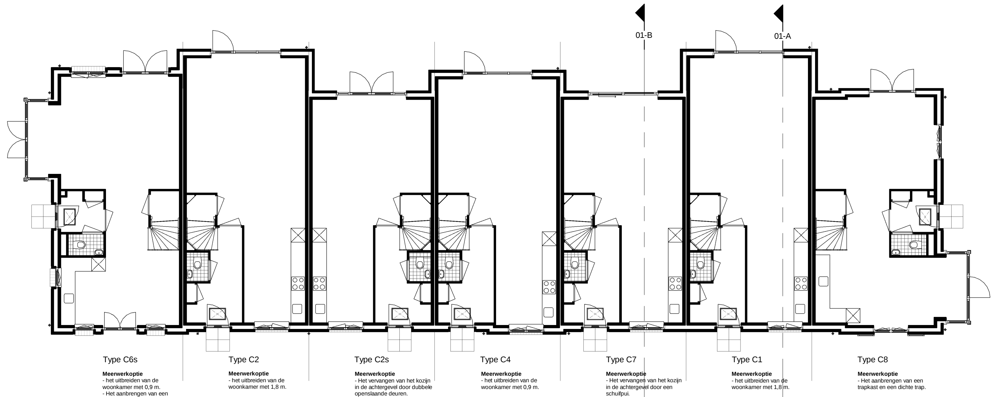
Begane grond
