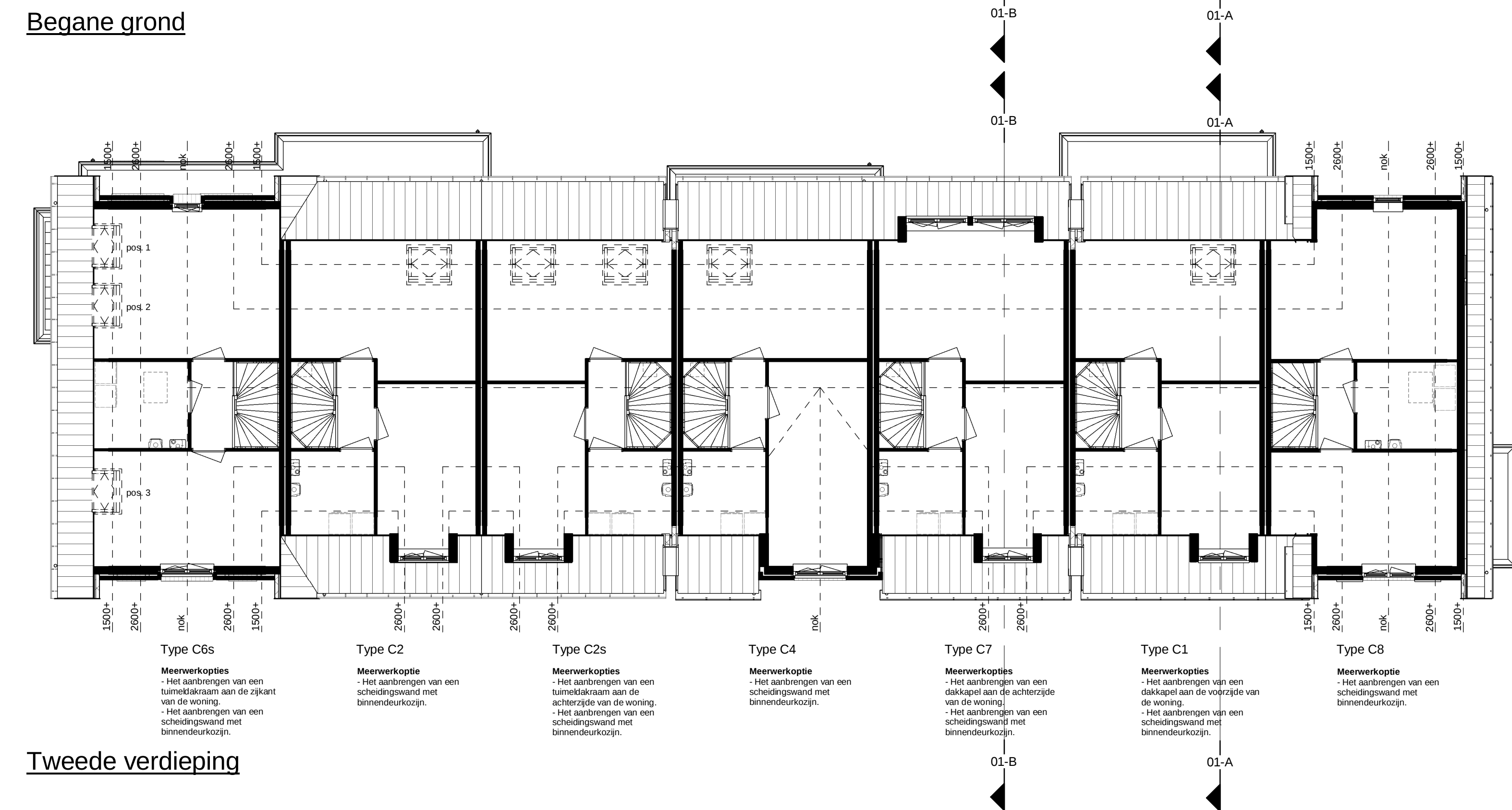
Begane grond
