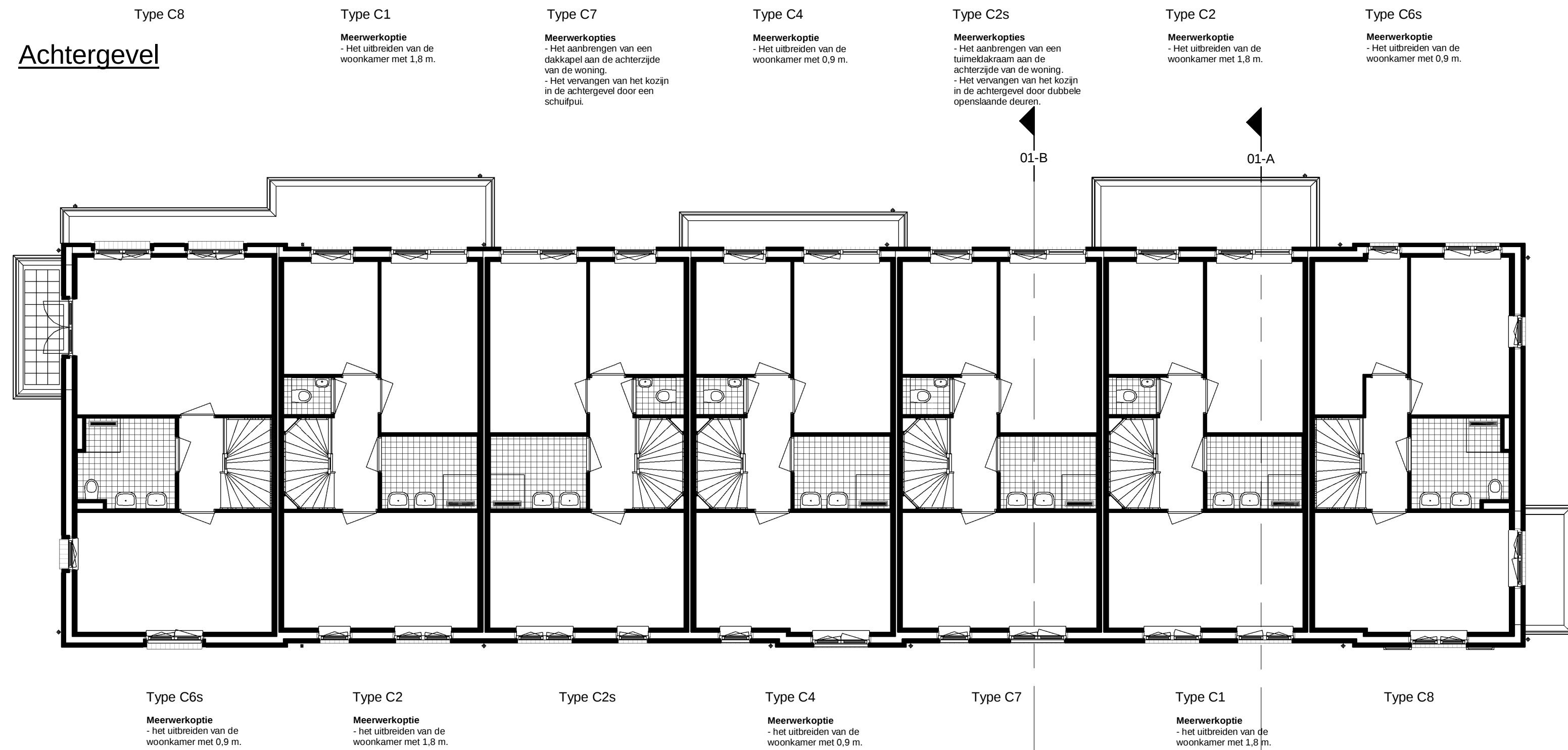
Eerste verdieping
