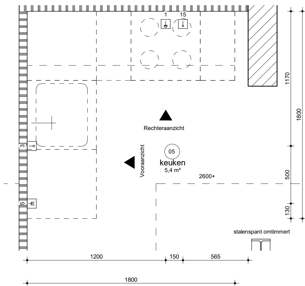
Plattegrond keuken
