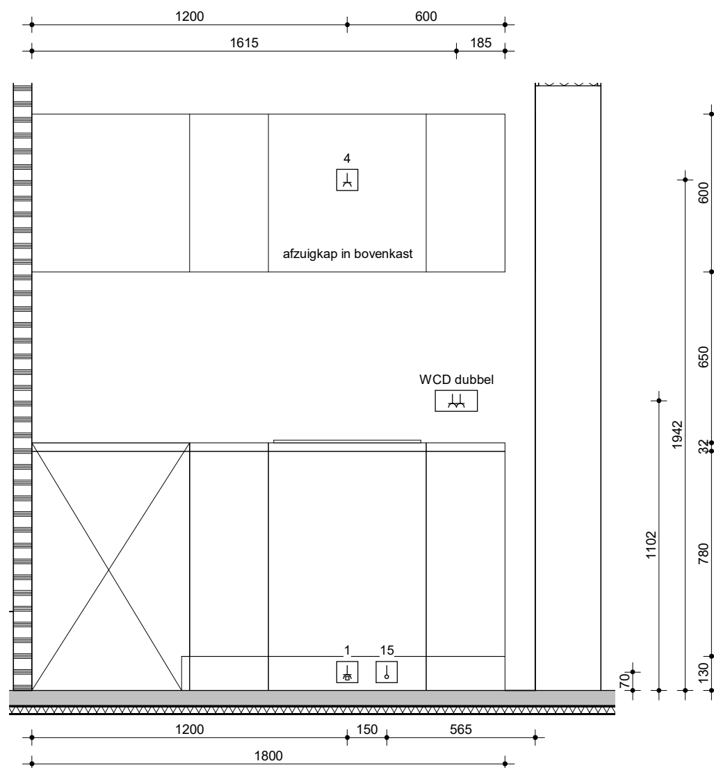
Rechter aanzicht
