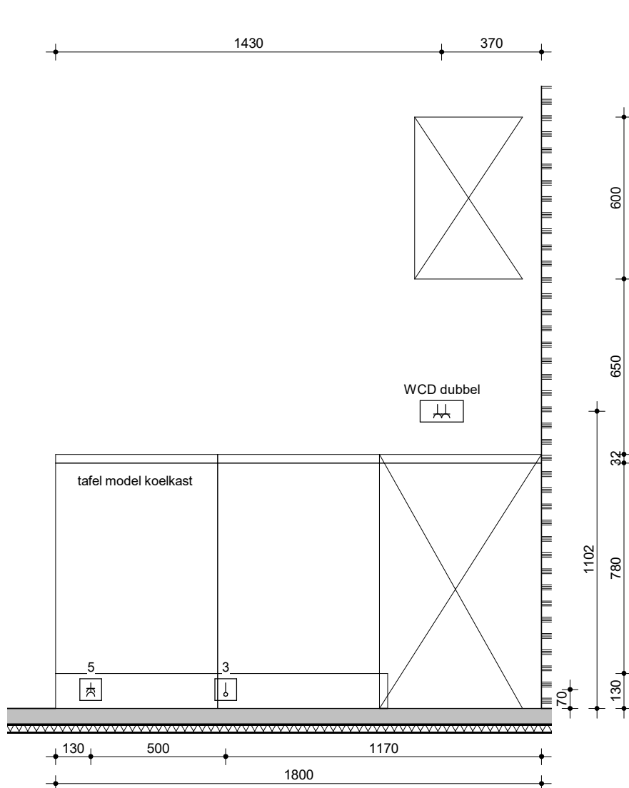
Vooraanzicht
