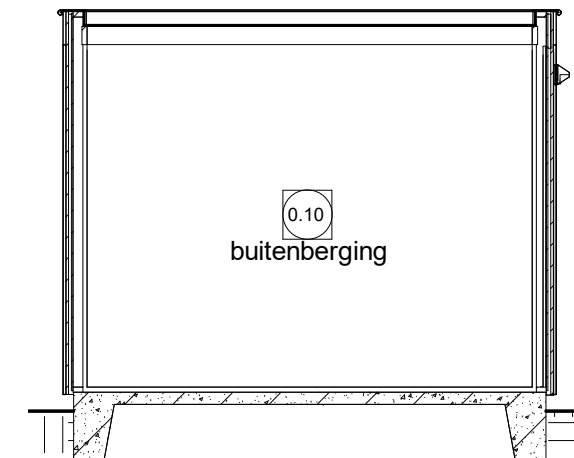
Doorsnede 18.2
