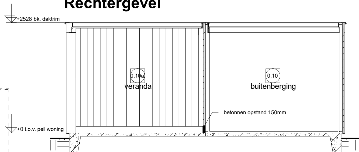
Doorsnede 18.1
