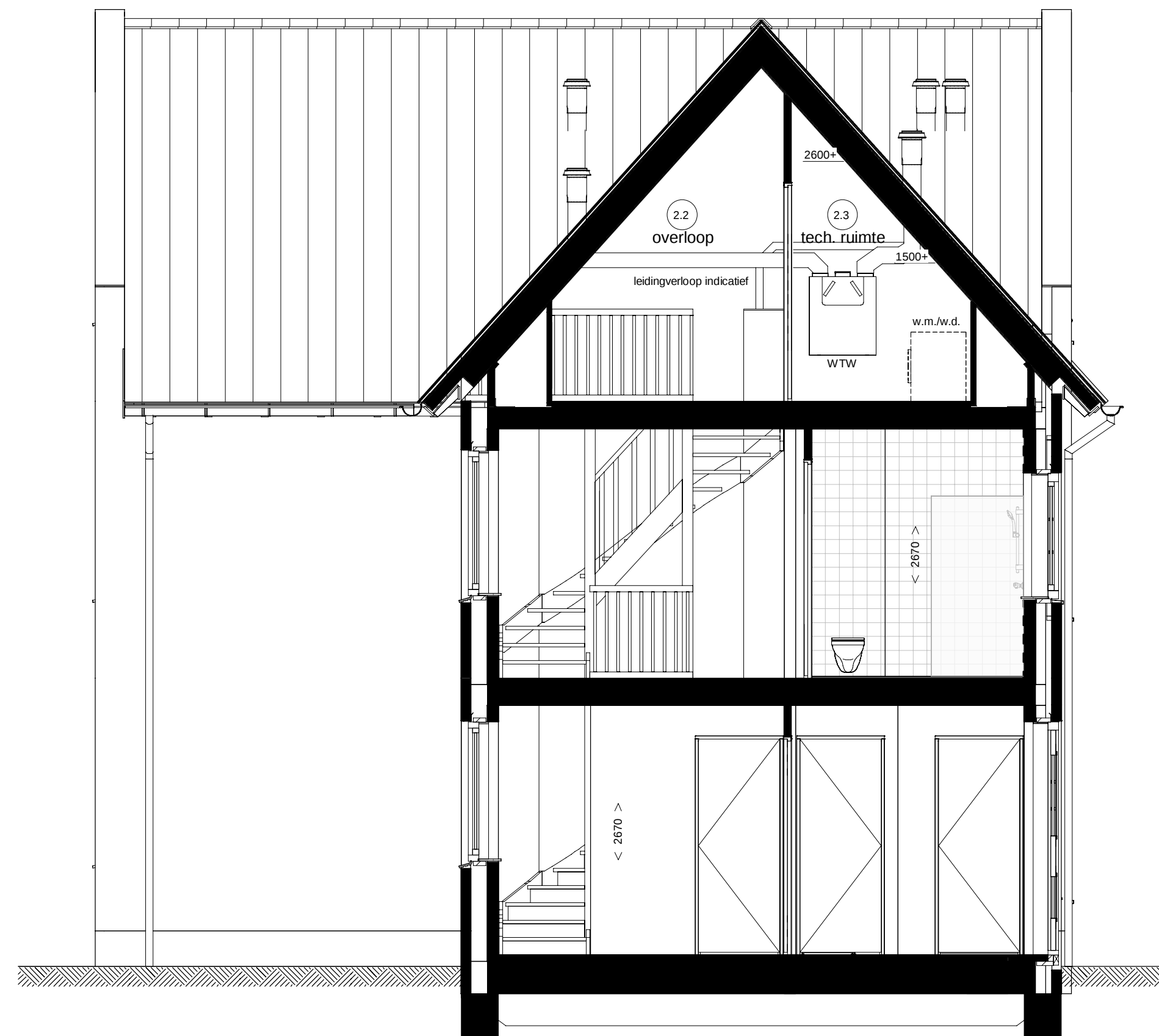
Doorsnede D10.A
