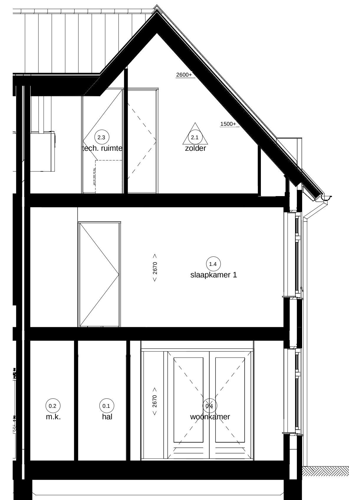
Doorsnede D10.B
