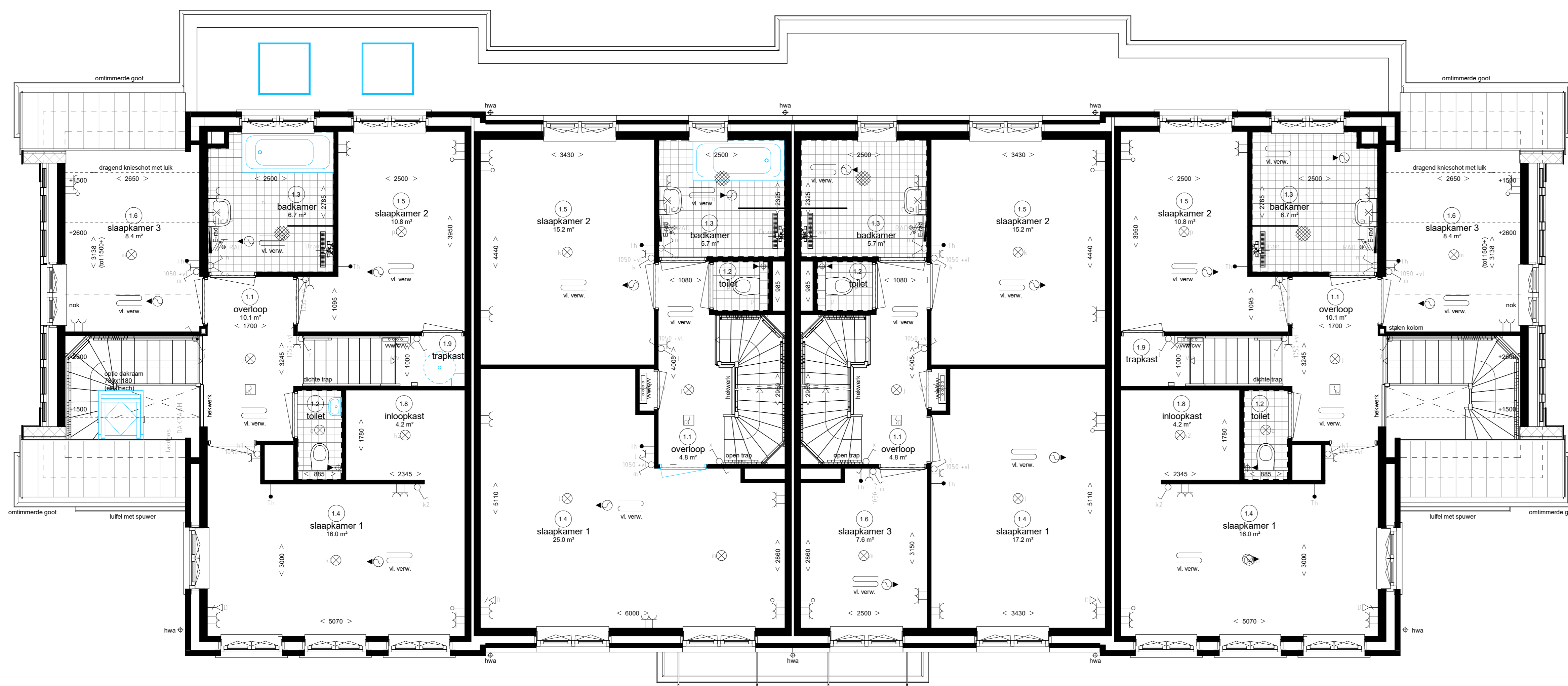
eerste verdieping
