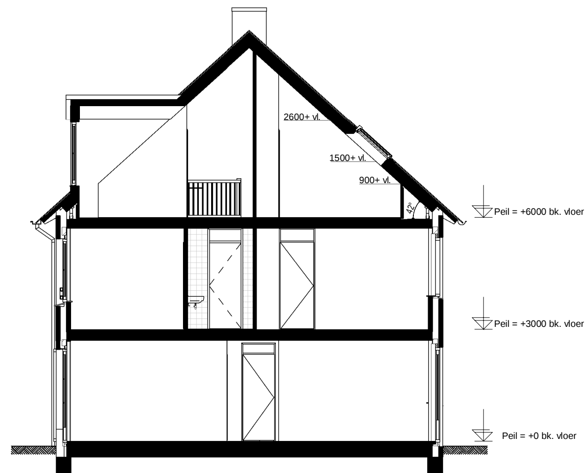
Doorsnede 11-B
