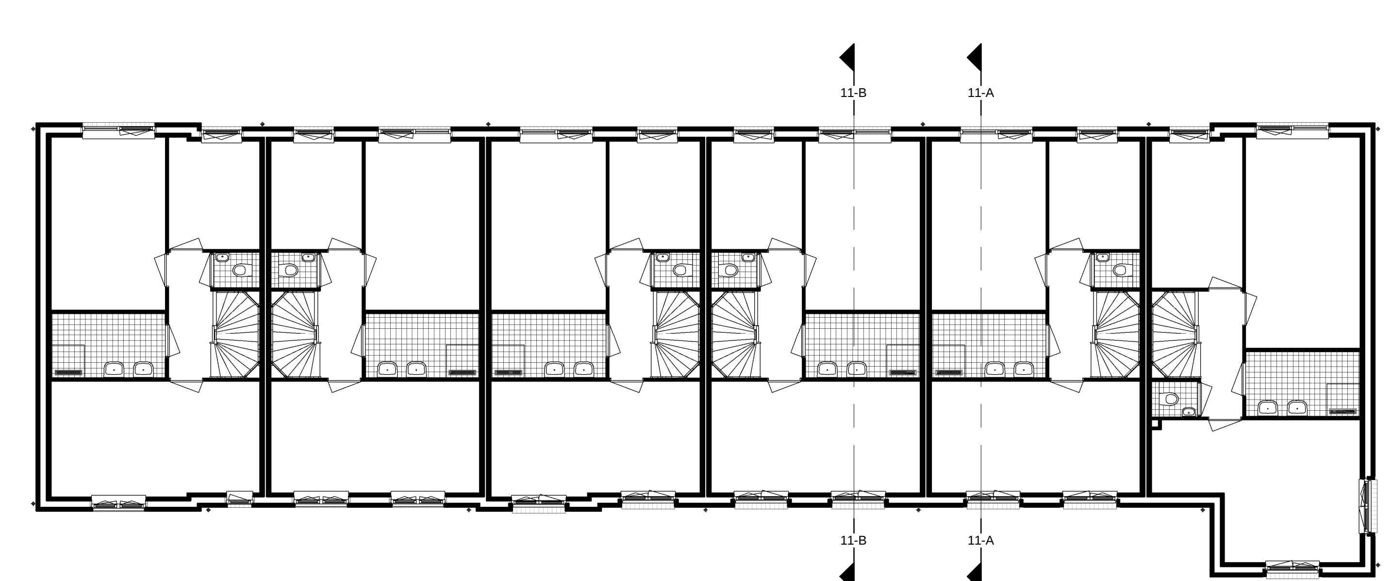
Eerste verdieping
