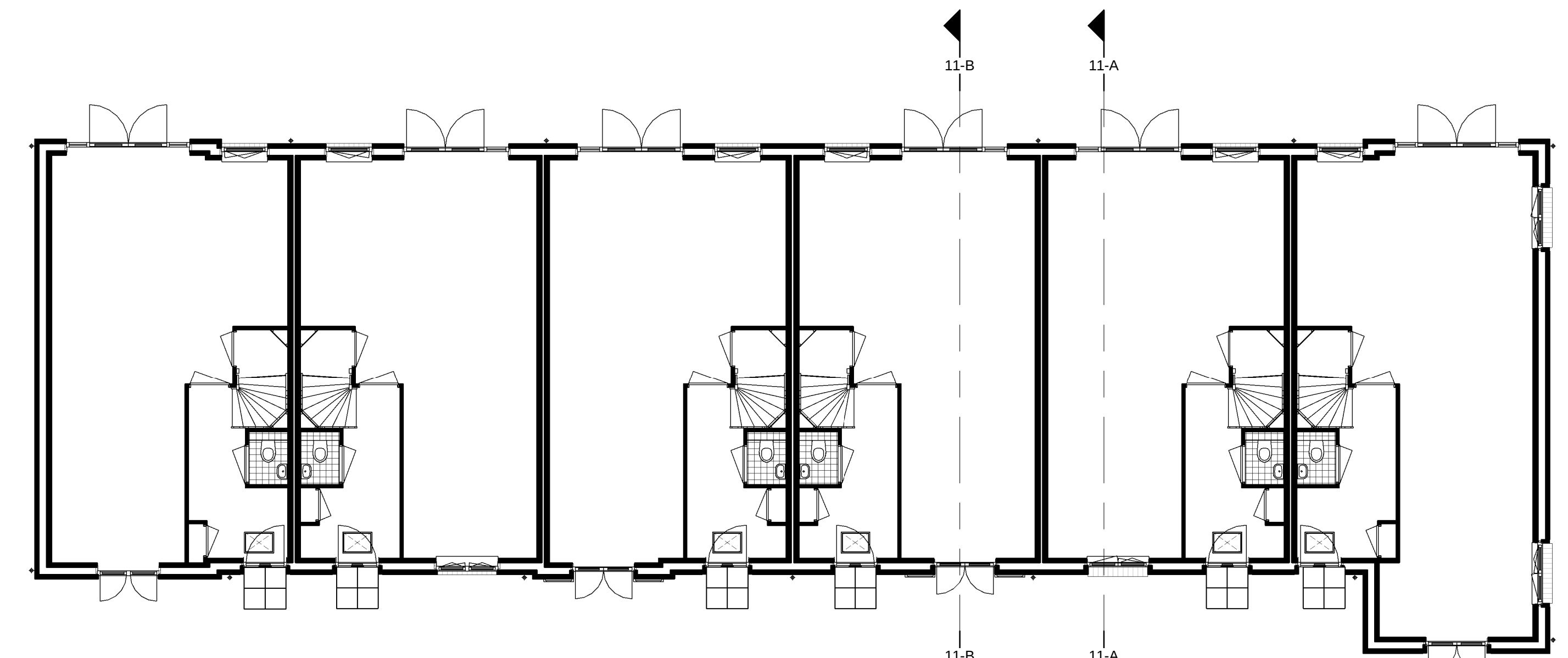
Begane grond
