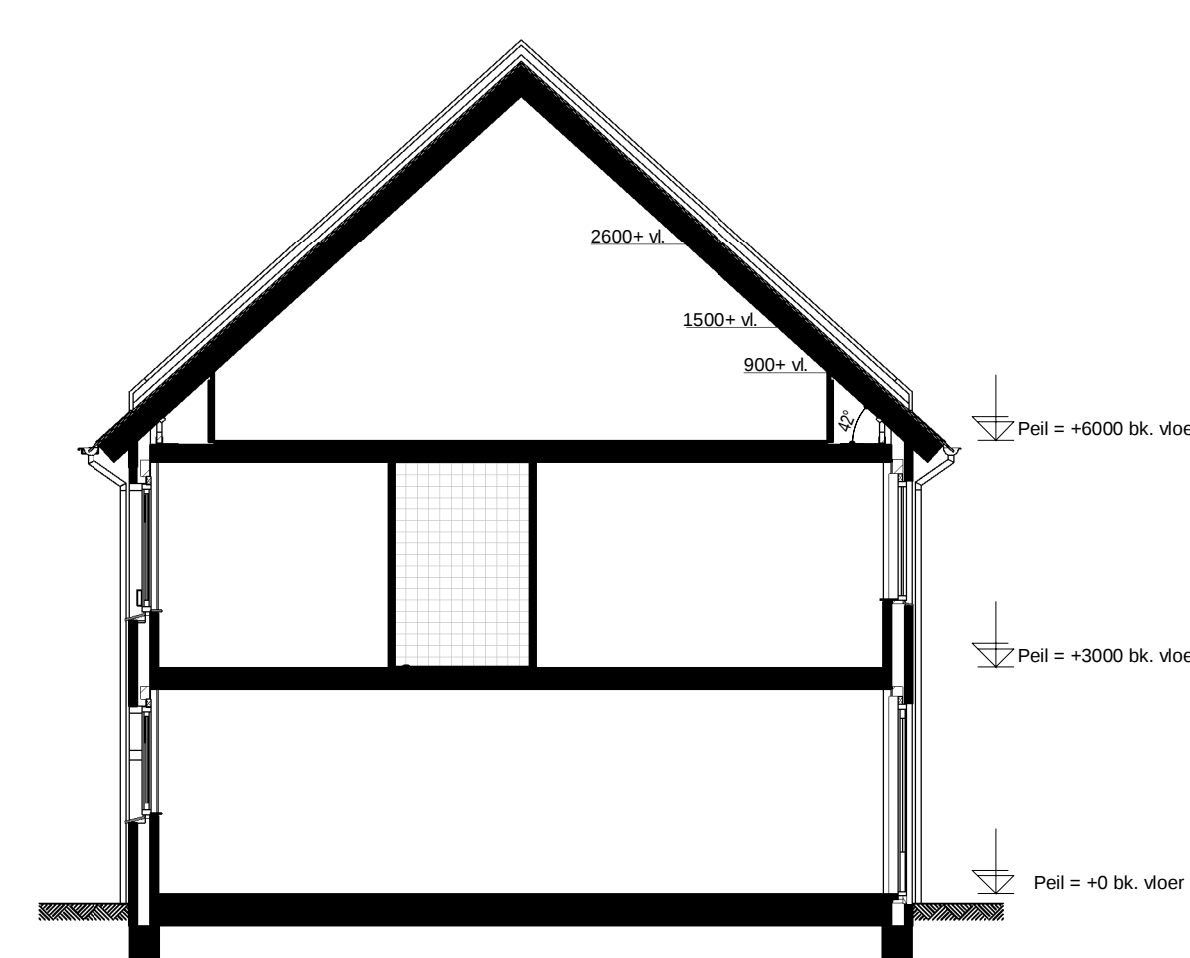
Doorsnede 11-A
