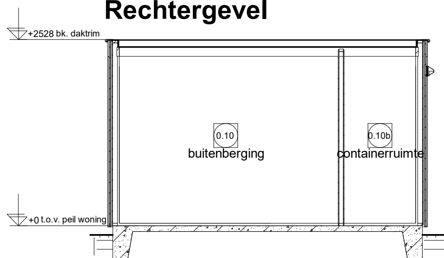
Doorsnede 19.1
