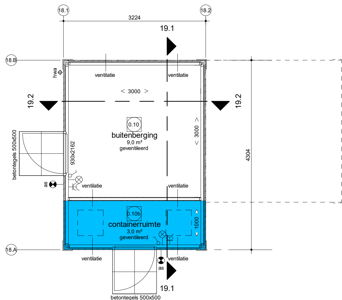
Begane grond
