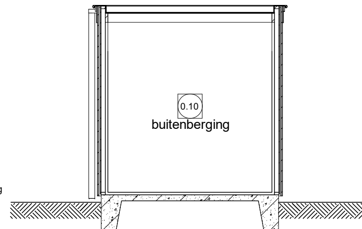
Doorsnede L
