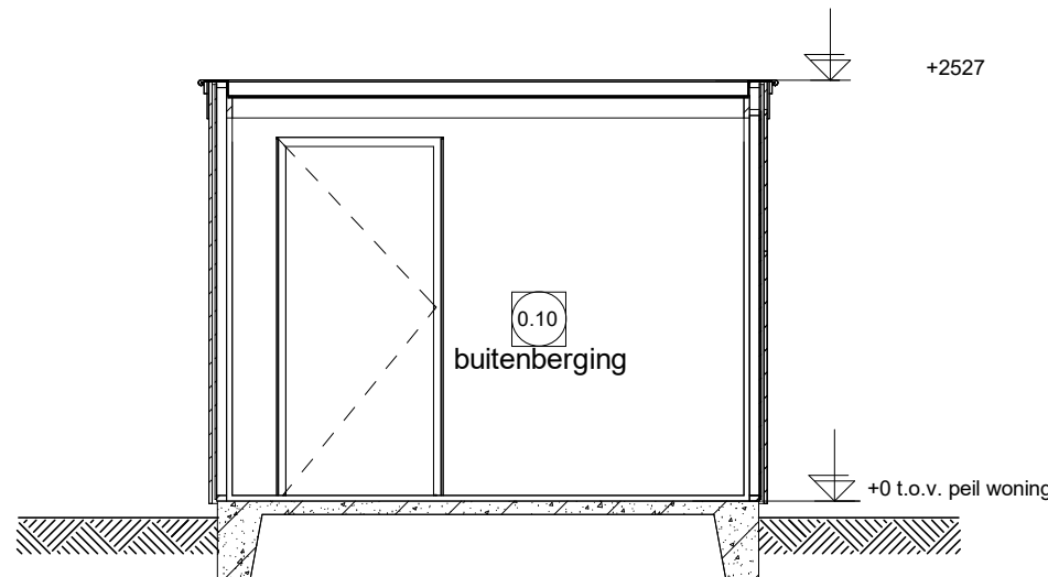
Doorsnede K
