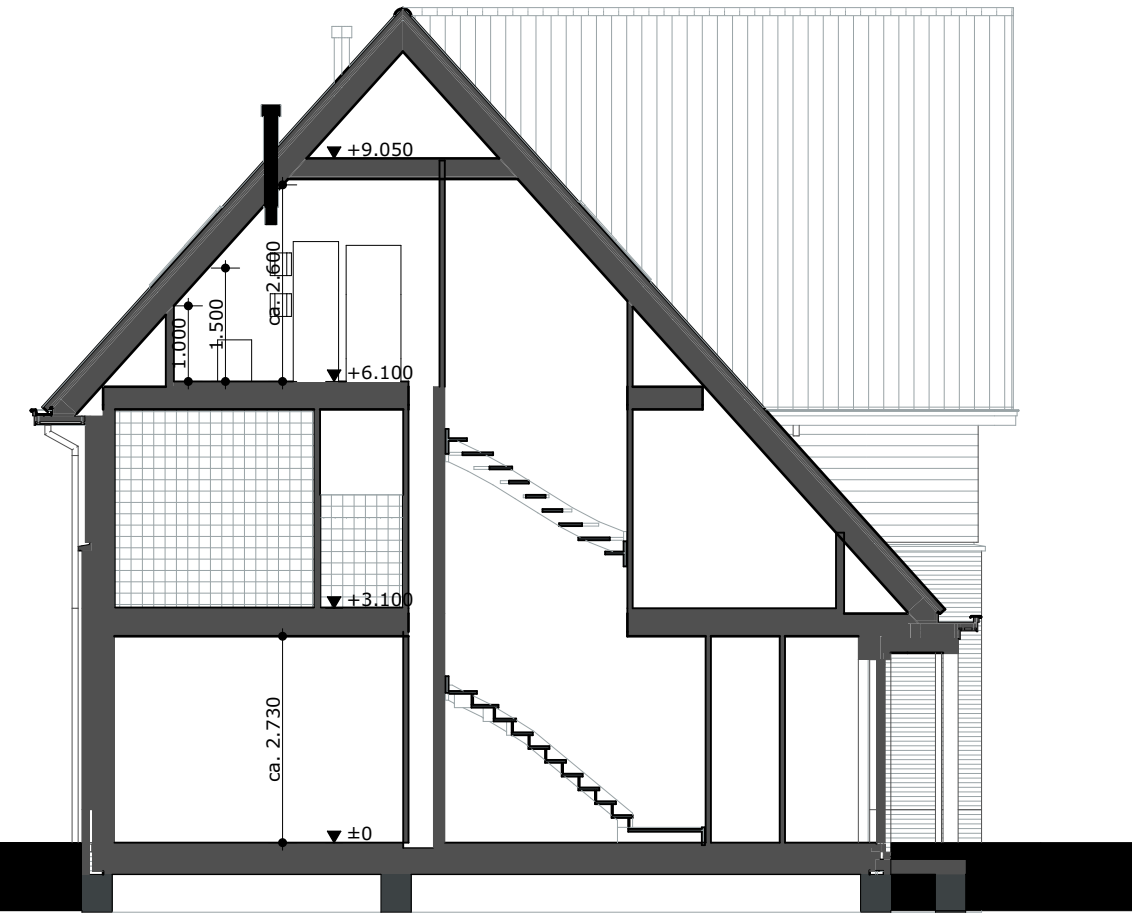
Doorsnede B-B
