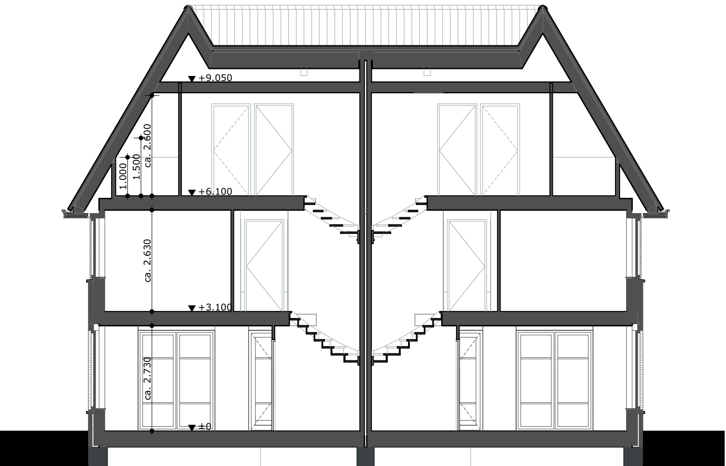
Doorsnede A-A
