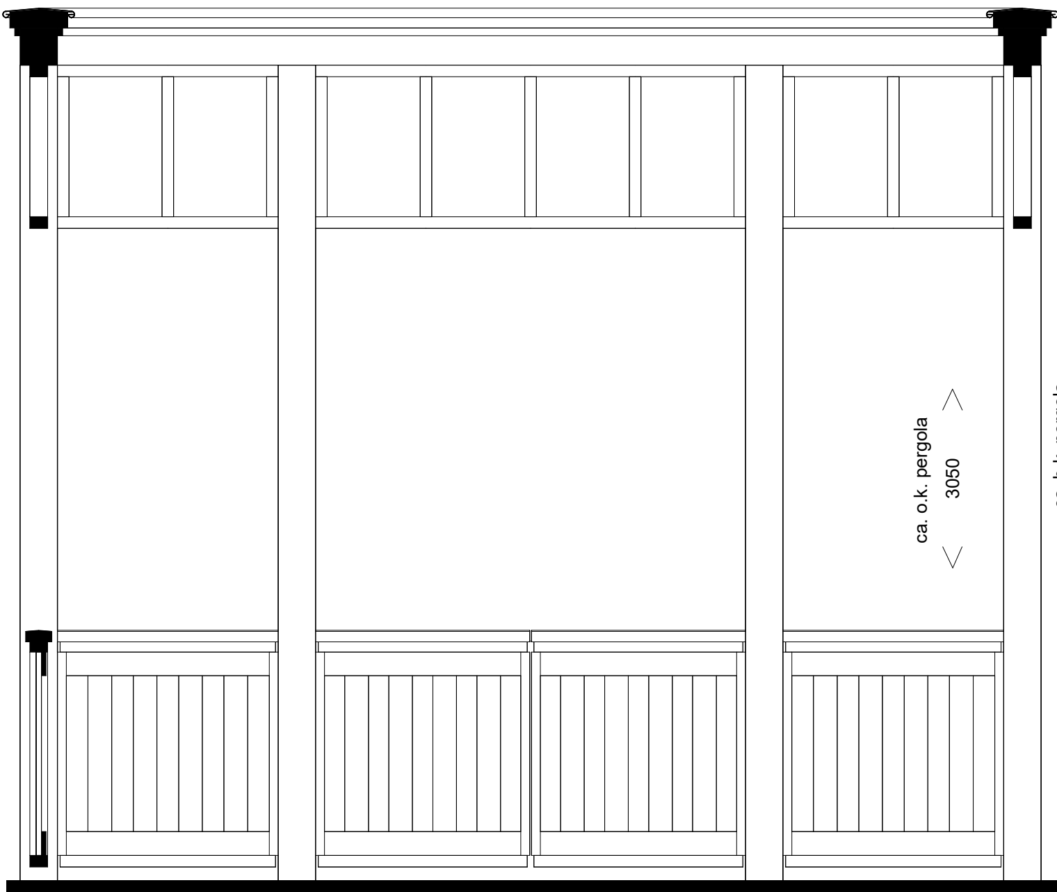
Doorsnede D.PA
