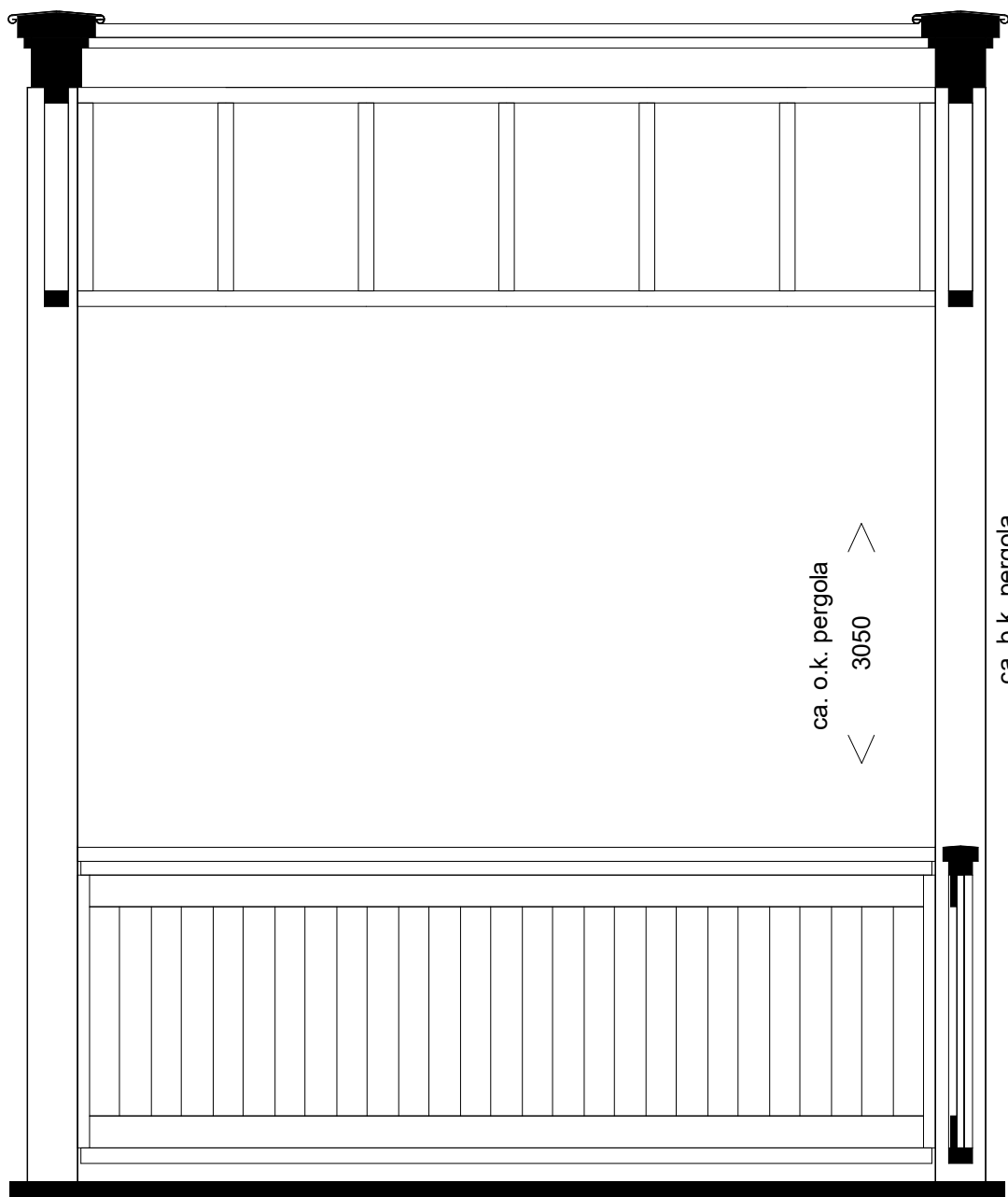
Doorsnede D.PB
