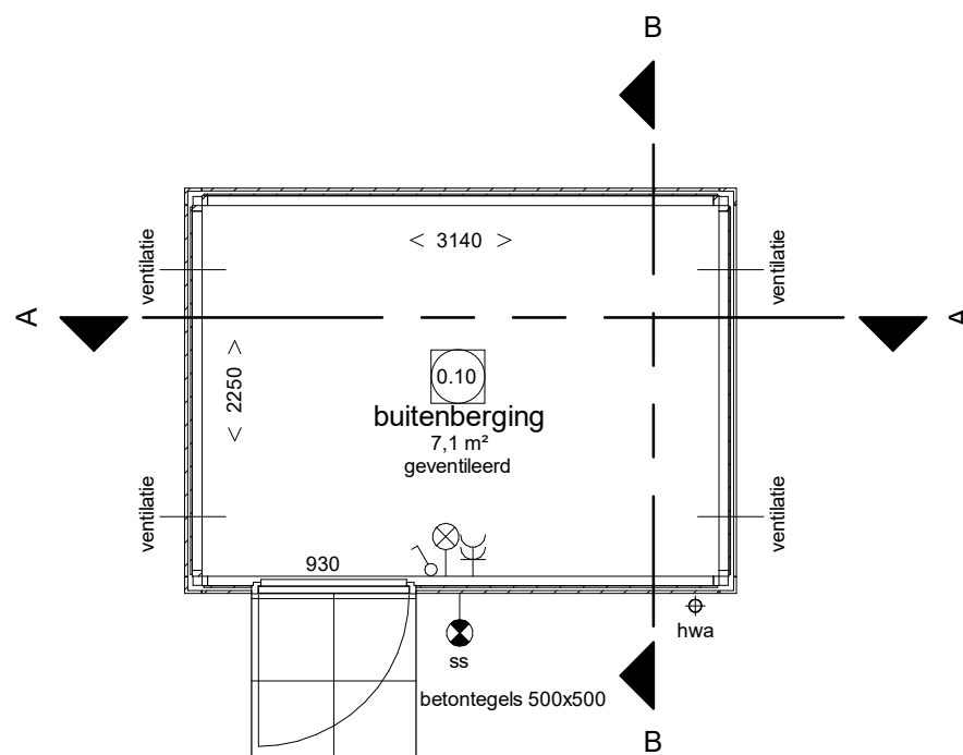
Begane grond
