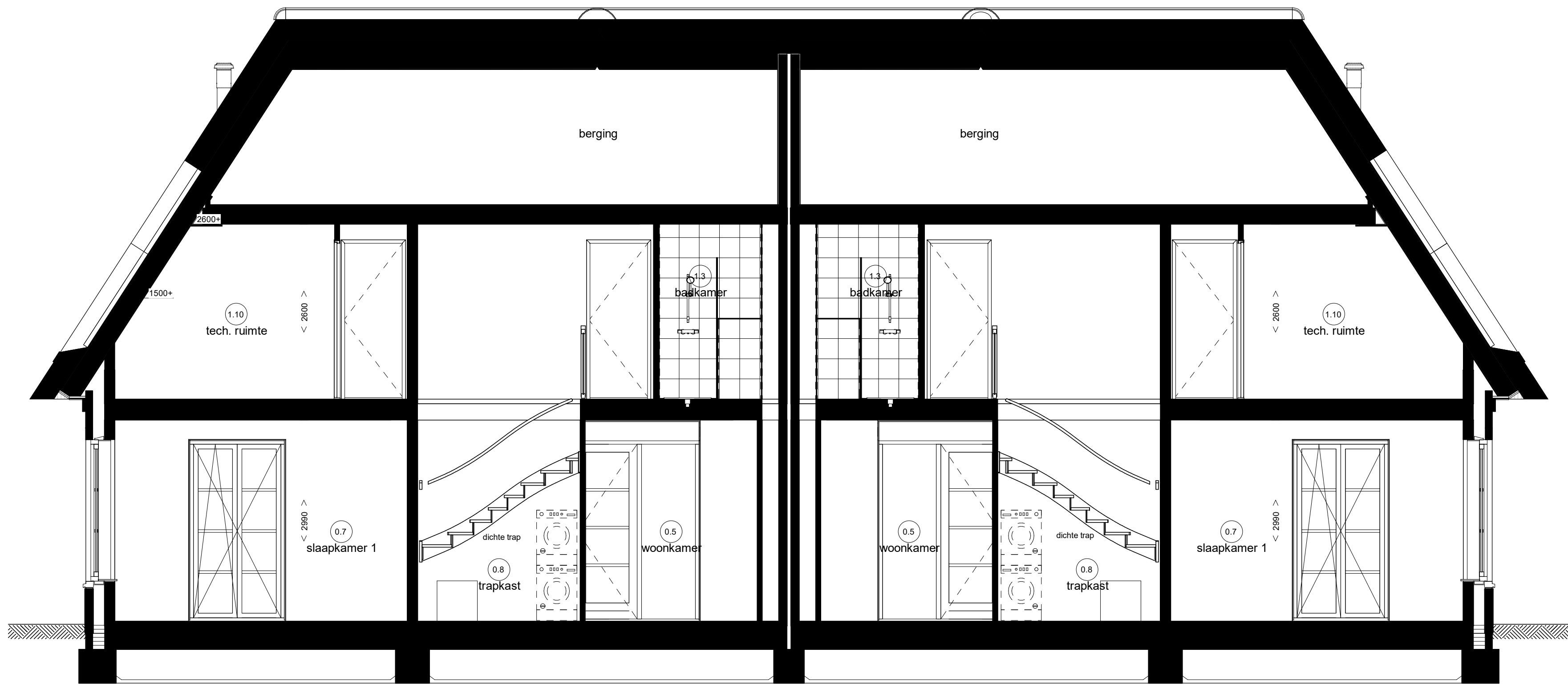
Doorsnede 12.2
