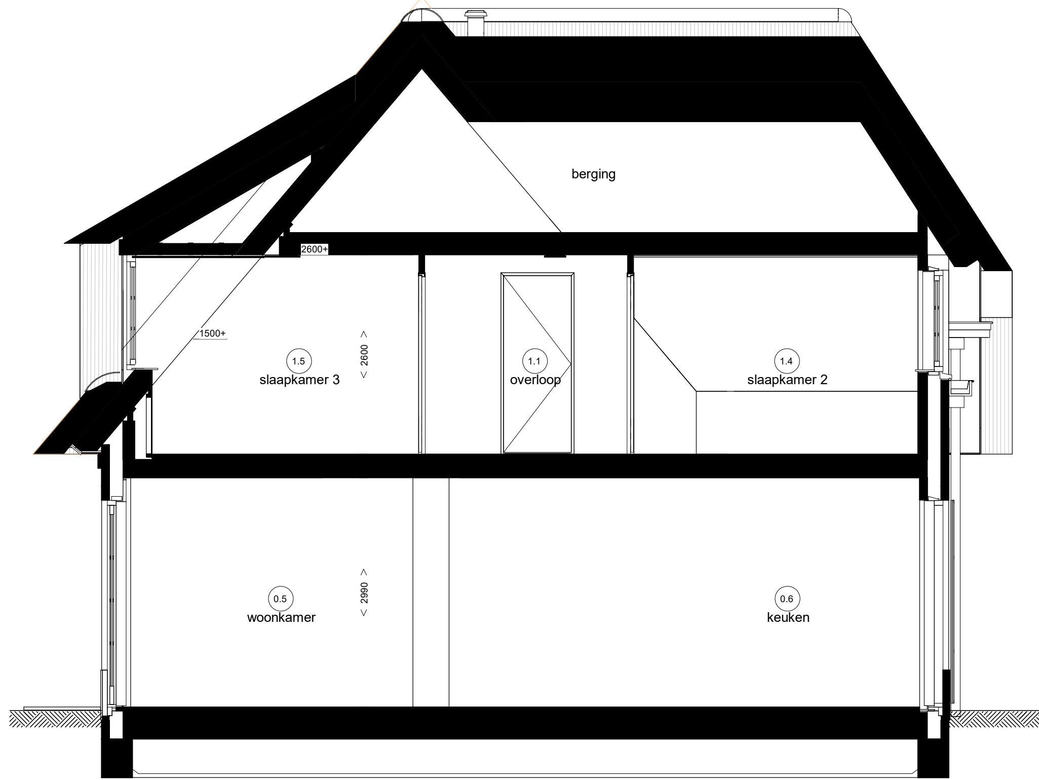
Doorsnede 12.1
