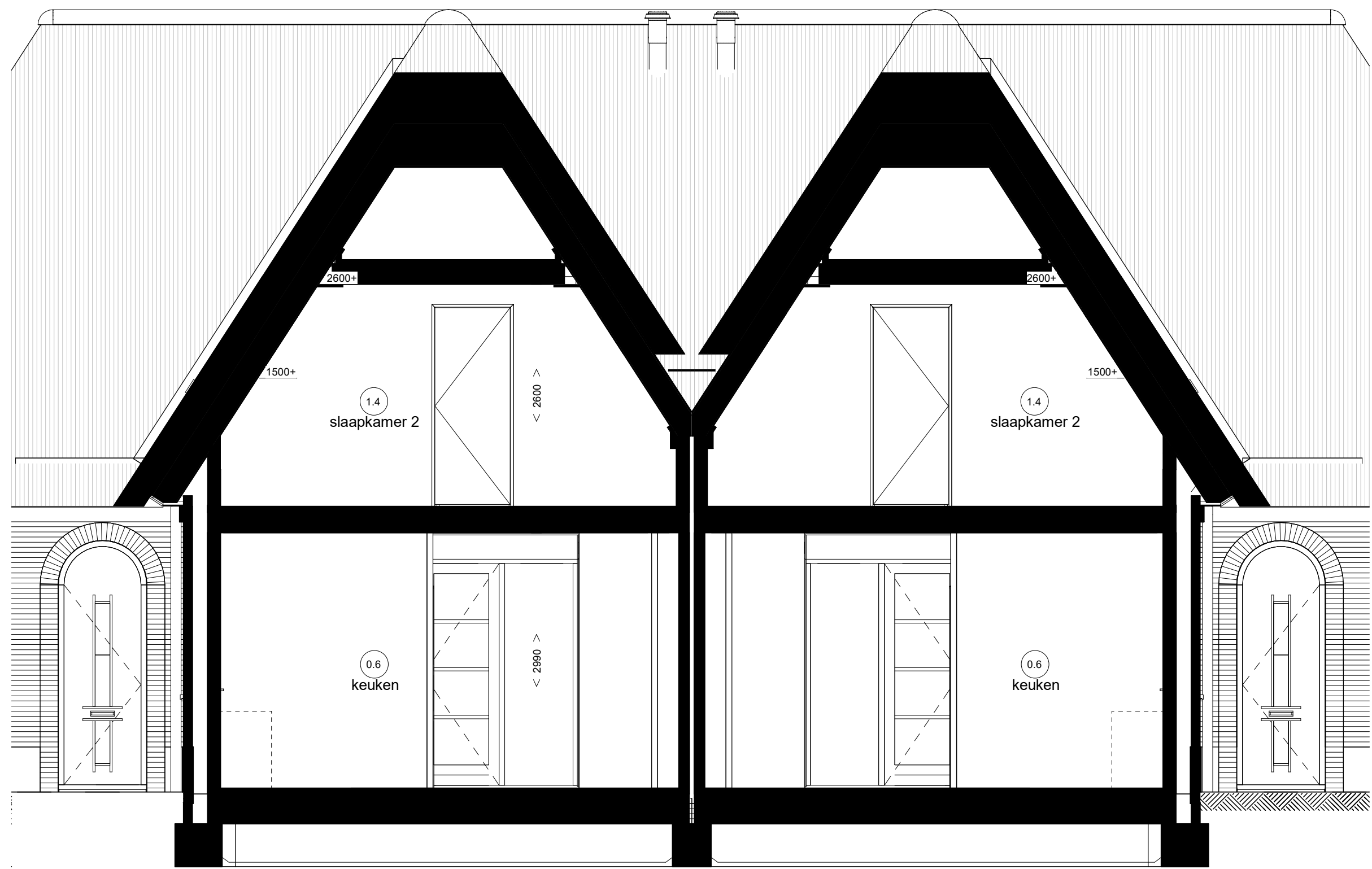
Doorsnede 12.3
