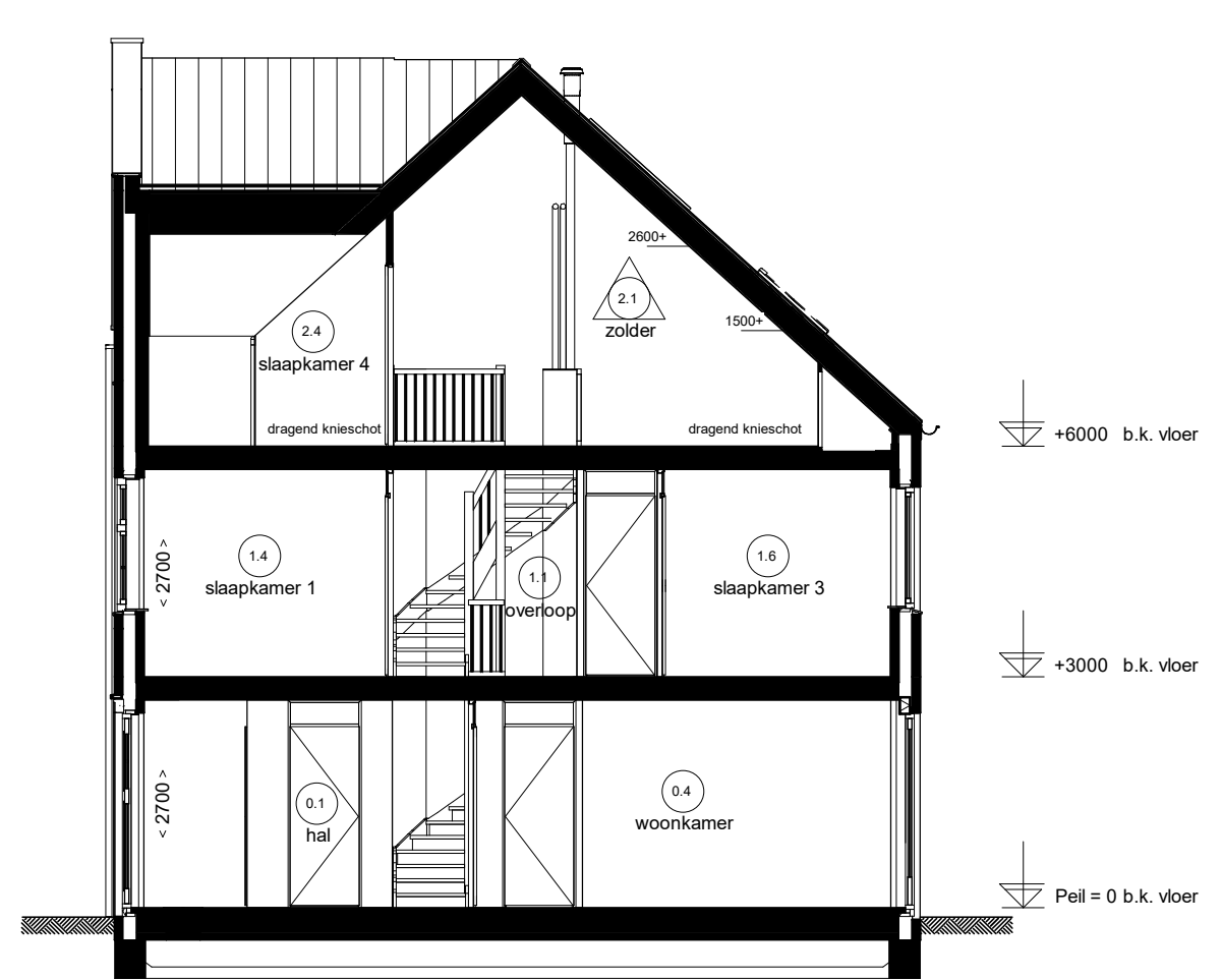
Doorsnede D1.B
