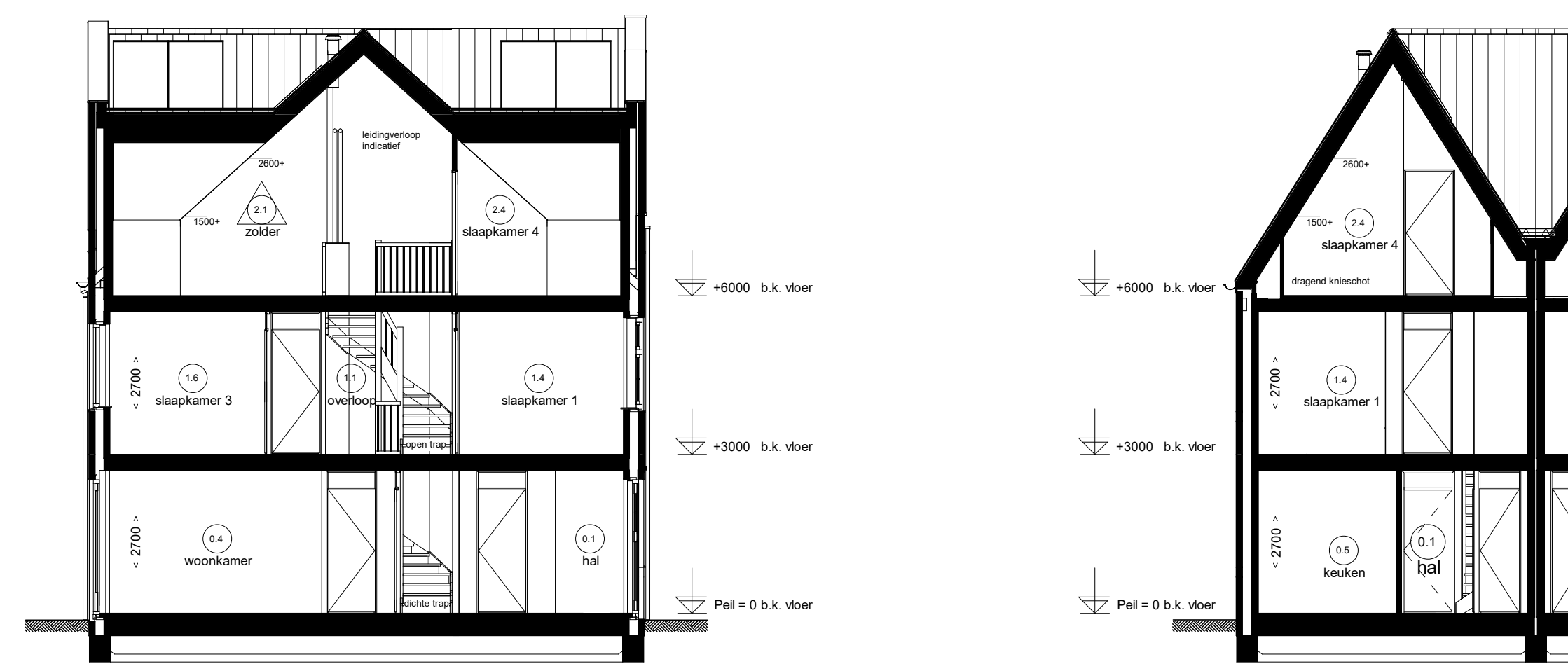
Doorsnede D10.2
