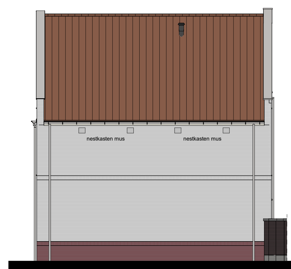
Linkergevel
