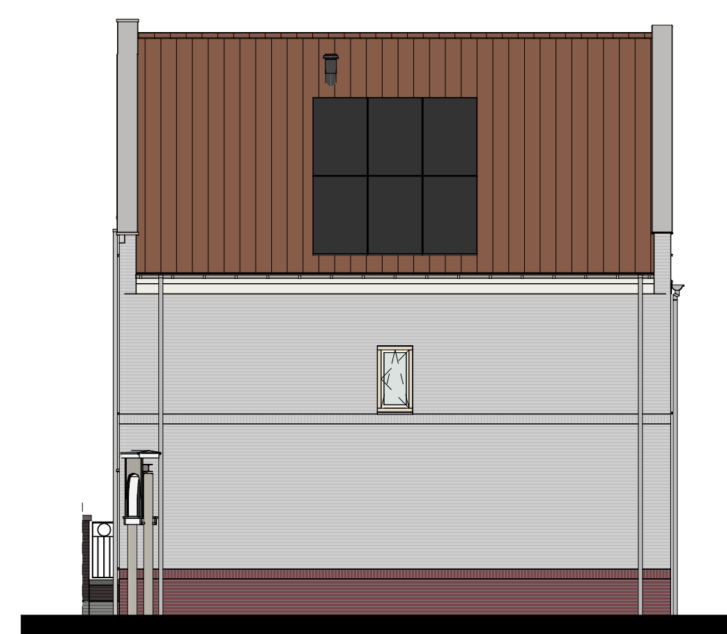
Rechtergevel
