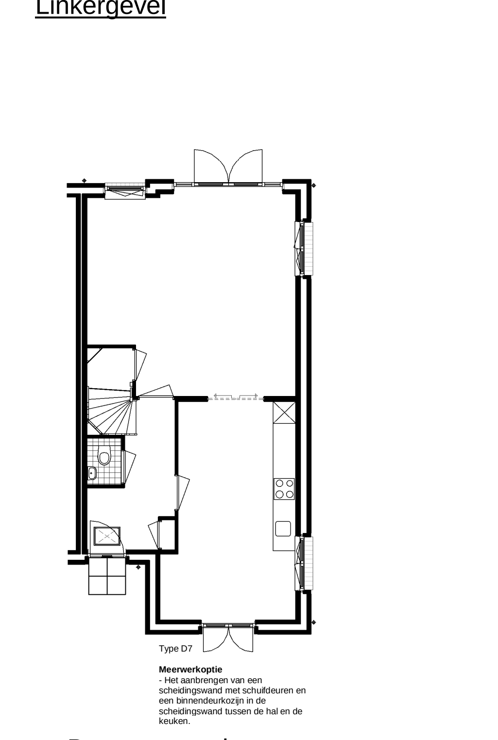
Begane grond
