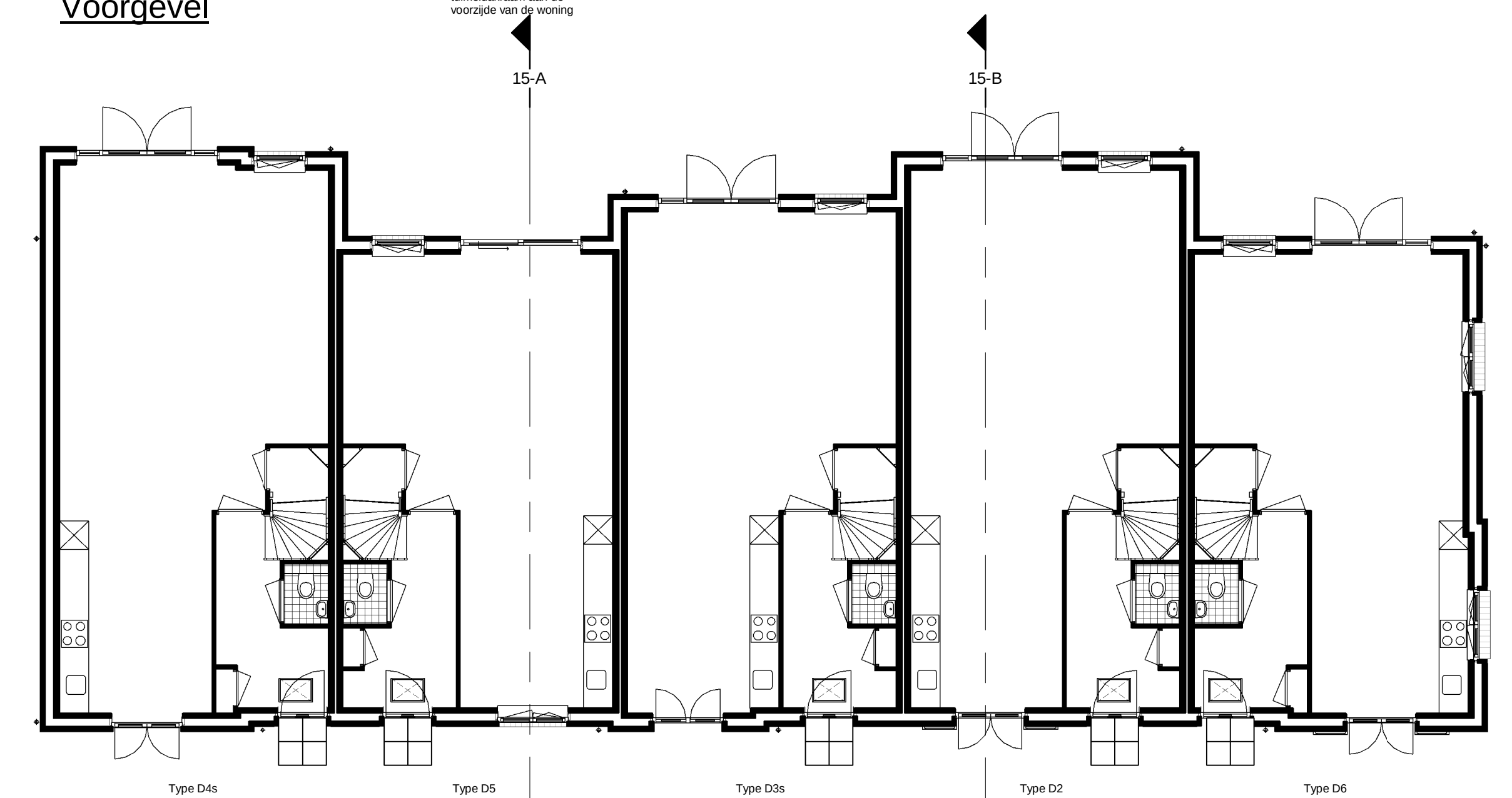
Voorgevel
