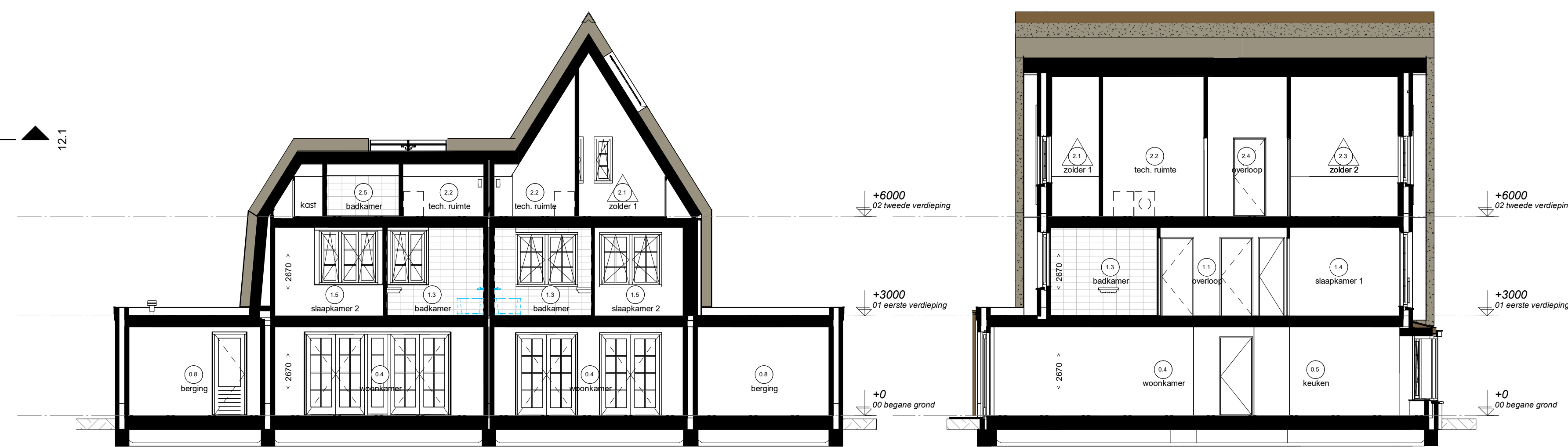
Doorsnede 12.1
