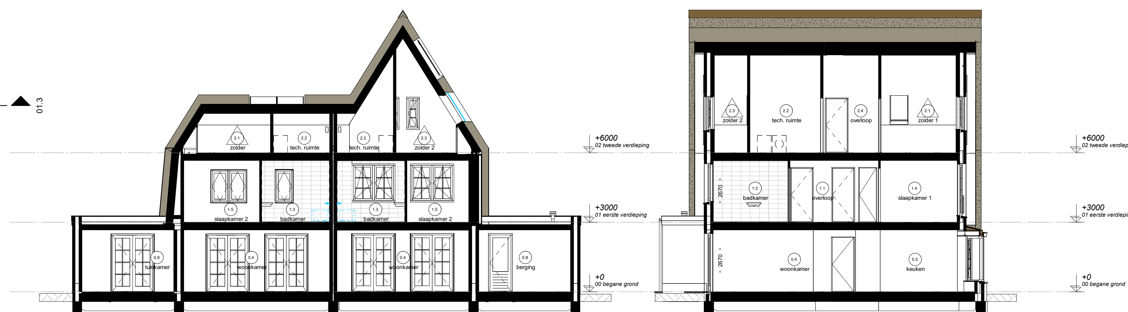
Doorsnede 01.4
