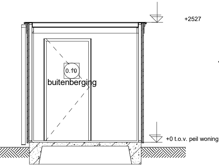
Doorsnede Q
