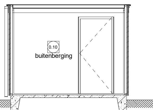
Doorsnede Z
