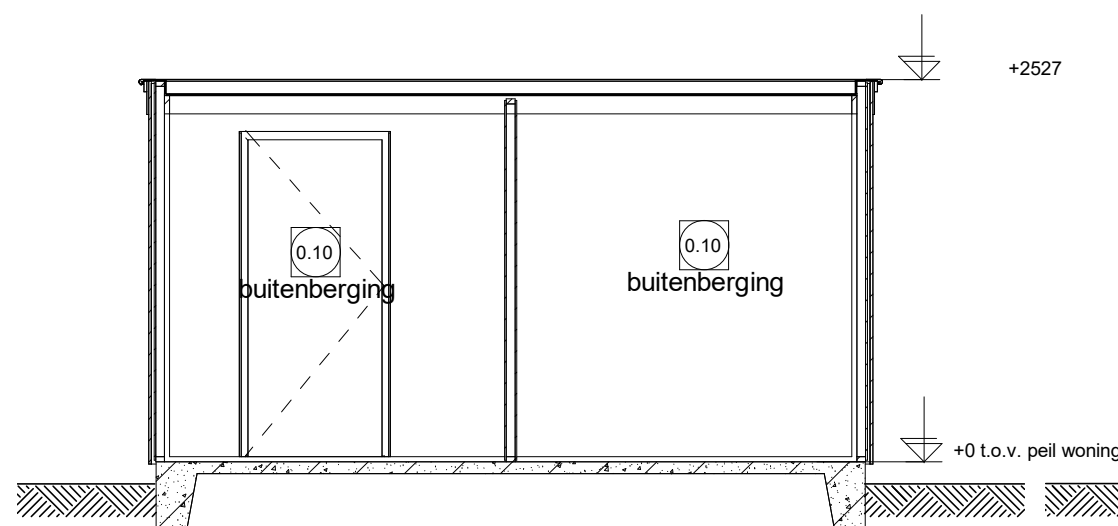
Doorsnede Y
