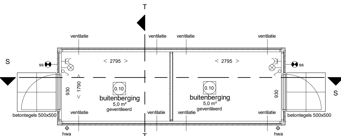
Begane grond
