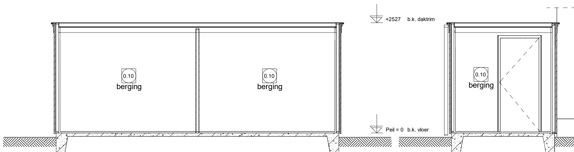
Doorsnede D
