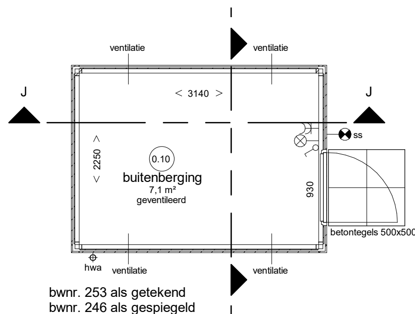
Begane grond
