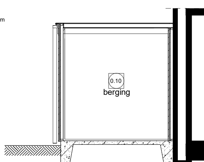
Doorsnede F
