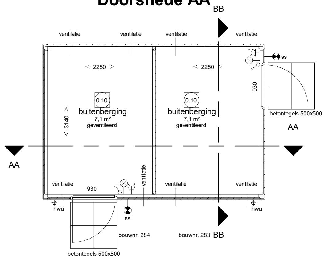
Begane grond
