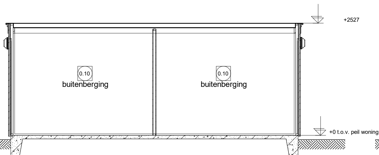
Doorsnede U
