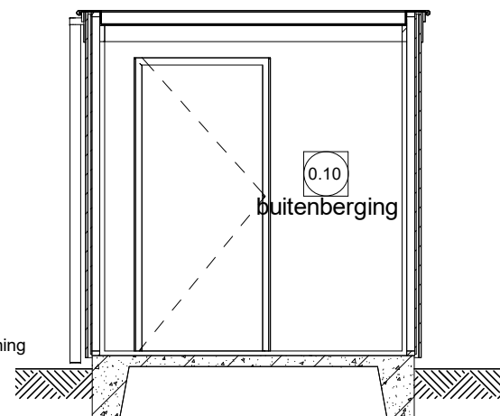
Doorsnede V
