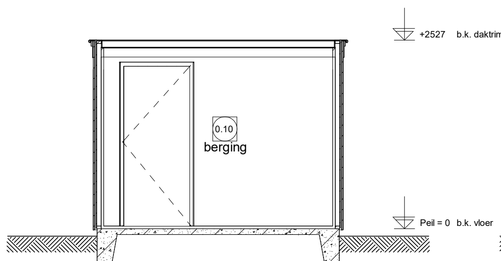
Doorsnede G
