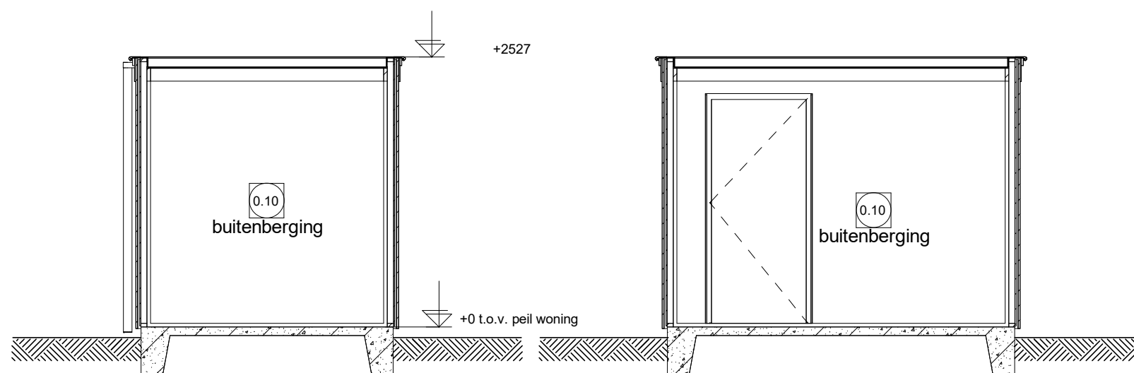
Doorsnede G
