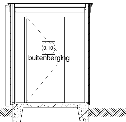
Doorsnede T
