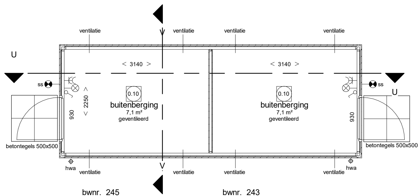
Begane grond
