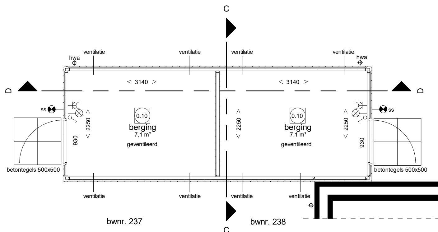
Begane grond
