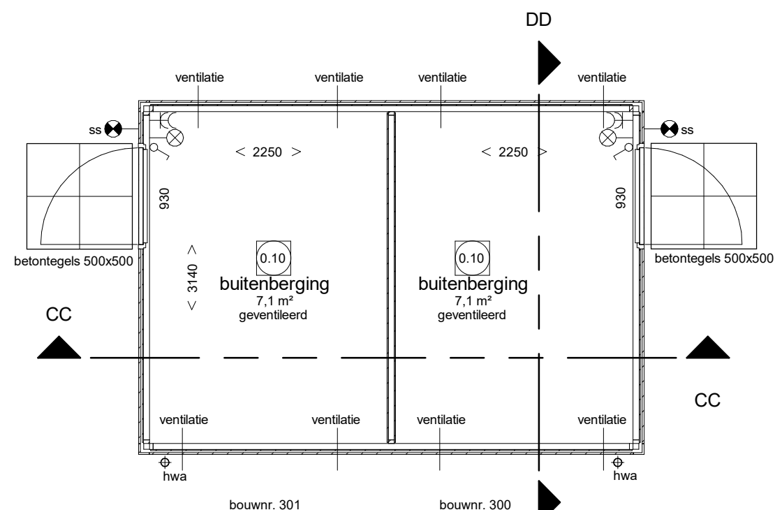
Begane grond
