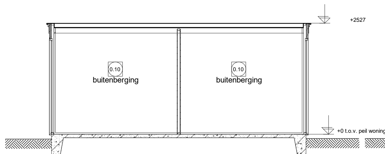
Doorsnede S
