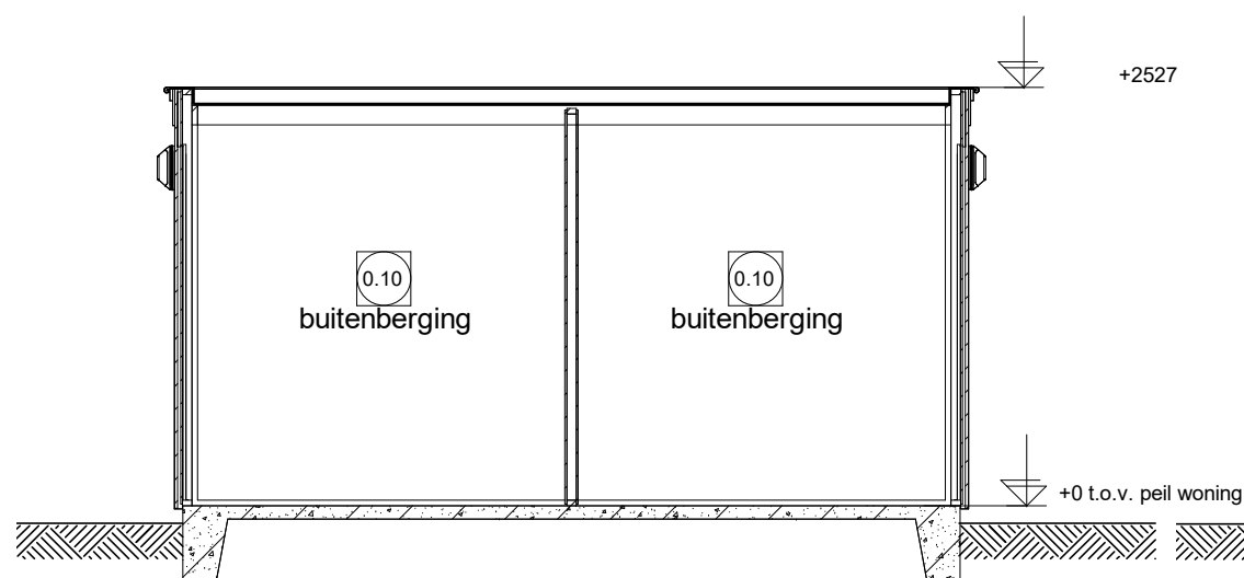
Doorsnede CC
