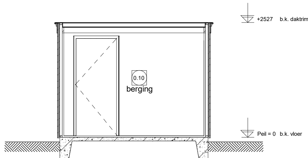
Doorsnede E
