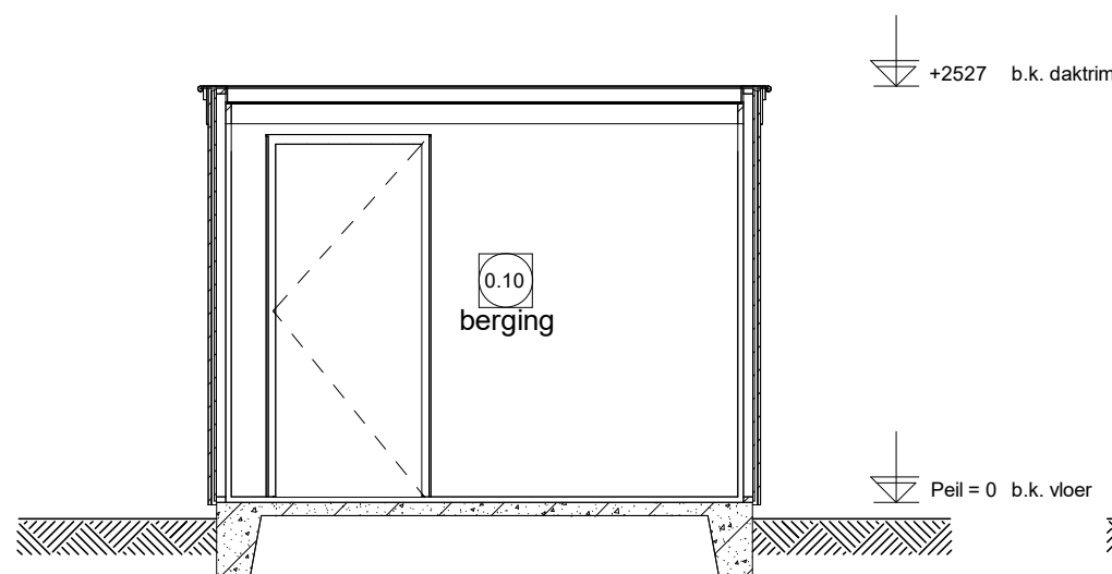
Doorsnede I
