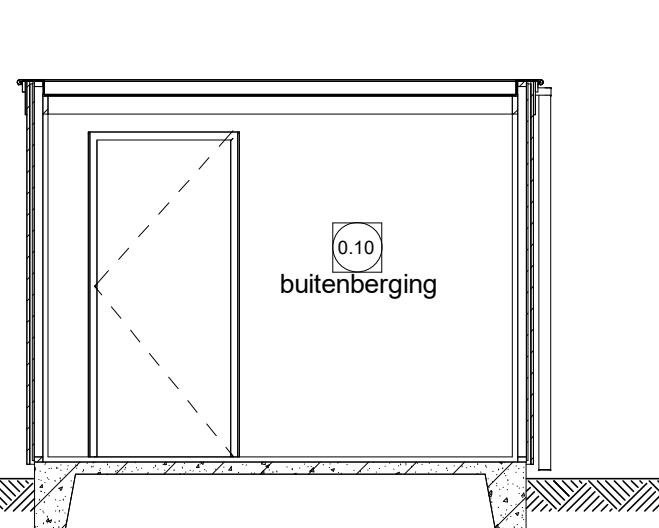
Doorsnede DD
