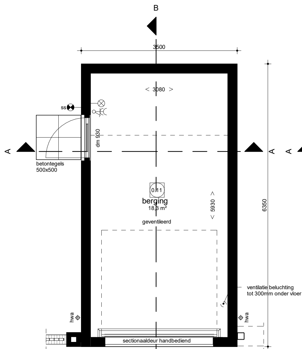
Begane grond
