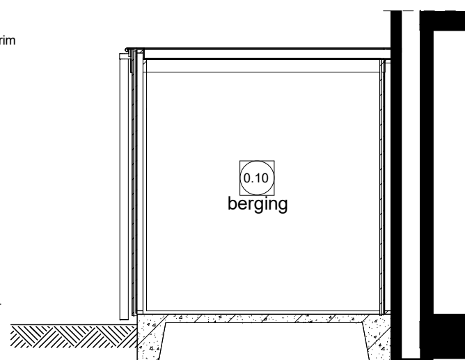
Doorsnede J
