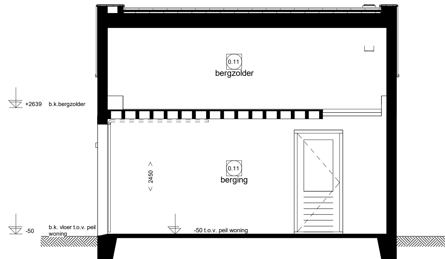
Doorsnede B
