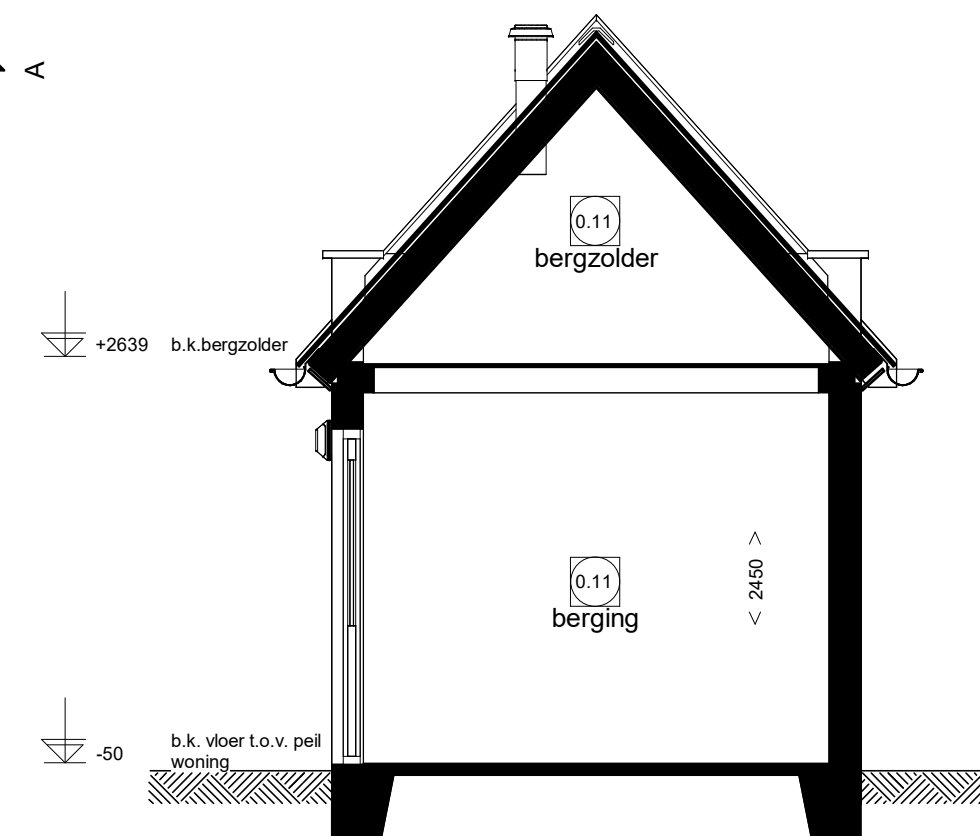
Doorsnede A
