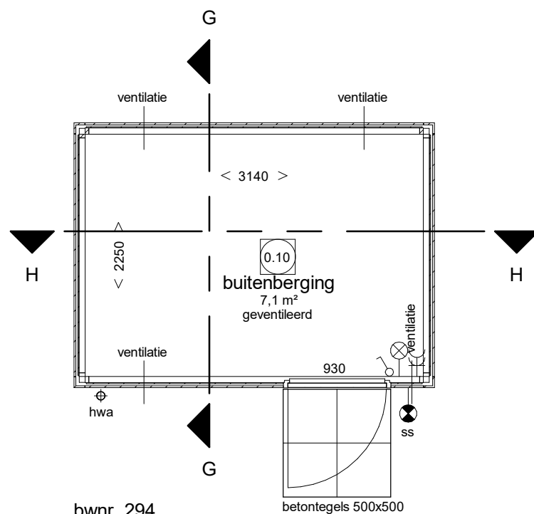
Begane grond
