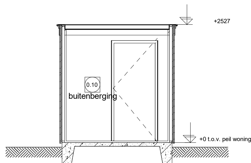
Doorsnede I
