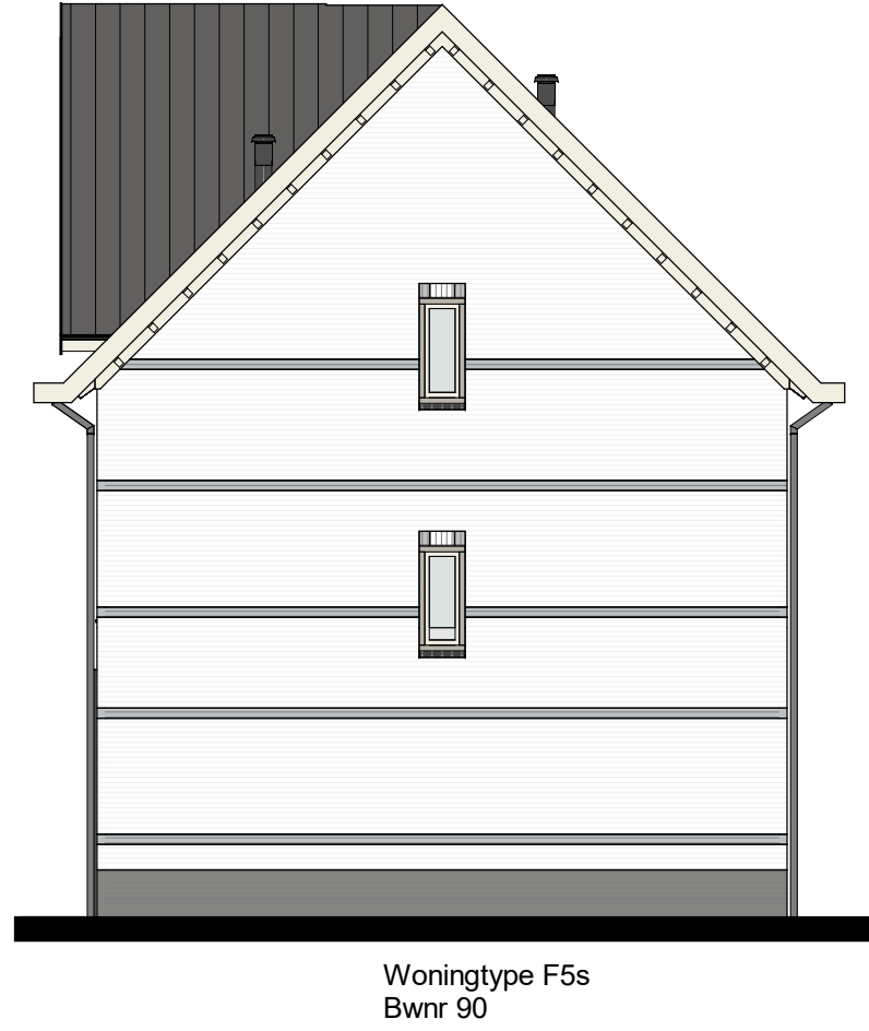
Rechtergevel
