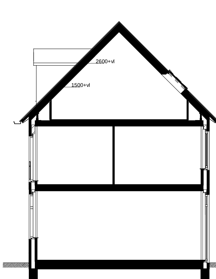
Doorsnede 18-A
