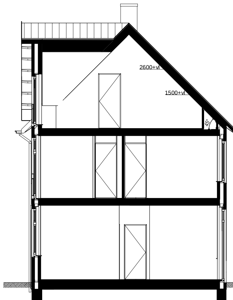
Doorsnede 18-B
