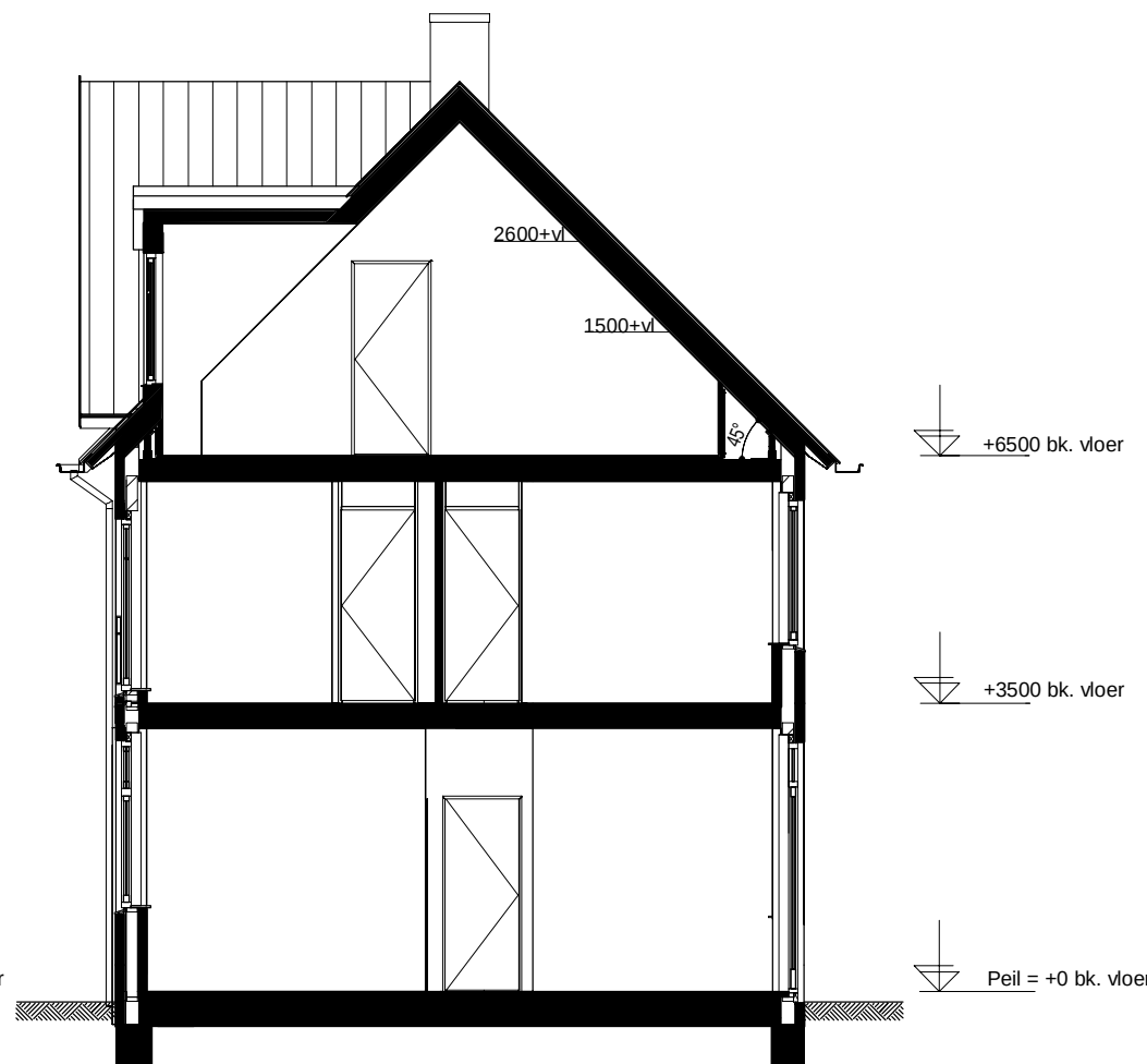
Doorsnede 18-C
