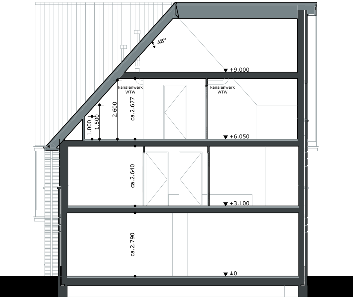
Doorsnede B-B
