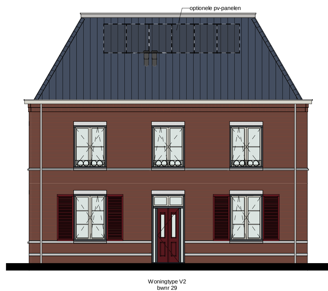
Voorgevel
