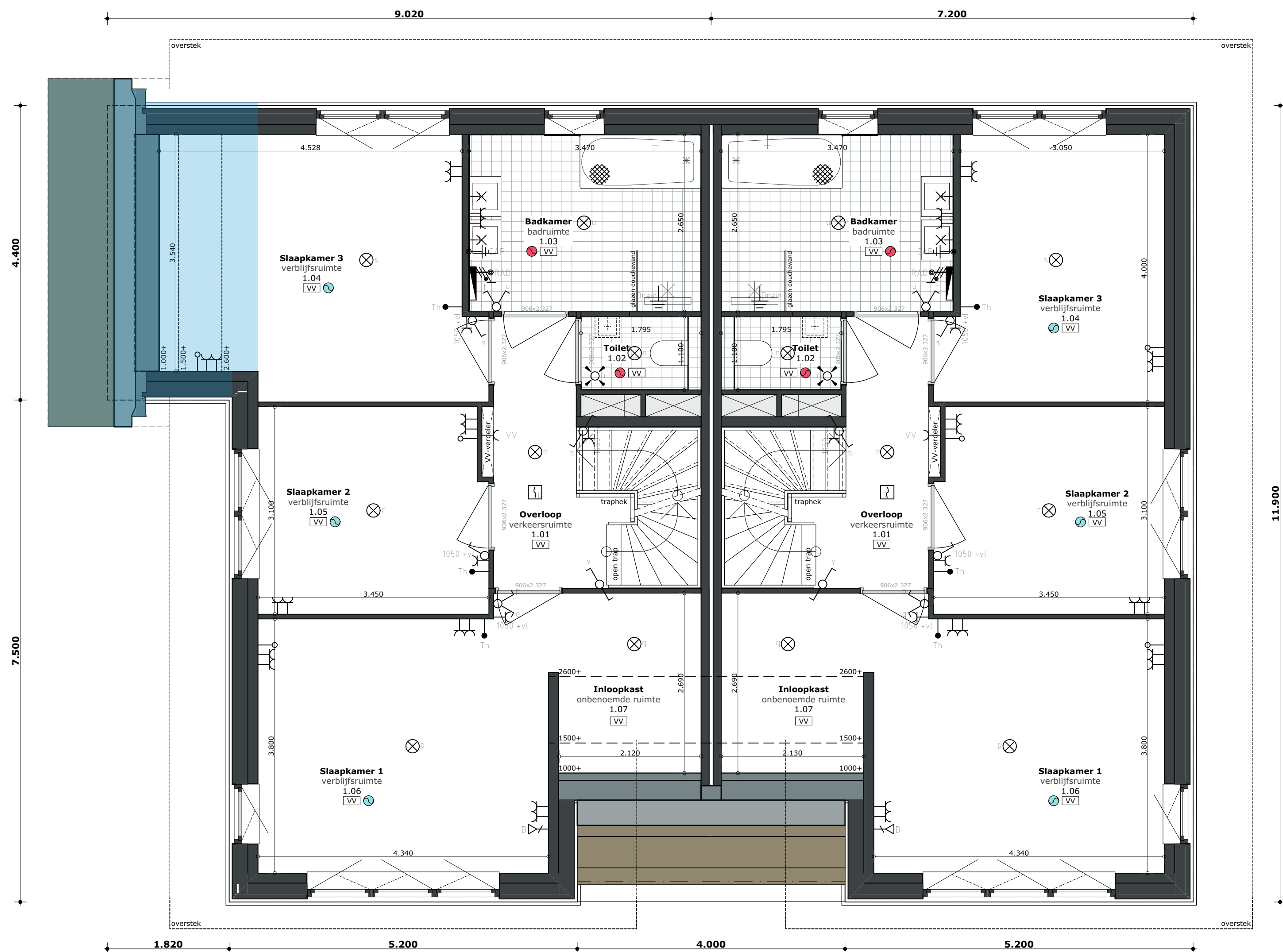
Type QRs A.08 - Uitbouw zijgevel bijkeuken en slaapkamer 3
