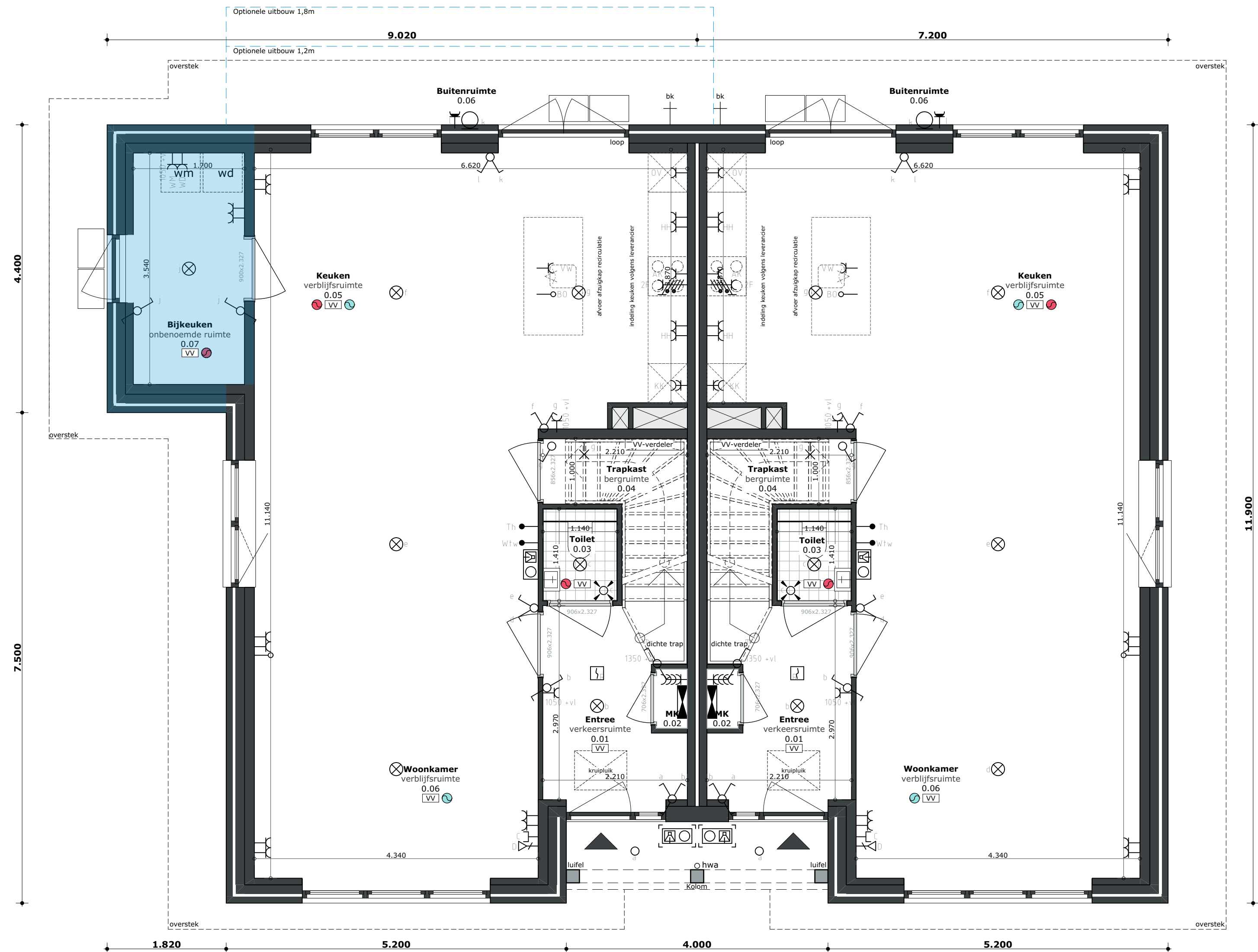
Type QRs A.08a - Uitbouw bijkeuken en slaapkamer 3
