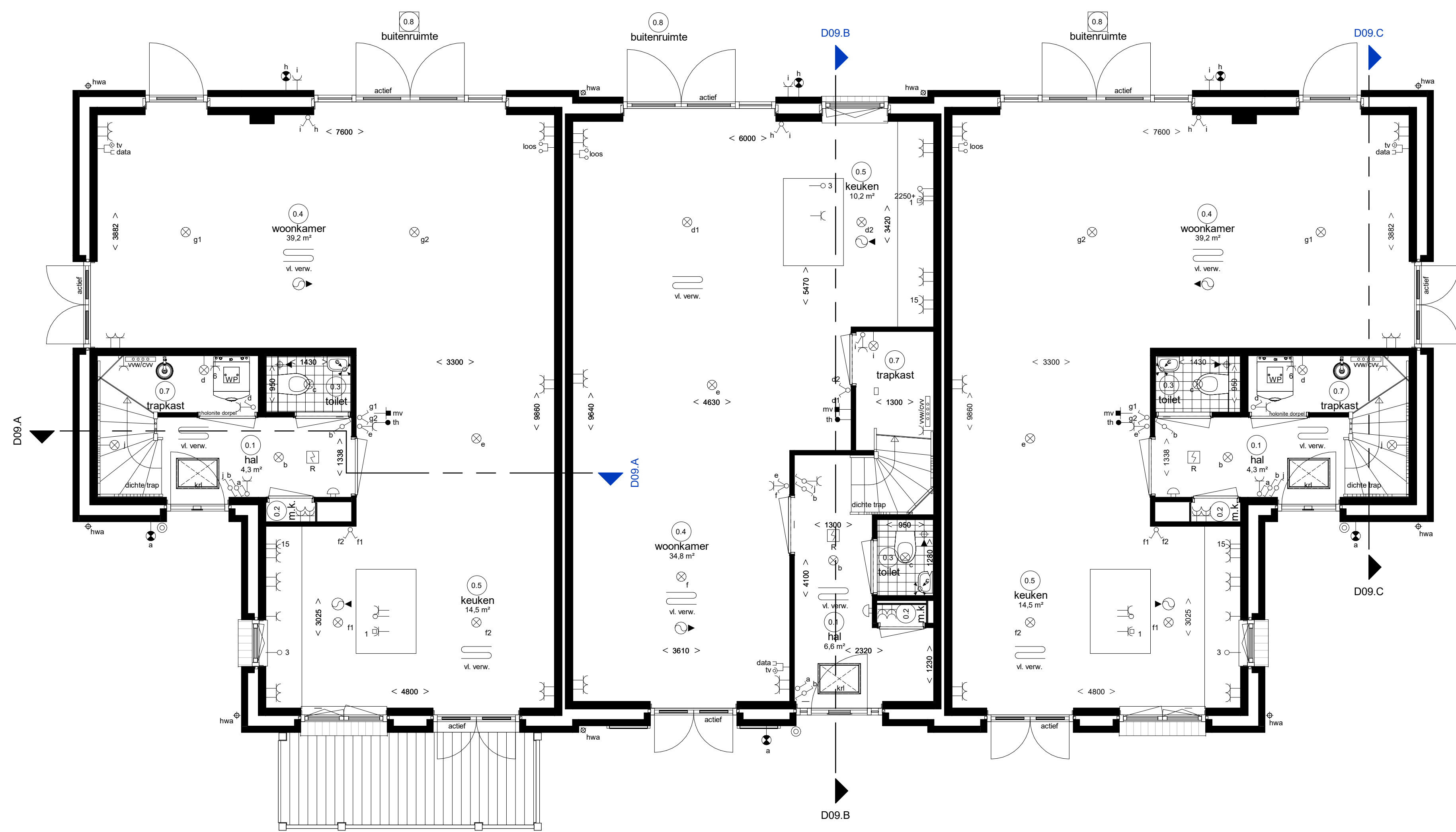
Begane grond
