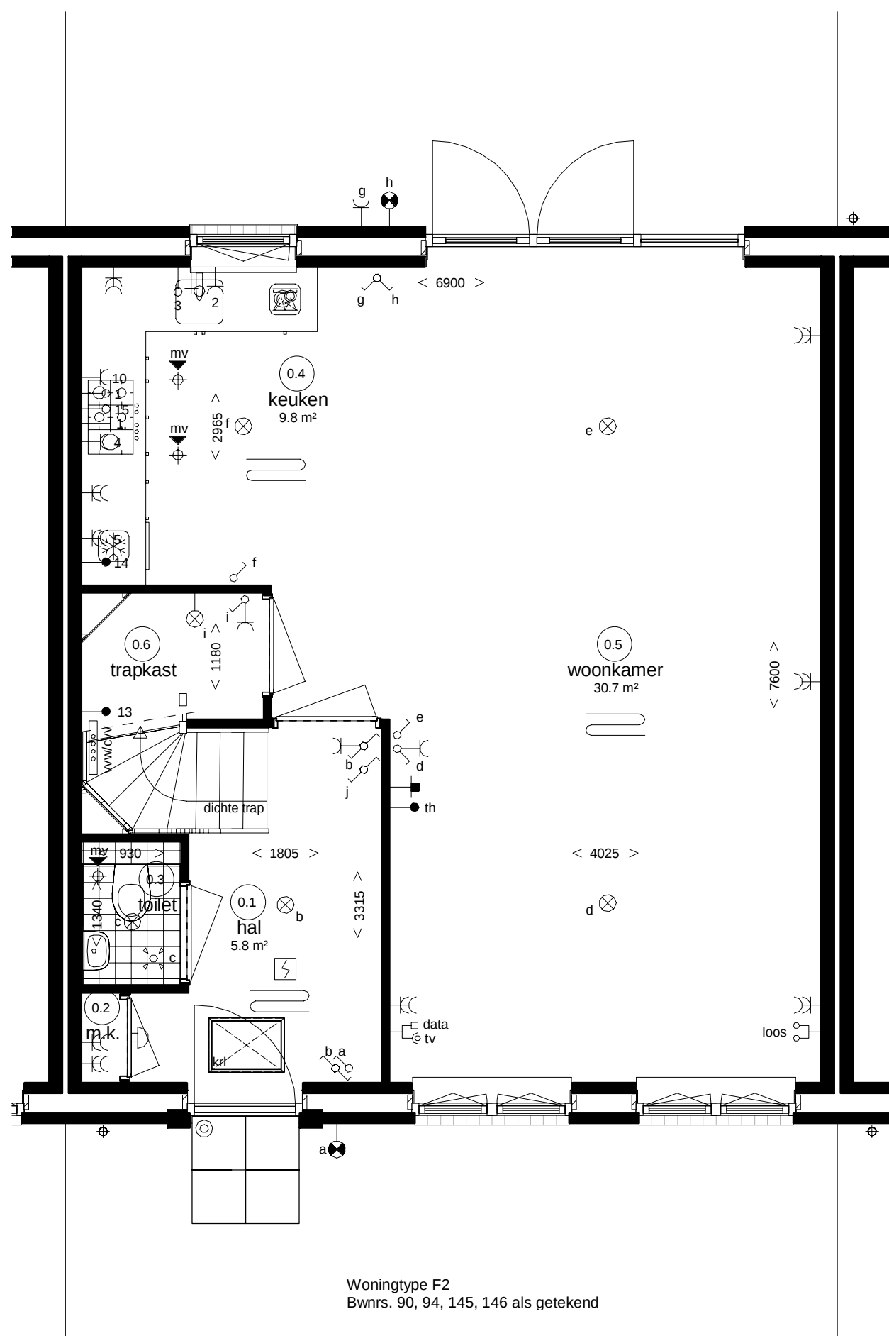
Begane grond
