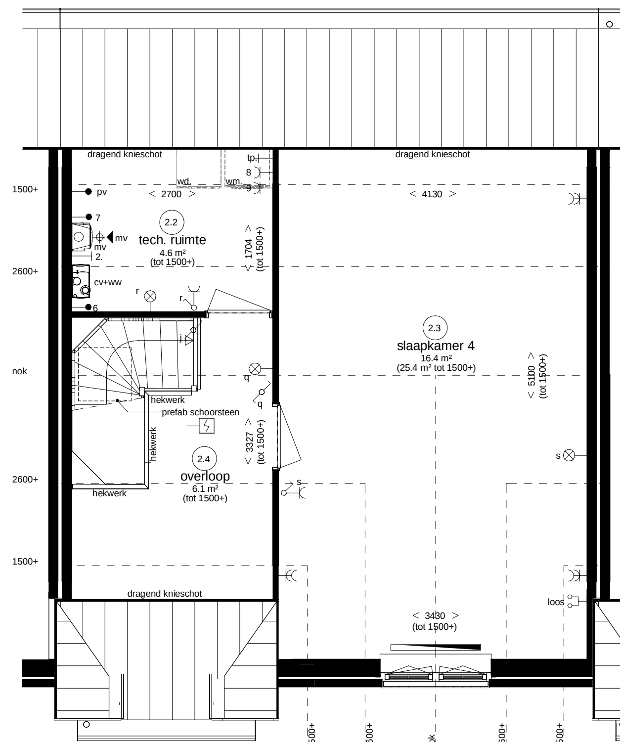
Tweede verdieping
