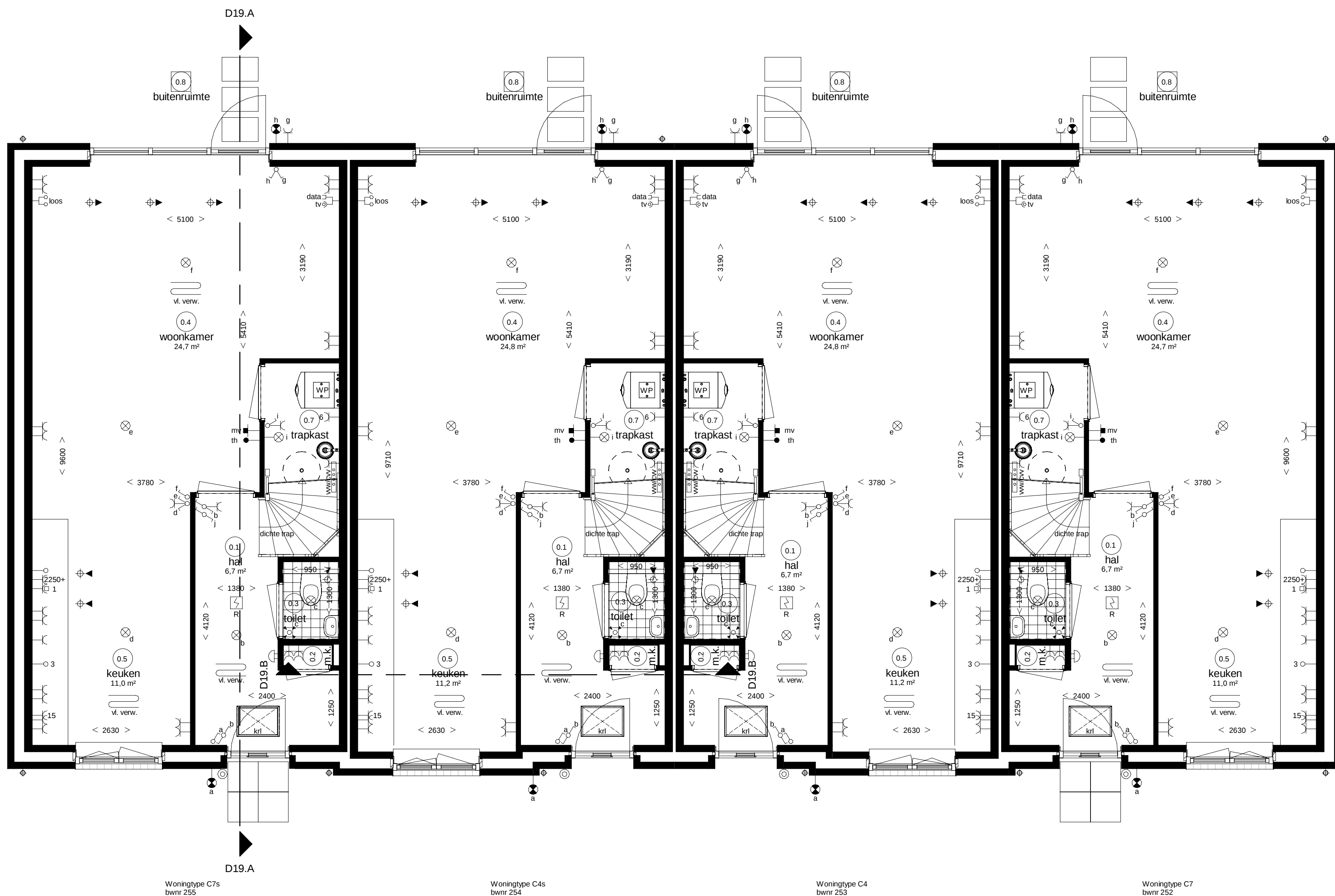
Begane grond
