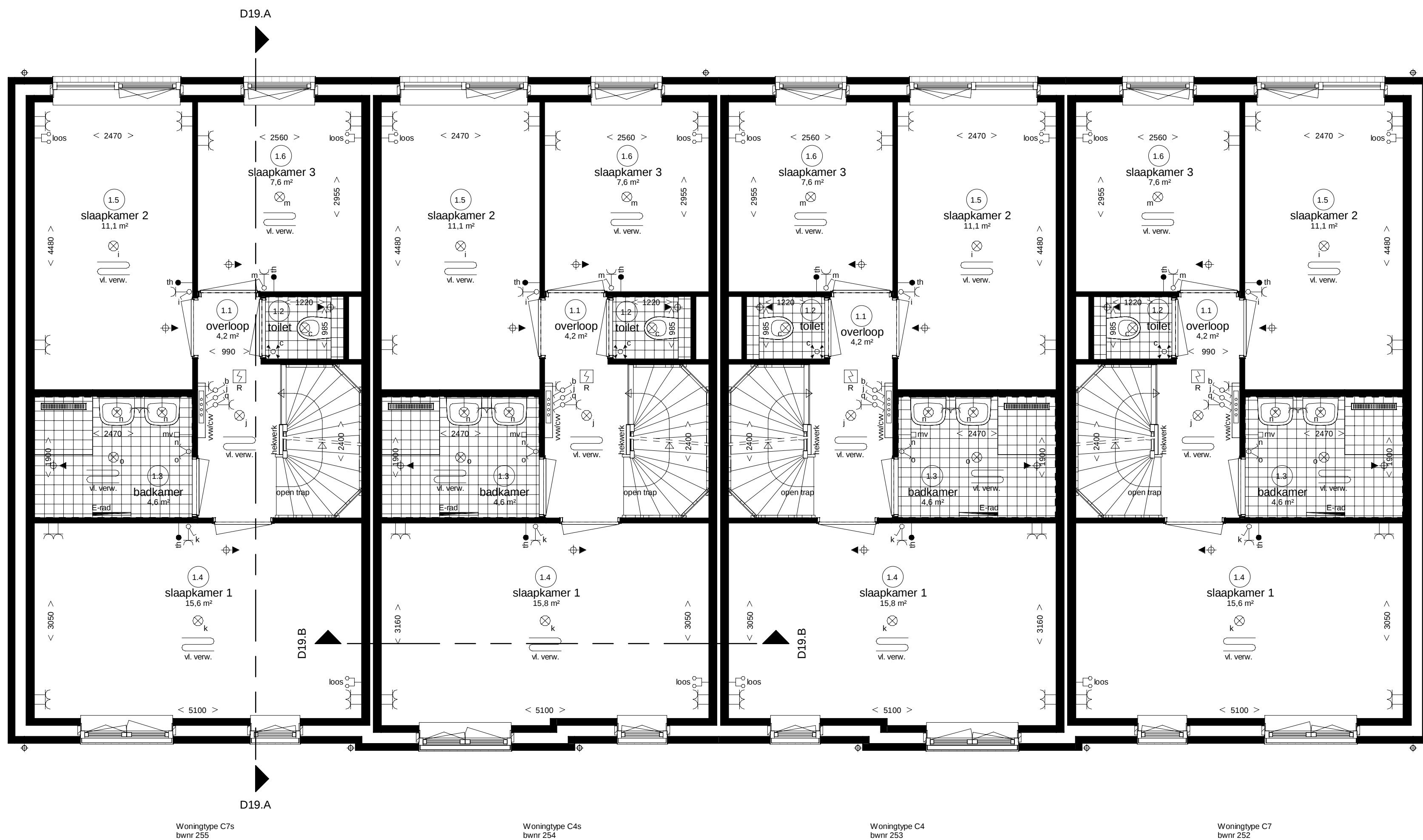
Eerste verdieping
