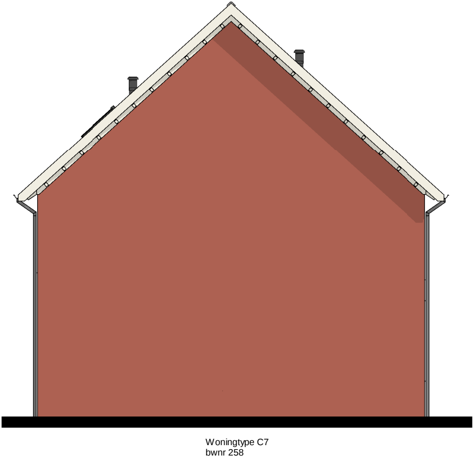
Linkergevel
