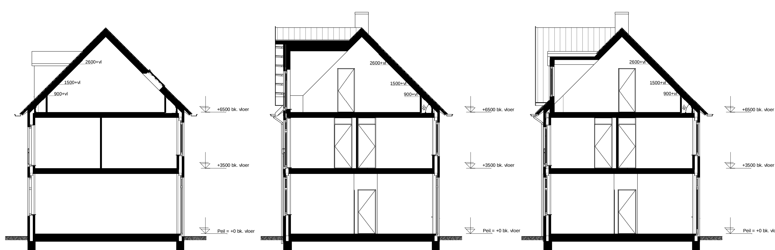
Doorsnede 18-A
