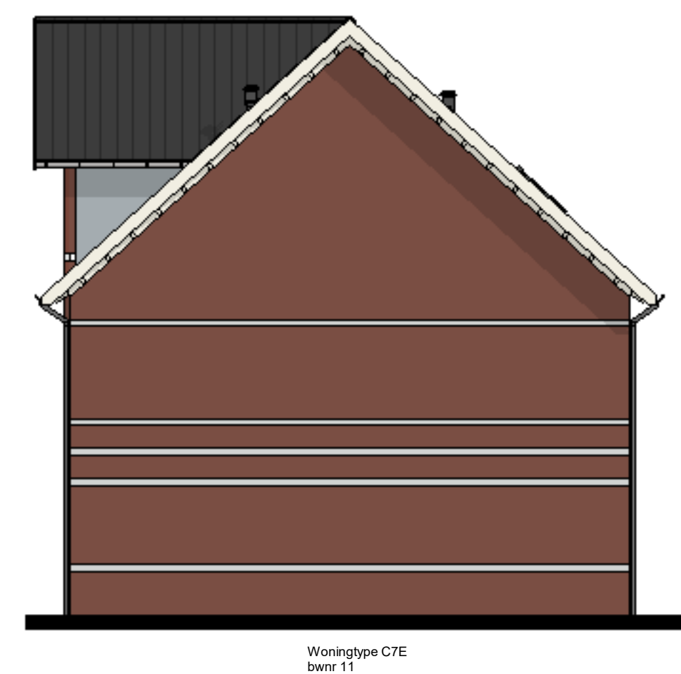
Rechtergevel
