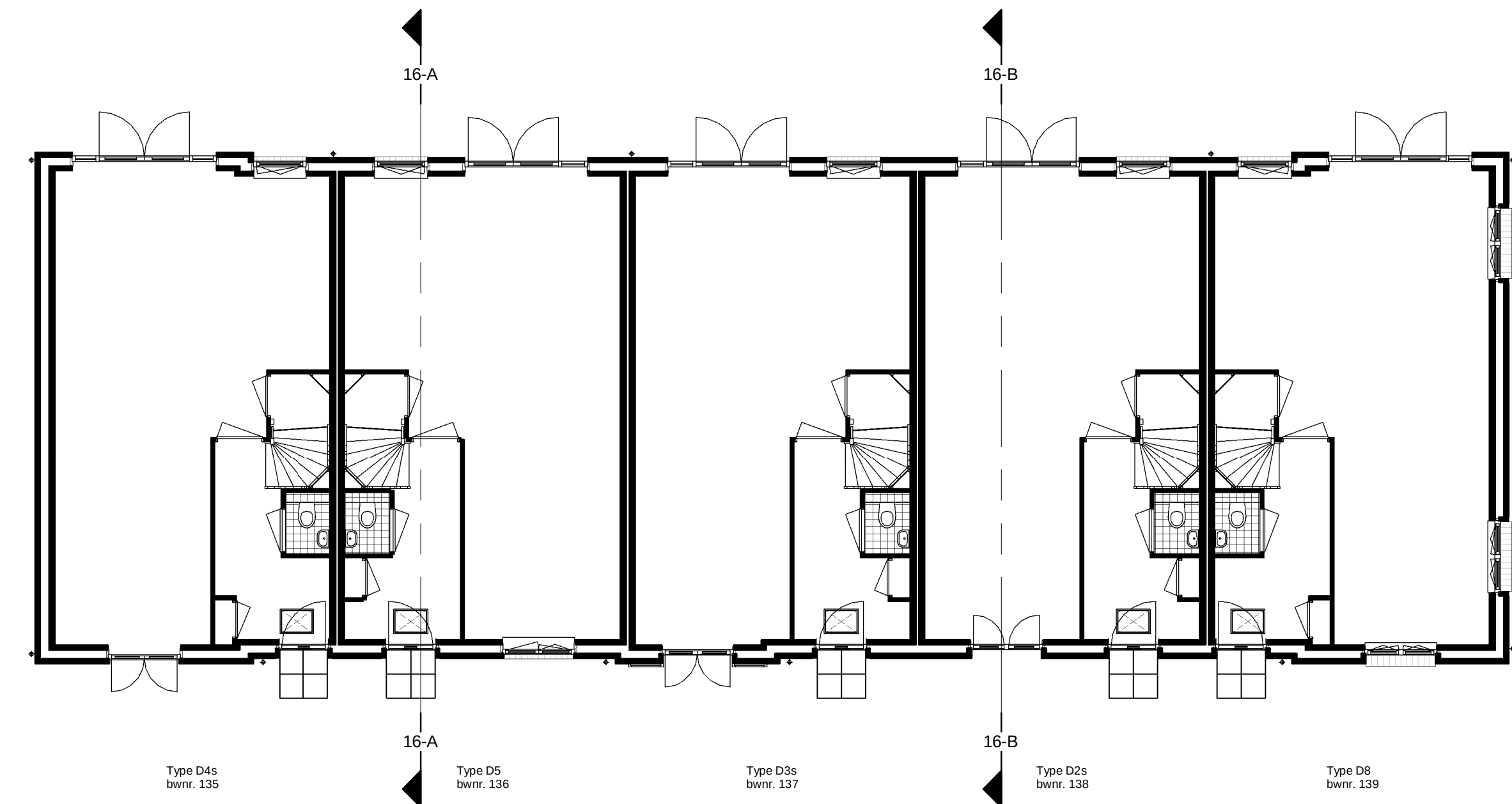
Begane grond
