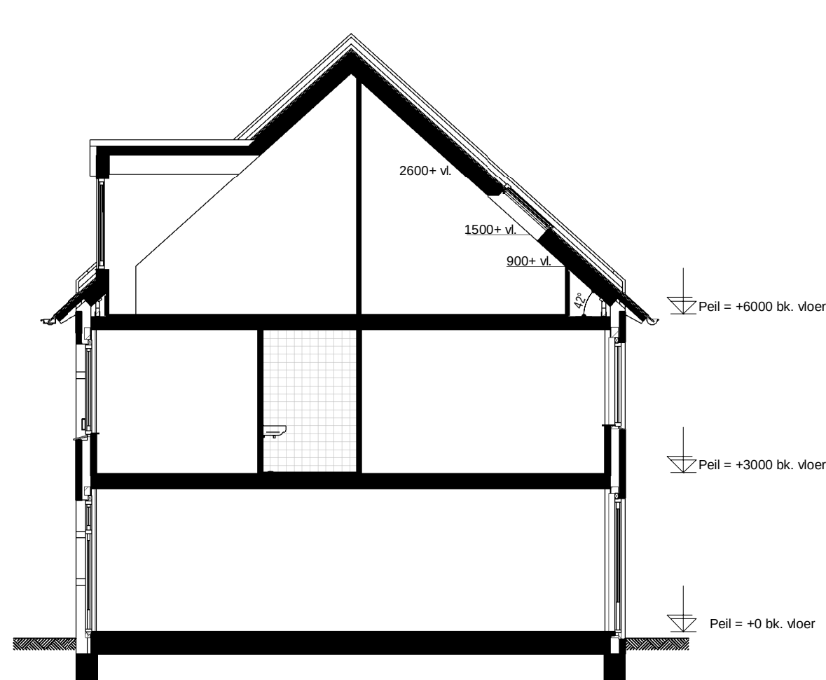
Doorsnede 16-B
