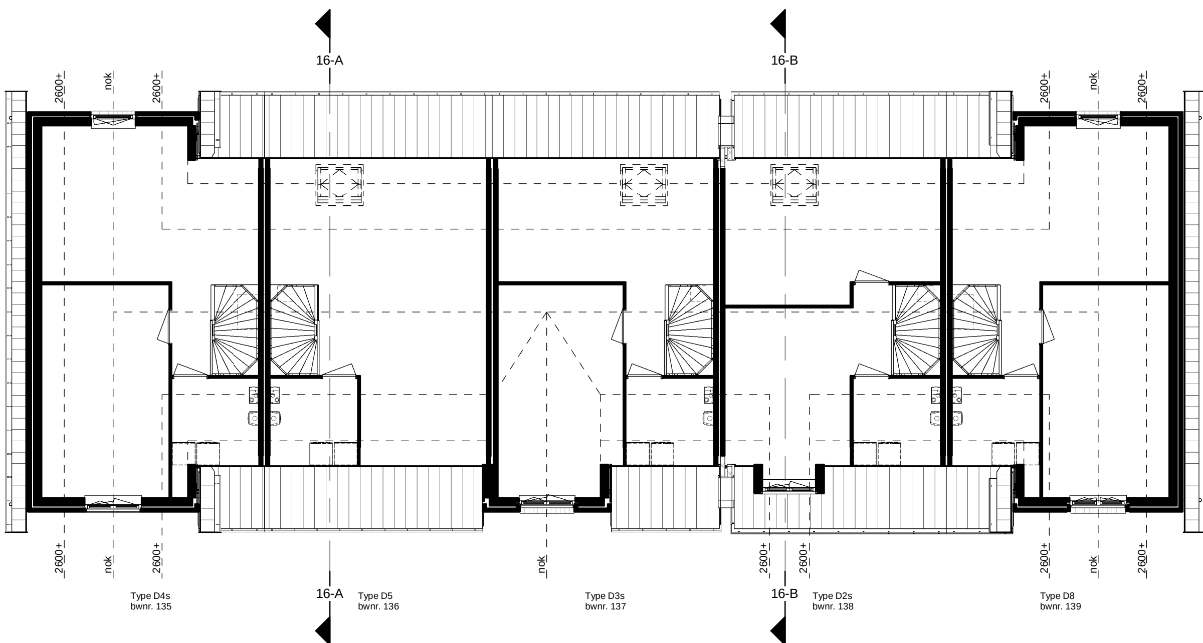
Tweede verdieping
