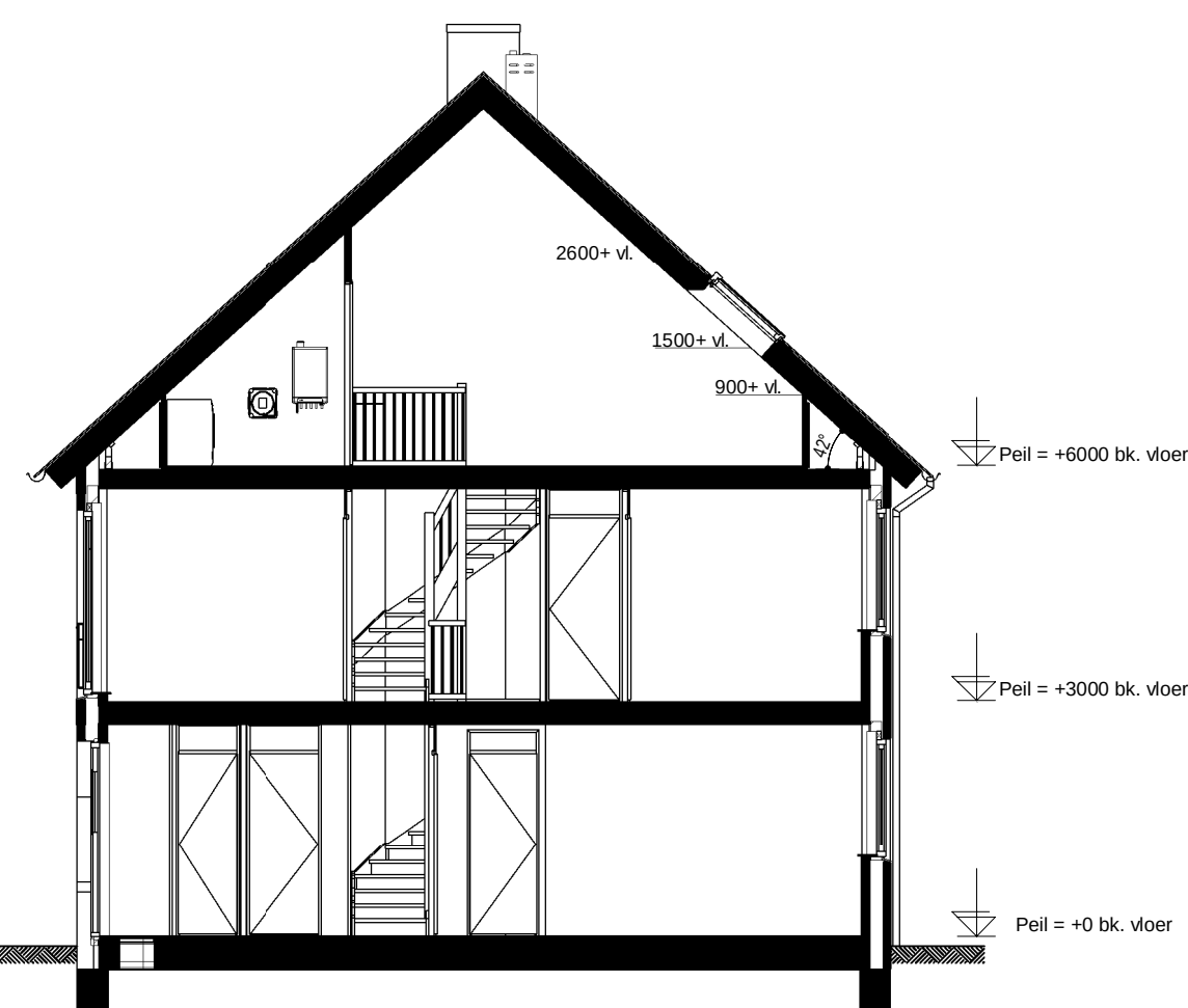
Doorsnede 16-A
