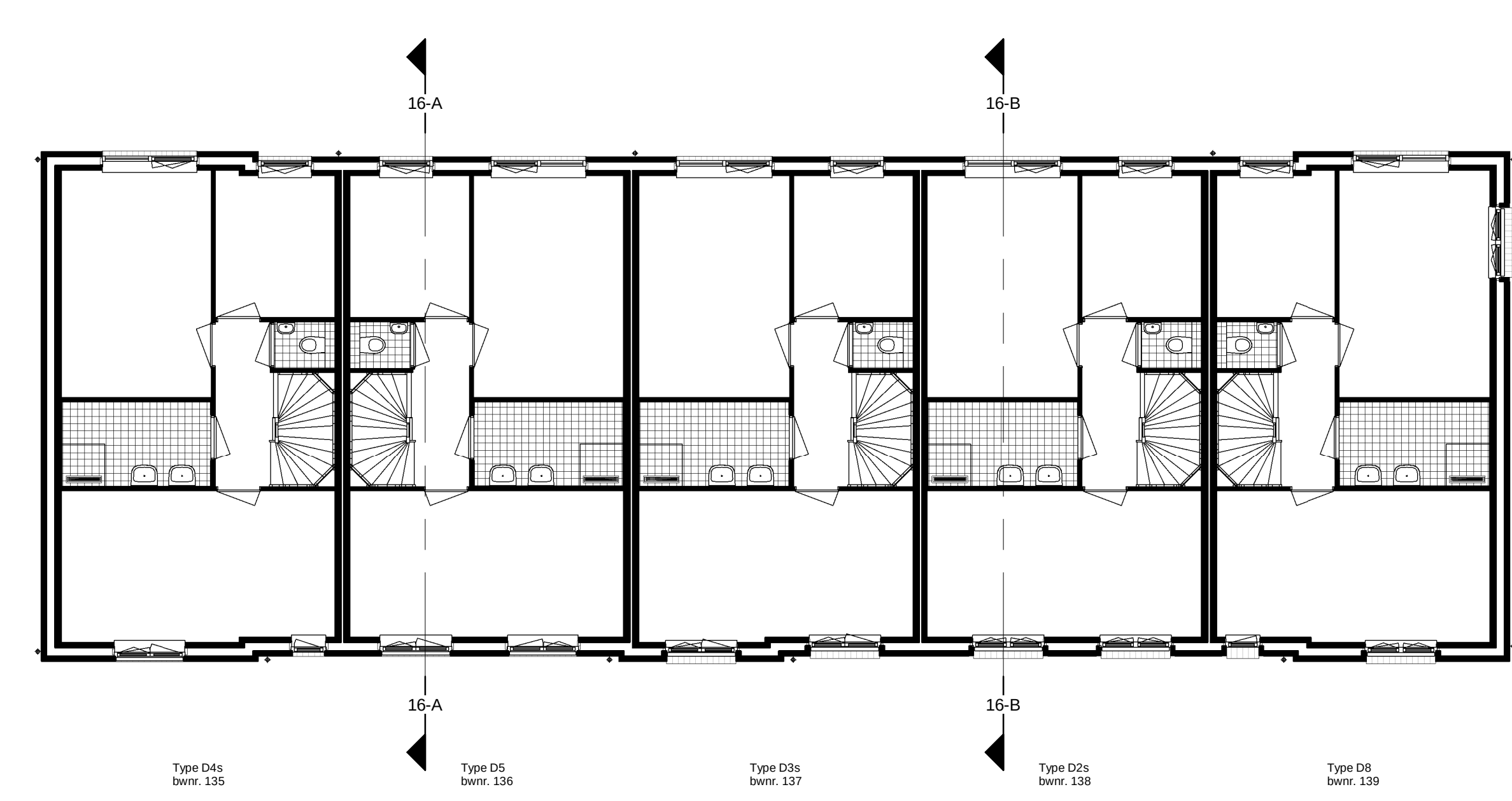
Eerste verdieping
