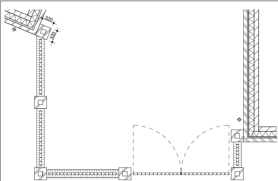
Tuinmuur 12
