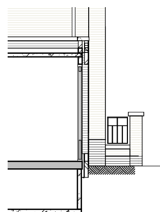
Doorsnede
