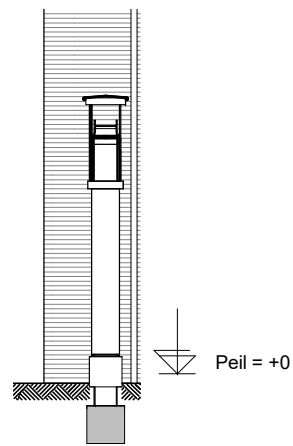
Doorsnede
