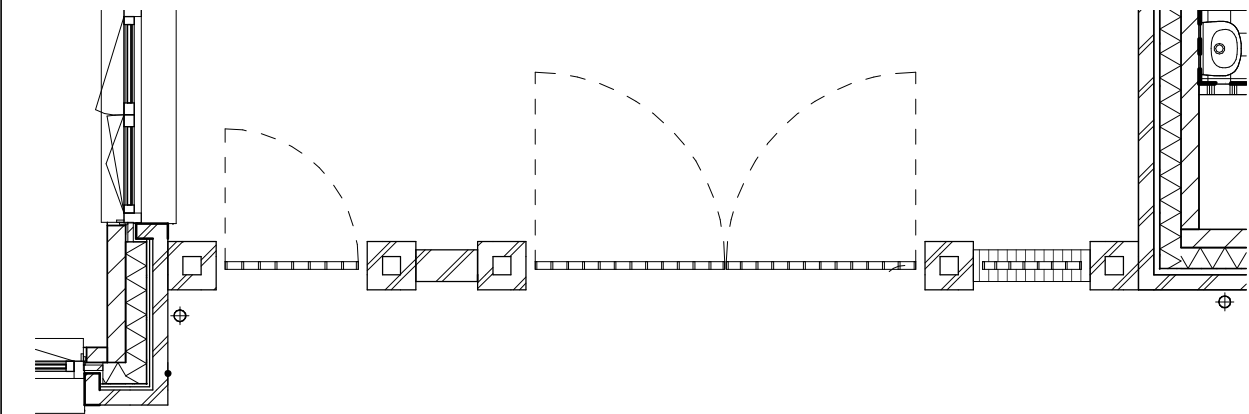
Tuinmuur 13
