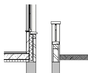
Doorsnede
