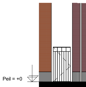
Aanzicht
