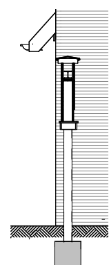
Doorsnede
