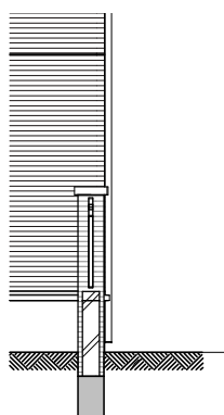
Doorsnede
