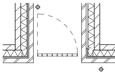
Poort 3
