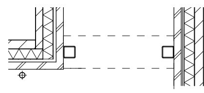
Poort 4
