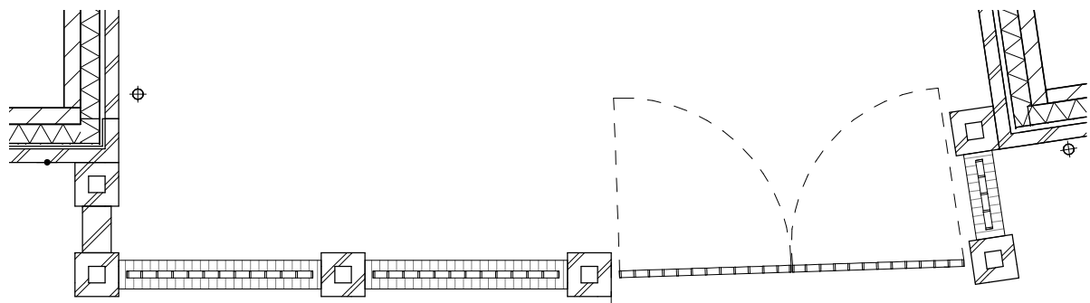
Tuinmuur 4
