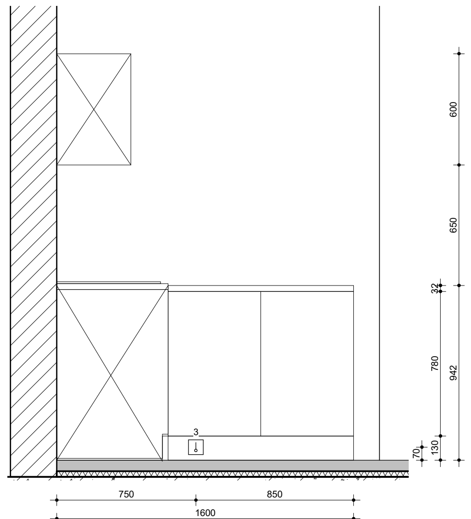
Rechteraanzicht
