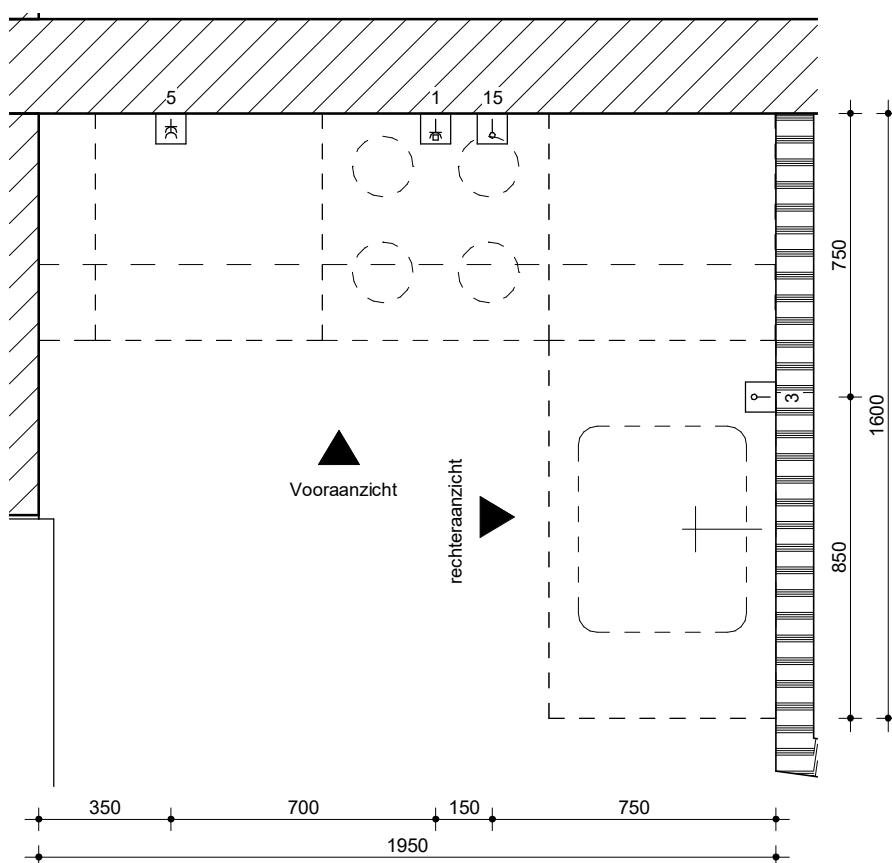
Plattegrond keuken
