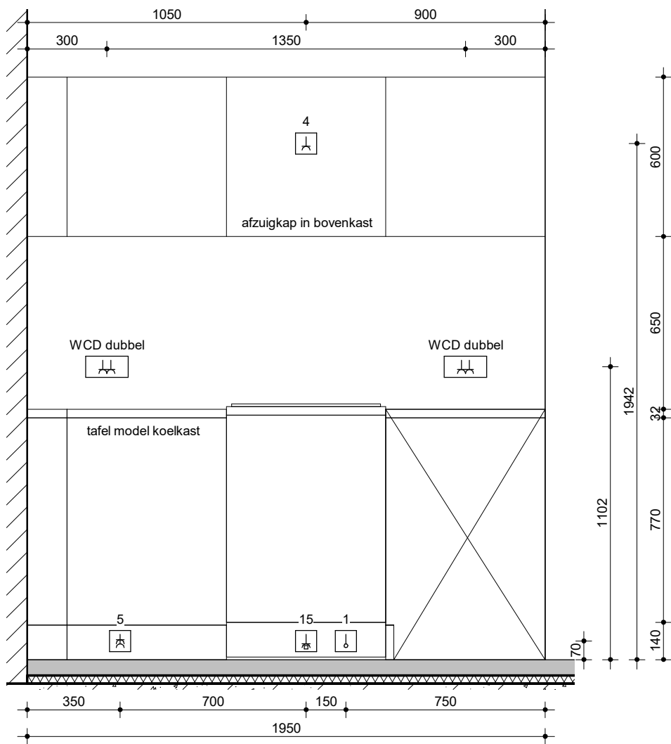
Vooraanzicht
